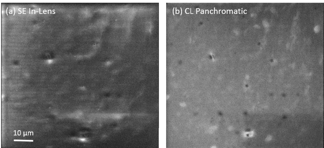
Figura 9. (a) Micrografia FE-SEM della superficie del film di MEH-PPV (zona Z3). (b) Immagine dell'intensità di CL pancromatica della stessa area.
