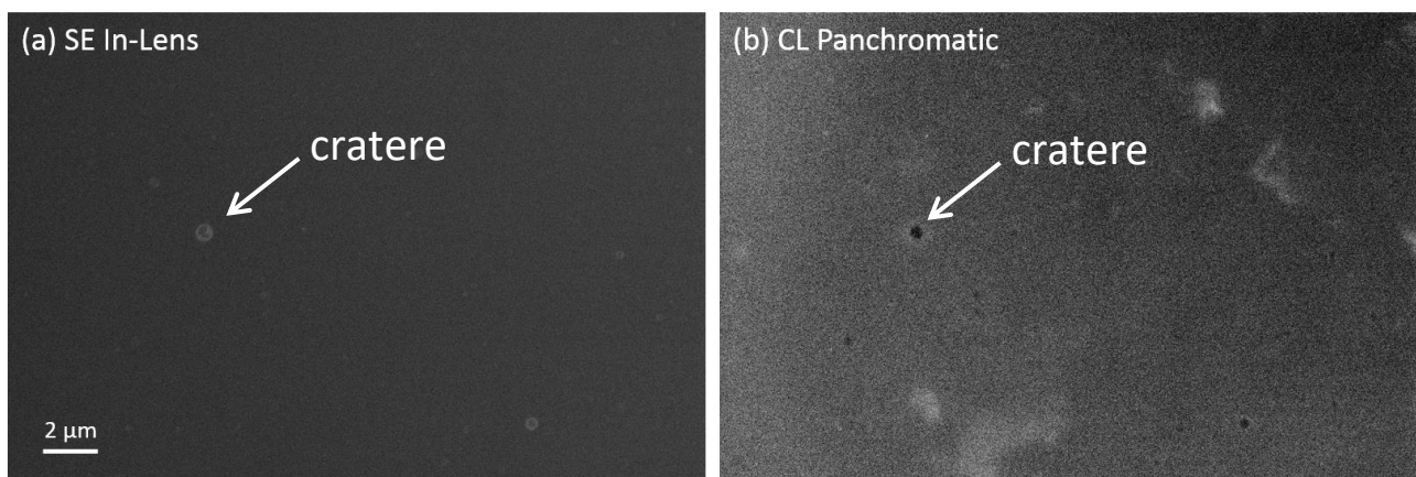
Figura 8. (a) Micrografia FE-SEM della superficie del film di MEH-PPV (zona Z1). (b) Immagine dell'intensità di CL pancromatica della stessa area.
