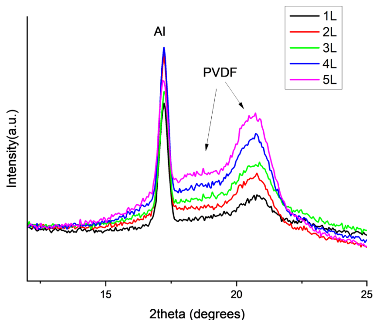
Figura 2. Spettro di diffrazione dei raggi X (Cu K \alpha ) di un film di PVDF multistrato (5 strati) ottenuto depositando mediante rotocalco inchiostri a concentrazione decrescente su un substrato di alluminio.
