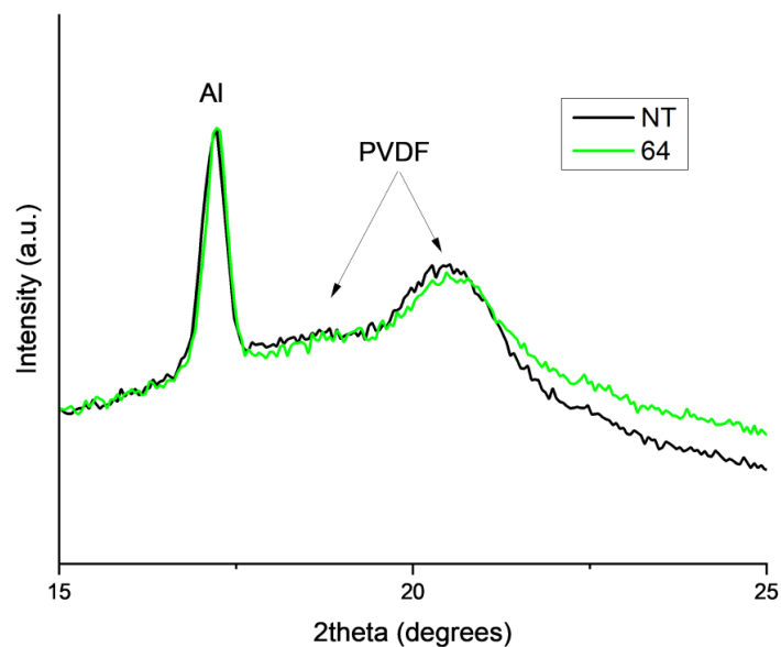
Figura 5. Spettro di diffrazione dei raggi X (Cu K \alpha ) di un film di PVDF multistrato (5 strati) a concentrazione decrescente mediante rotocalco depositato su substrato di alluminio tal quale (NT) e trattato corona alla potenza nominale di 120W per 64 secondi (64).
