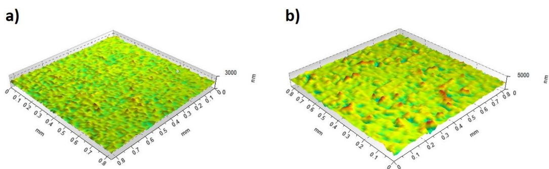
Figura 1. Topografia superficiale: a) superficie del multistrato (5 strati) a concentrazione decrescente di PVDF stampato con rotocalco su ITO-PET; b) superficie dell'elettrodo superiore di rame.
