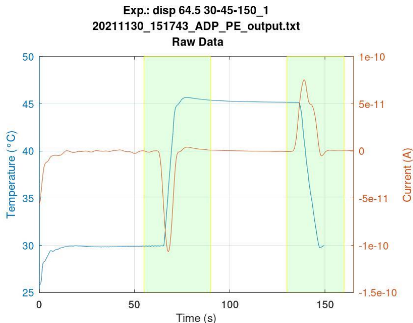
Figura 7: Grafico della temperatura e della corrente elettrica misurate in funzione del tempo per un dispositivo con dielettrico in PVDF multistrato stampato su substrato di ITO-PET trattato corona alla potenza nominale di 120W per 64 secondi.
