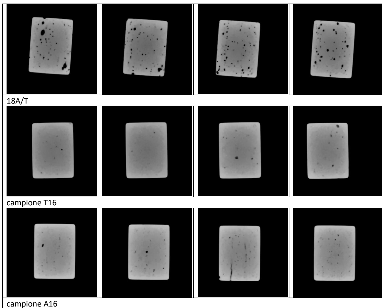
Figura 2: sezioni tomografiche xy
