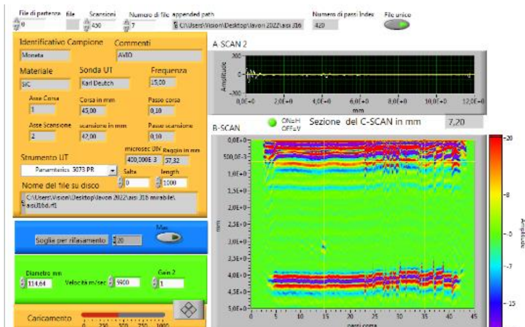
Figura 20. Parametri di misura e di elaborazione. La mappa di sezione o B-scan è focalizzata su un difetto interno a circa 3 mm dalla superficie di ispezione
