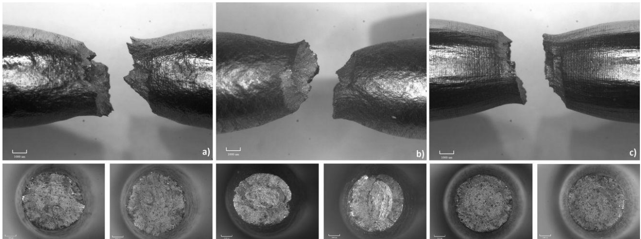
Figura 29: immagini al microscopio ottico, delle zone di frattura dopo le prove meccaniche a 400°C. Campioni con asse ortogonale alla direzione di crescita: NH \perp , a); H \perp , b). Campione con asse parallelo alla direzione di crescita NH \parallel : c) (dimensione del marker 1 mm).
