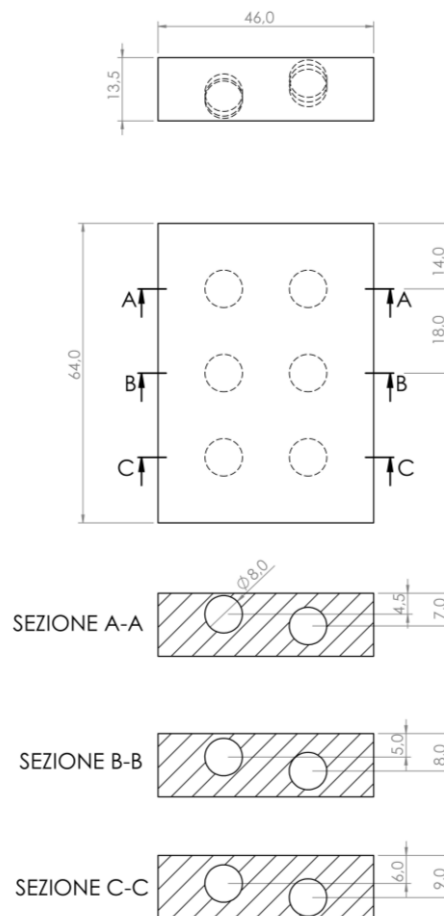
Figura 41. Disegno del campione usato per le prove del sistema prototipale. Le quote sono in mm.
