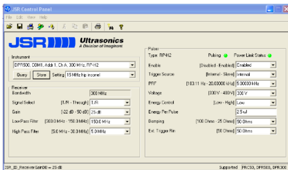
Figura 18: schermata del software di controllo del segnale ultrasonoro
