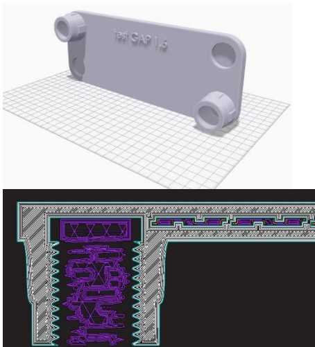
Figura 16: scambiatore di prova posizionato in verticale rispetto al piatto di stampa della Metal X (sinistra); trasparenza con i diversi strati (centro); sezione che mostra il percorso seguito dai due estrusori durante la stampa (destra). I colori sono analoghi a quelli descritti nell'immagine precedente.
