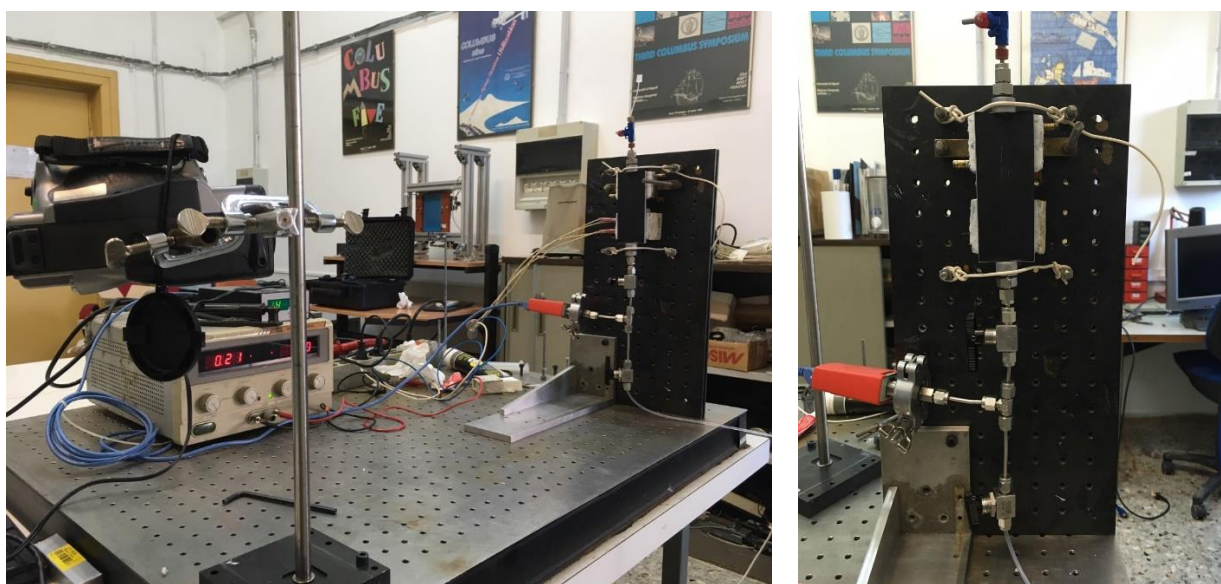
Figura 14 – Impianto sperimentale durante la fase di riempimento.
