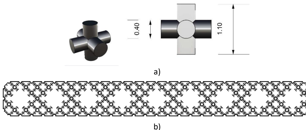
Figura 6 – Cella elementare e quote della cella elementare in millimetri a), struttura capillare del prototipo finale b).
