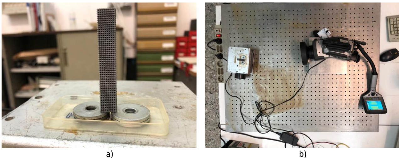
Figura 2 – a) struttura capillare immersa in un disco Petri durante le prove di salita capillare, b) setup sperimentale utilizzato per la misura di salita capillare.
