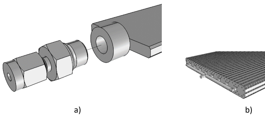
Figura 8 – Particolari del sistema di riempimento utilizzato nel caso di prototipo di heat pipe di tipo flat.
