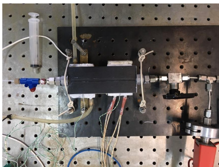
Figura 12 – Setup sperimentale. Il prototipo viene riscaldato e raffreddato alle due estremità utilizzando dei riscaldatori a cartuccia
