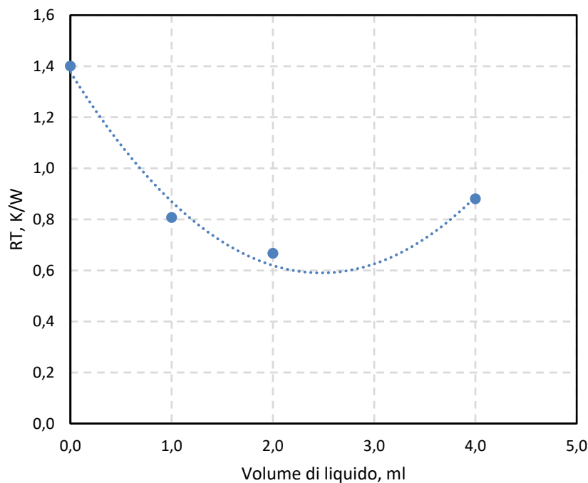
Figura 16 – RT al variare del volume di liquido all'interno della struttura porosa. Potenza all'evaporatore di 15 Watt, temperatura al condensatore fissa a 20°C.
