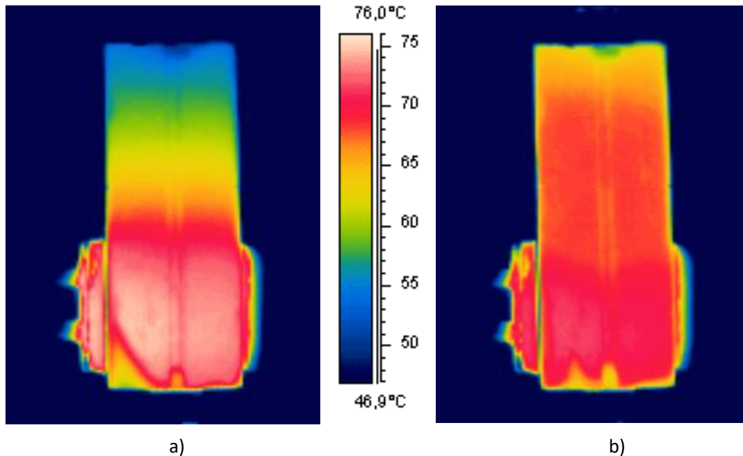
Figura 15 – immagini termografiche prima a) e dopo b) la fase di riempimento.
