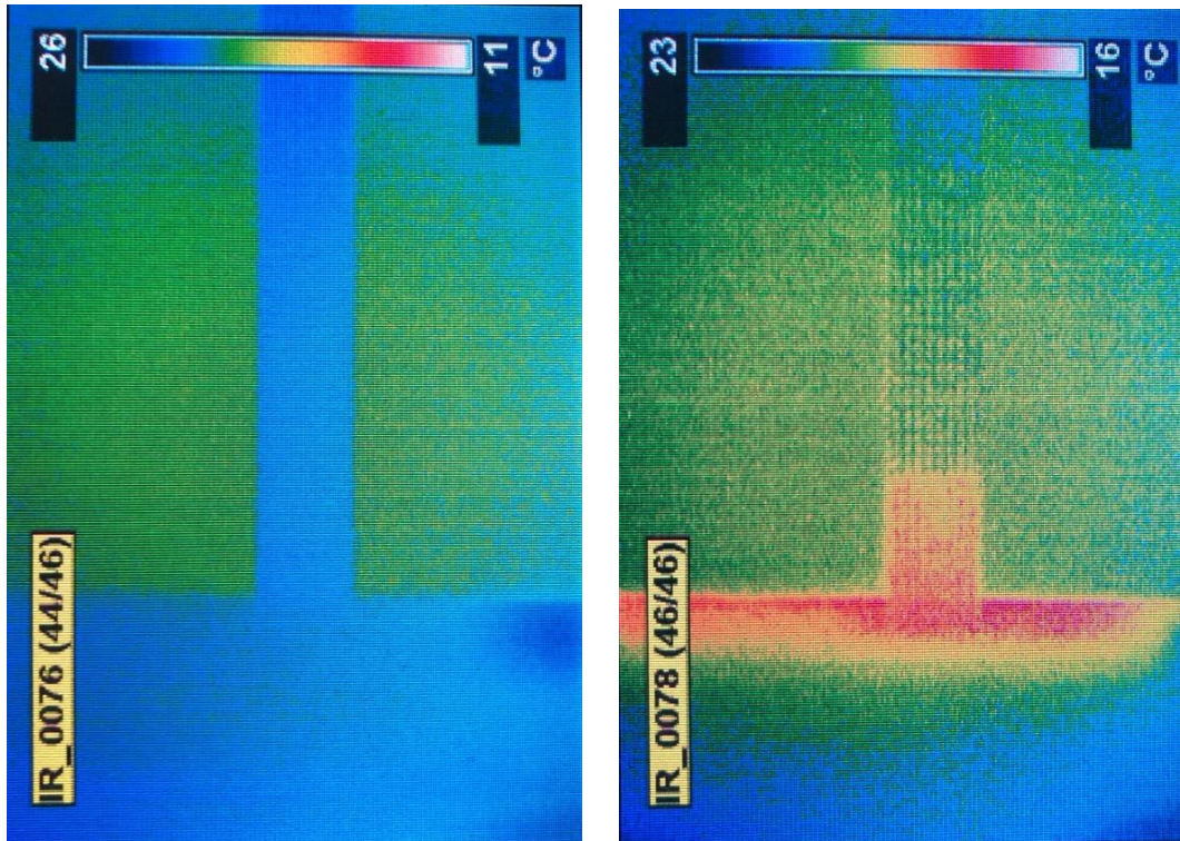
Figura 3 – salita capillare della struttura reticolare bagnata con etanolo. a) immagine termografica in assenza di liquido, b) immagine termografica quando la struttura è bagnata con etanolo.
