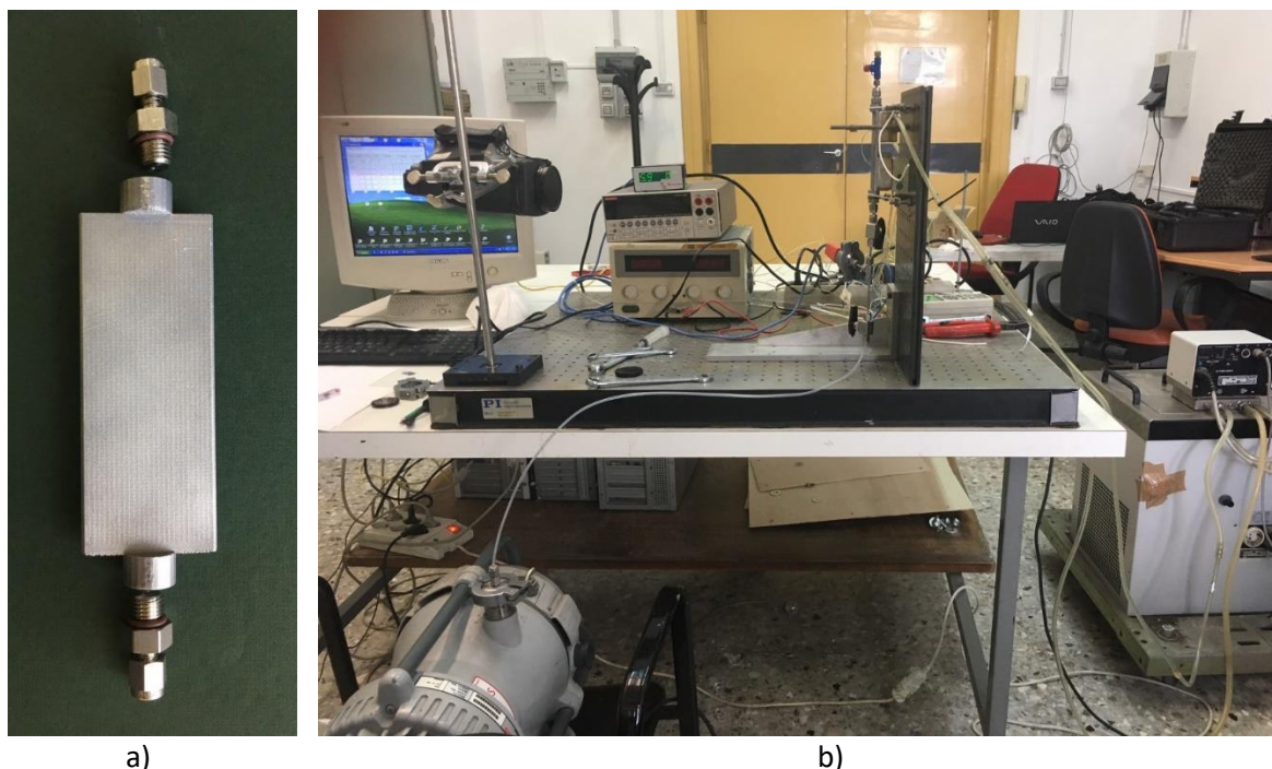
Figura 11 – setup sperimentale allestito per le misure di resistenza e costituito da un alimentatore, un bagno termostatico, un data logger, una pompa da vuoto ed il prototipo.
