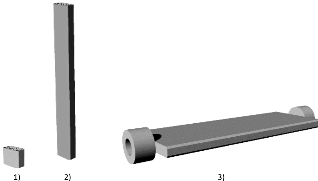
Figura 5 – CAD dei tre prototipi realizzati tramite SLM. 1 2 3
