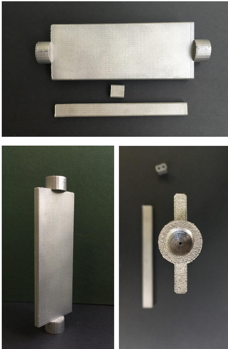
Figura 9 – prototipi realizzati in lega di alluminio AlSi10Mg-0403 tramite SLM.
