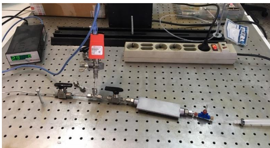
Figura 13 – prototipo di FHP durante la prova di vuoto.
