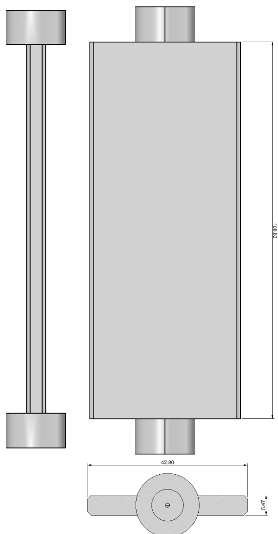
Figura 7 – prototipo di FHP da realizzare tramite tecniche AM.
