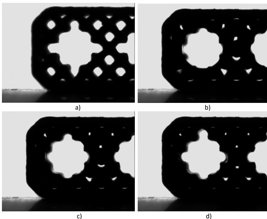
Figura 10 – evaporazione del liquido di lavoro all'interno della struttura capillare. a) prototipo 1 senza liquido di lavoro, b) con liquido di lavoro.
