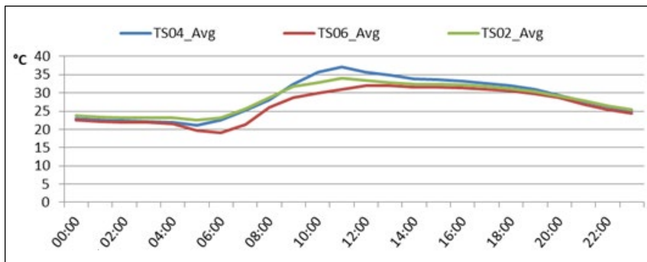
Figura 12. Analisi delle temperature superficiali del 1° luglio 2019. Valori medi (Avg) di temperature superficiali (TS) della parete schermata da Trachospermum jasminoides (TS06), della parete schermata da Partenocissus quinquefolia (TS02) e della parete non schermata (TS04).
