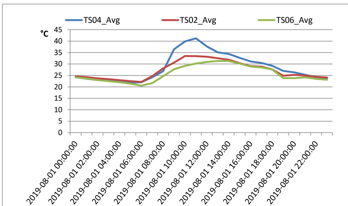
Figura 14. Analisi delle temperature superficiali del 1° agosto 2019. Valori medi (Avg) di temperature superficiali (TS) della parete schermata da Trachospermum jasminoides (TS06), della parete schermata da Partenocissus quinquefolia (TS02) e della parete non schermata (TS04).
