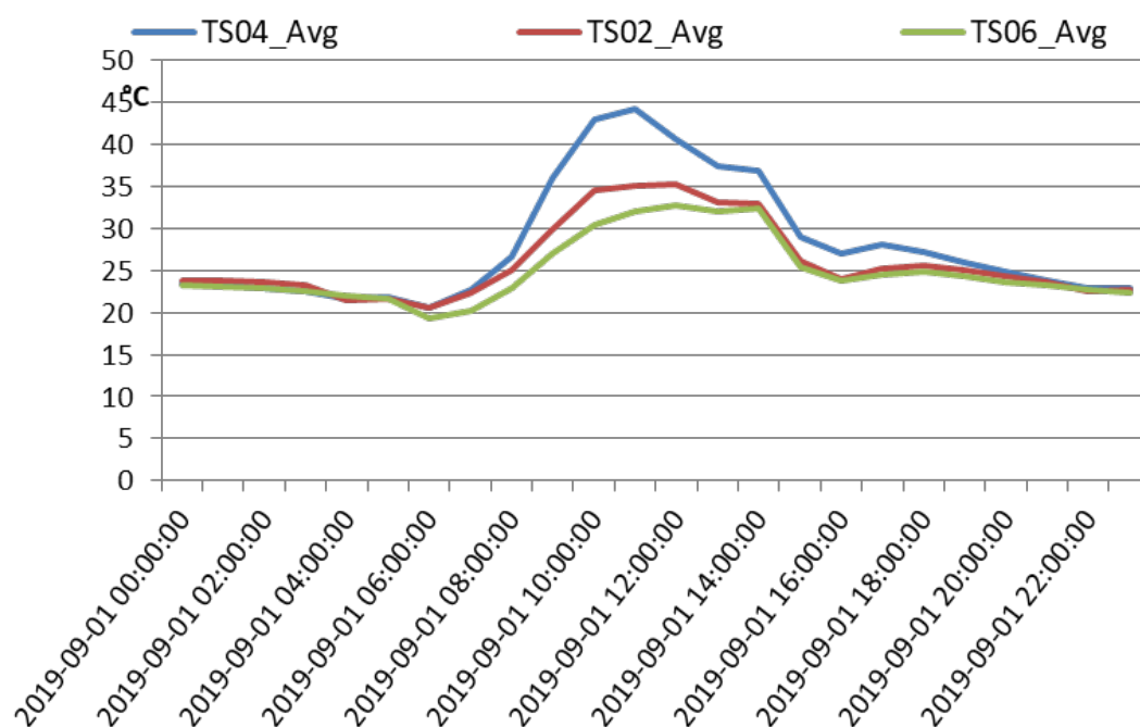
Figura 16. Analisi delle temperature superficiali del 1° settembre 2019. Valori medi (Avg) di temperature superficiali (TS) della parete schermata da Trachlospermum jasminoides (TS06), della parete schermata da Partenocissus quinquefolia (TS02) e della parete non schermata (TS04).
