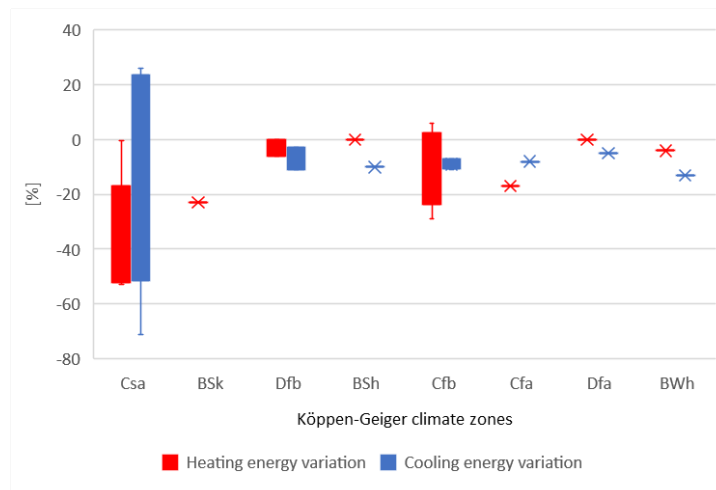
Figura 3. Variazione della domanda di energia per riscaldamento e raffreddamento per tetti verdi installati su solai di copertura isolati termicamente suddivisa per aree climatiche. Fonte: (1)
