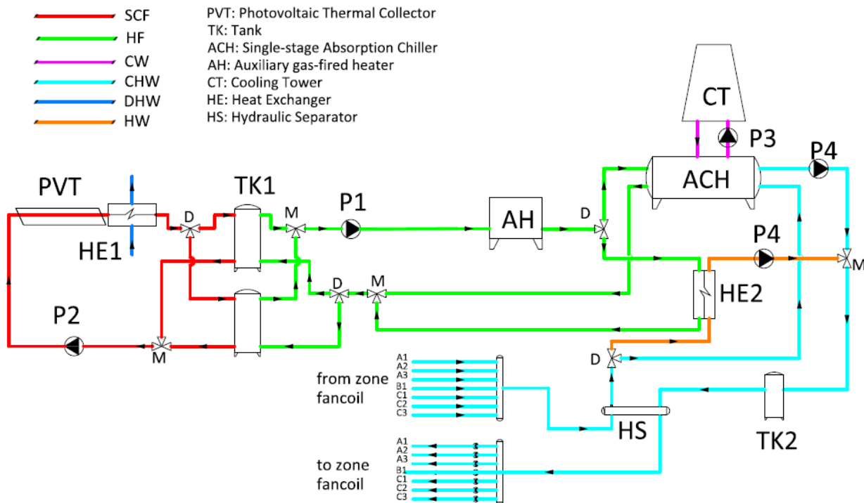
Figura 2. Layout dell'impianto di trigenerazione alimentato da energia solare [8]
