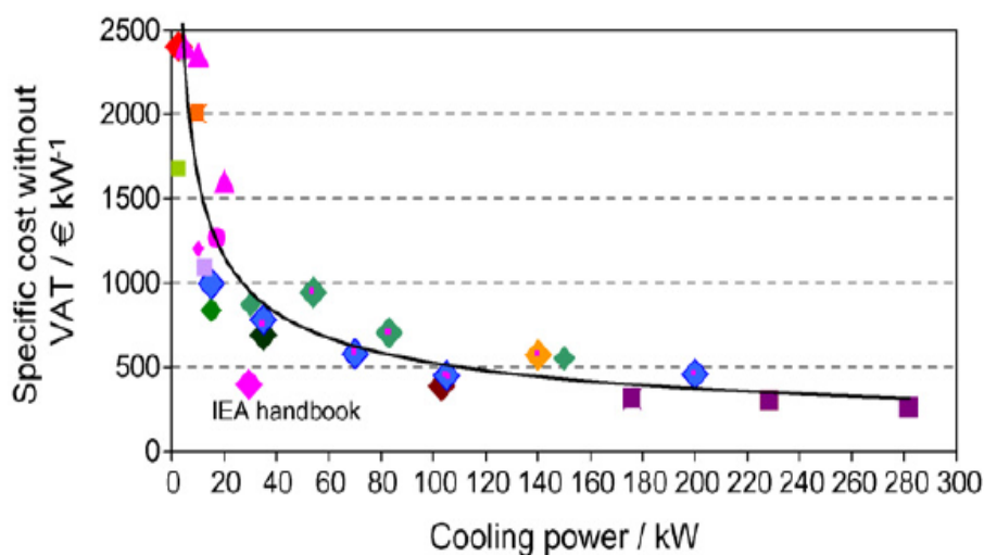
Figura 24. Andamento del costo specifico di una macchina ad assorbimento in funzione della potenza frigorifera secondo Eicker e Pietruschka [41]
