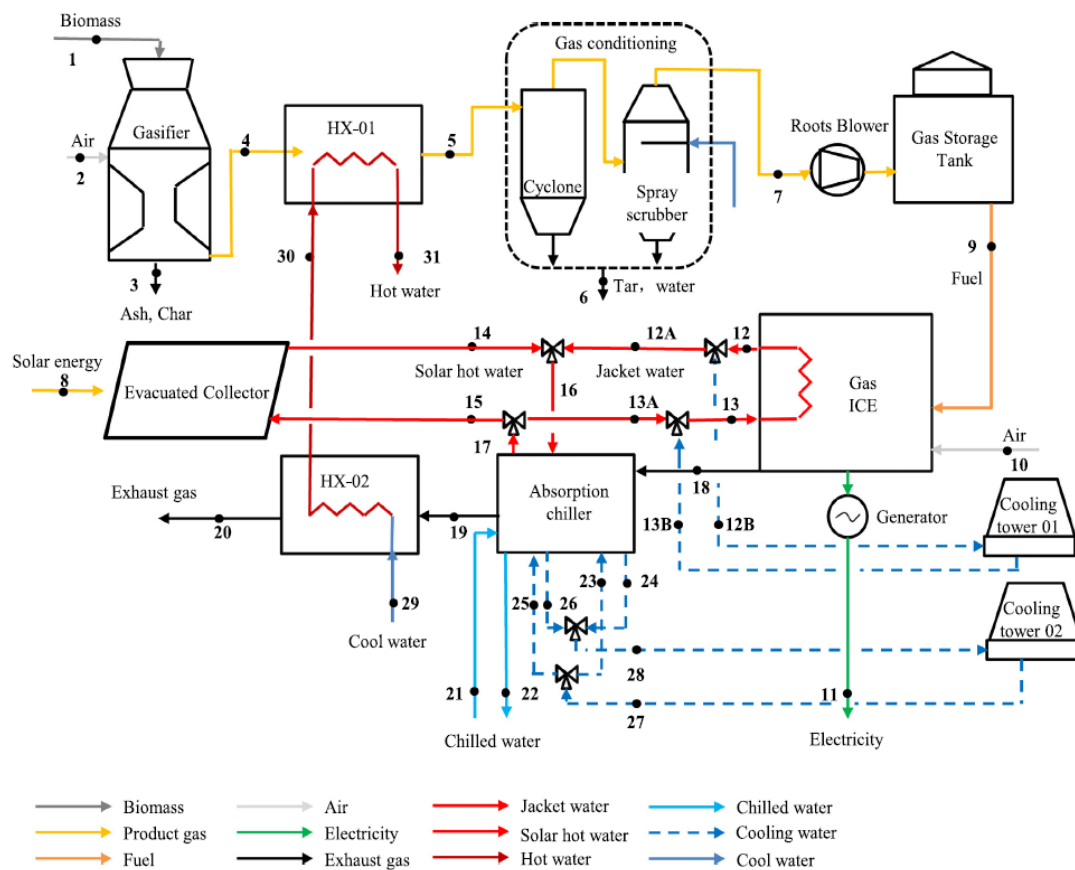
Figura 4. Layout di un impianto di trigenerazione alimentato da energia solare e biomasse [14]
