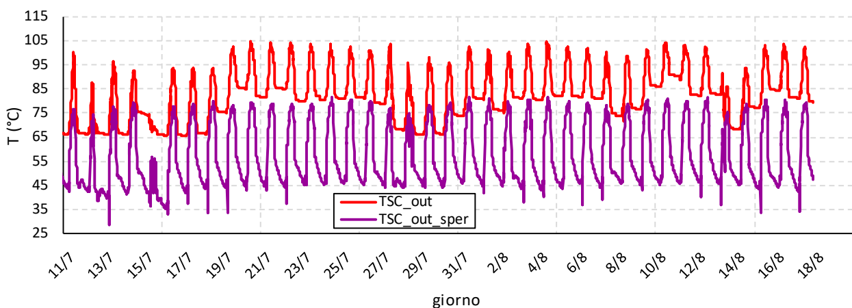
Figura 12. Confronto tra la temperatura all'uscita del campo solare calcolata dal modello di simulazione e quella misurata sperimentalmente
