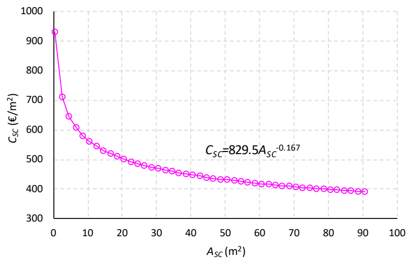
Figura 22. Andamento del costo specifico dei collettori solari a tubi evacuati [41]
