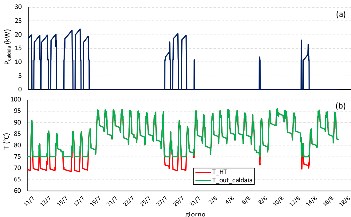
Figura 13. Andamento della potenza termica fornita dalla caldaia a biomassa (a) e della temperatura dell'acqua all'uscita della caldaia e all'interno del serbatoio di accumulo caldo (b)
