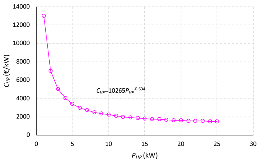
Figura 28. Costo della pompa di calore geotermica in funzione della potenza termica prodotta [53].
