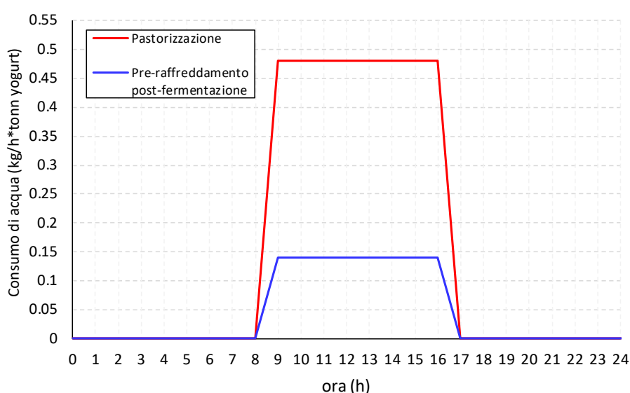
Figura 18. Profili dei consumi di acqua calda e fredda nel processo di produzione dello yogurt
