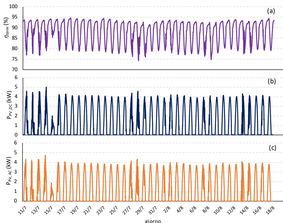
Figura 15. Andamento del rendimento termico (a), della potenza elettrica in corrente continua (b) e della potenza elettrica in corrente alternata (c) nel periodo compreso tra il 11/7/2019 ed il 18/8/2019.
