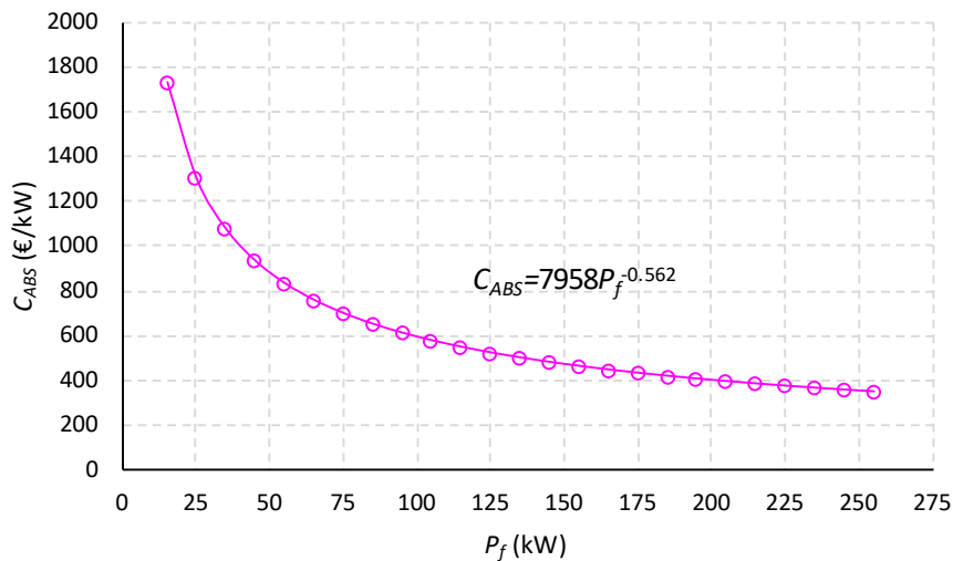
Figura 25. Funzione di costo per macchine ad assorbimento a singolo effetto ottenuta a partire dai dati acquisiti nel progetto SACH - Promotion of solar assisted heating and cooling in the agrofood sector [39]
