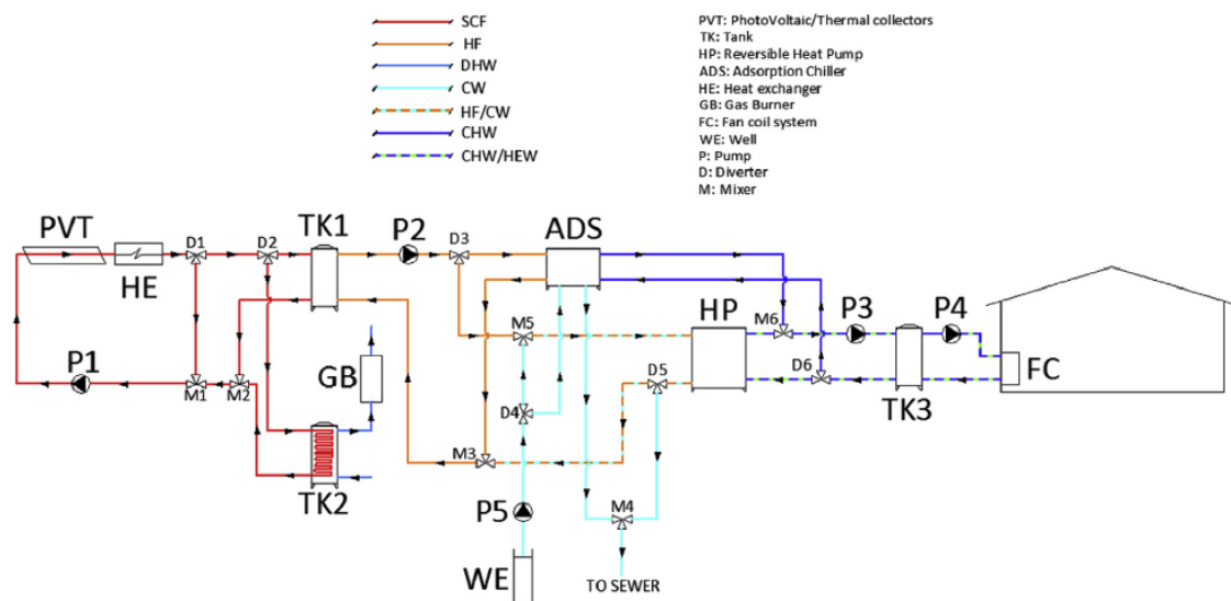
Figura 3. Layout di un impianto di trigenerazione con moduli termo-fotovoltaici, pompa di calore e chiller ad adsorbimento [5]
