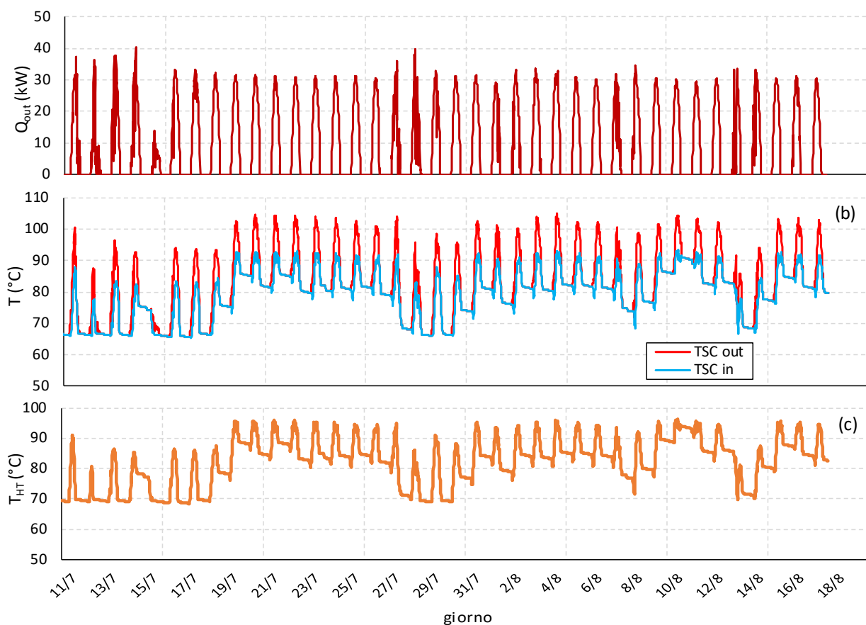
Figura 10. Andamento della potenza termica prodotta, delle temperature all'ingresso e all'uscita del campo solare e della temperatura media del serbatoio di stoccaggio nel periodo compreso tra l'11/07/2019 e l'18/08/2019
