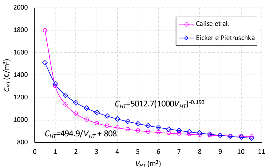
Figura 23. Andamento del costo specifico di un serbatoio di accumulo senza scambiatore secondo Eicker e Pietruschka [41] e Calise et al. [46].
