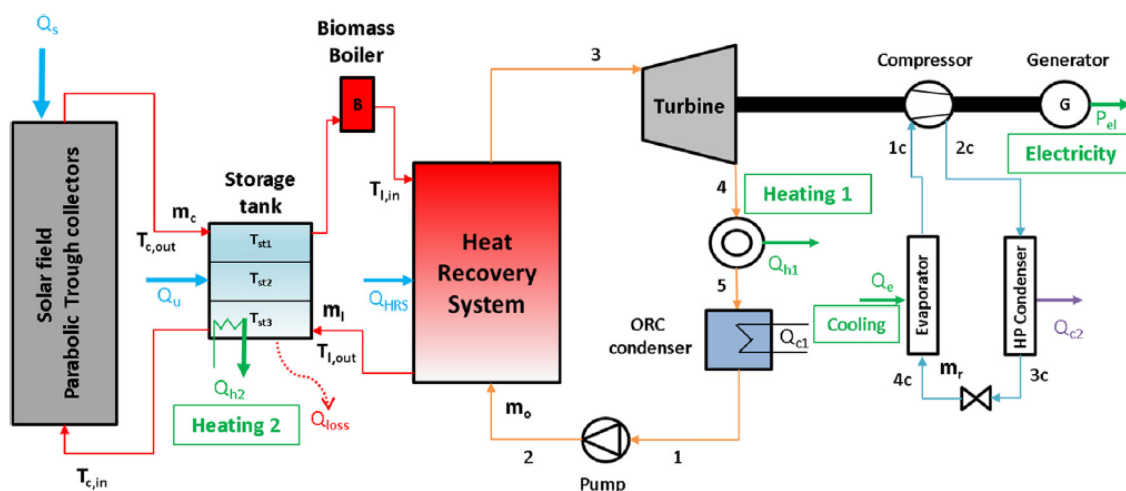
Figura 5. Sistema di trigenerazione integrante collettori solari parabolici, ORC, caldaia ausiliaria a biomasse, serbatoio di accumulo caldo e VCC [18]
