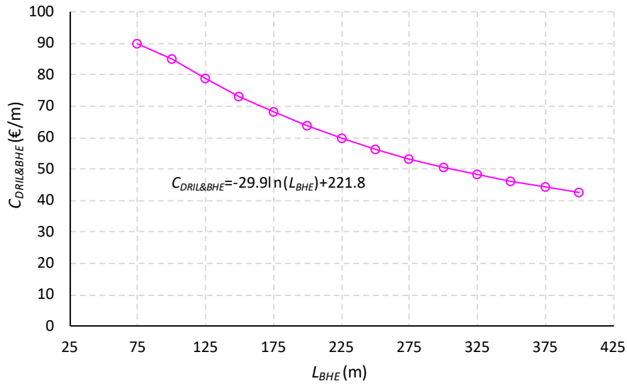
Figura 29. Costo dello scavo e della sonda geotermica in funzione della profondità [53].
