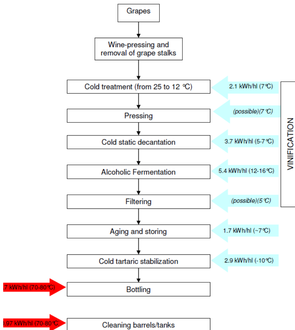
Figura 21. Schema di processo di produzione del vino bianco ed indicazione dei consumi energetici delle diverse fasi di processo [39]
