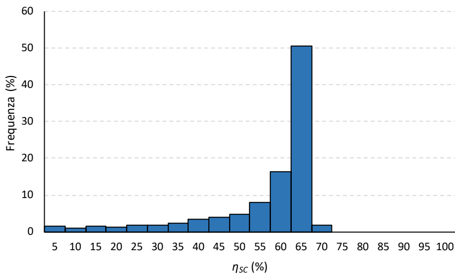
Figura 11. Funzione di distribuzione del rendimento dei collettori solari nel periodo compreso tra l'11/07/2019 e l'18/08/2019
