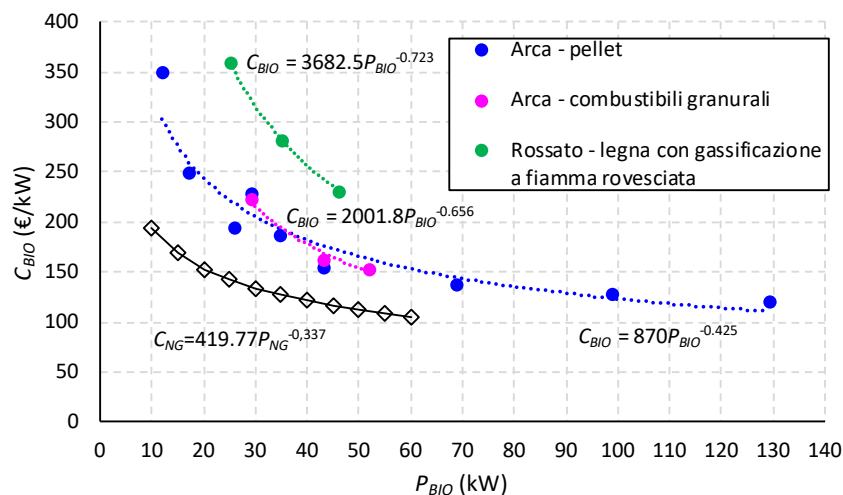
Figura 27. Funzioni di costo per differenti tipologie di caldaia a biomassa, desunte dai dati provenienti dalle case costruttrici Arca [51] e Rossato [52] e confronto con il caso di una caldaia ausiliaria a gas naturale [39].
