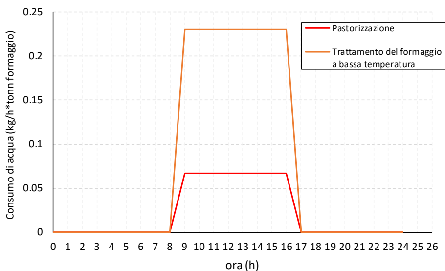
Figura 19. Profili dei consumi di acqua calda nel processo di produzione di formaggio a pasta molle
