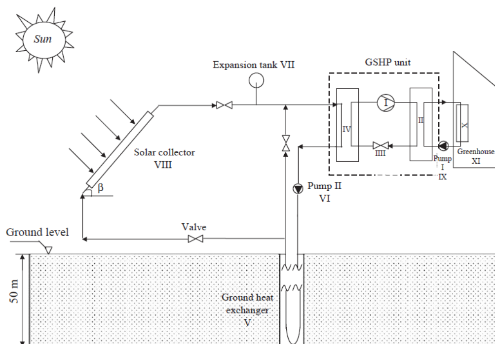
Figura 8. Impianto sperimentale di condizionamento di una serra alimentato da energia solare e geotermica [29]
