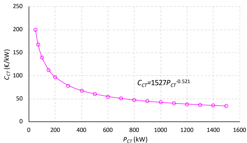
Figura 26. Funzione di costo per una torre evaporativa ottenuta a partire dai dati acquisiti nel progetto SACH - Promotion of solar assisted heating and cooling in the agrofood sector [39]
