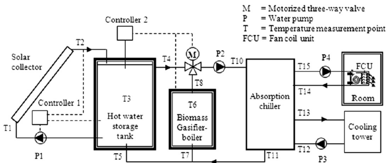
Figura 7. Impianto sperimentale di condizionamento dell'aria alimentato ad energia solare e biomasse [28]
