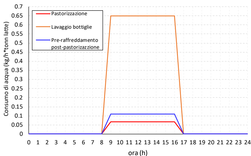
Figura 17. Profili dei consumi di acqua calda e fredda nel processo di produzione del latte
