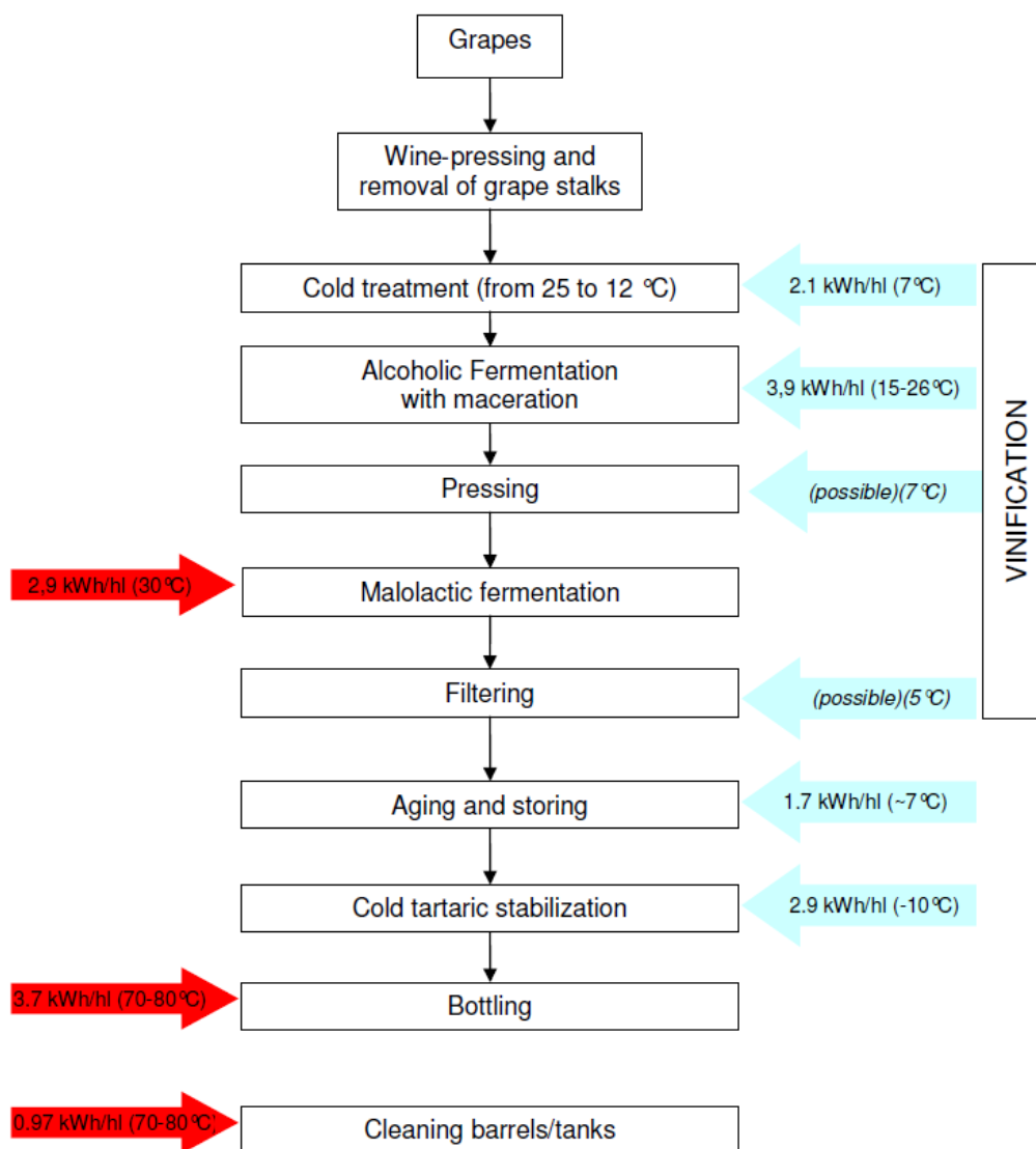
Figura 20. Schema di processo di produzione del vino rosso ed indicazione dei consumi energetici delle diverse fasi di processo [39]
