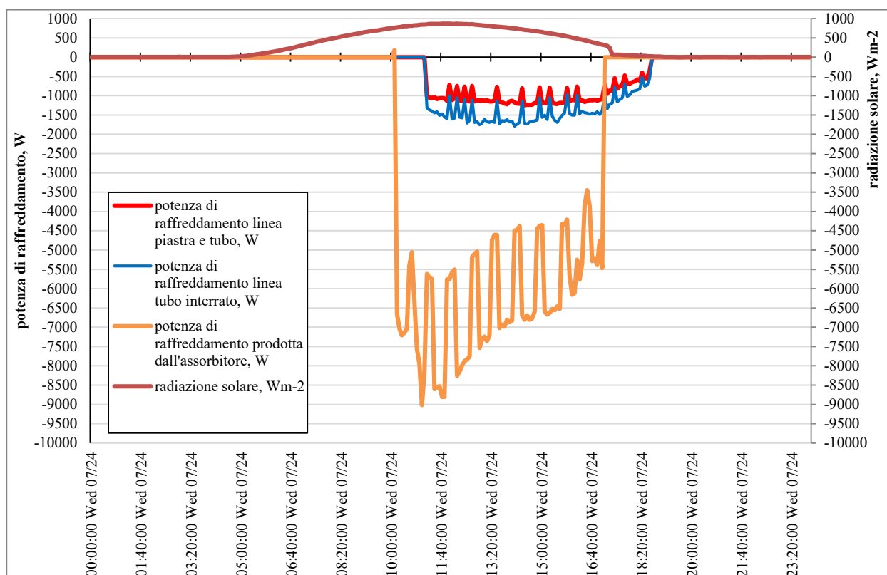
Figura 16. Potenza di raffreddamento fornita dall'assorbitore ed erogata sulla linea di coltivazione con piastra e tubo e con tubo interrato; radiazione solare; 24/07/2019.
