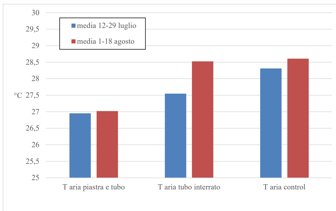
Figura 20. Media delle temperature dell'aria misurate nelle zone di coltivazione in presenza di raffreddamento con piastra e tubo, con tubi interrati e in assenza di raffreddamento (controllo); medie dei periodi 12-29/07/2019 e 1-18/08/2019.
