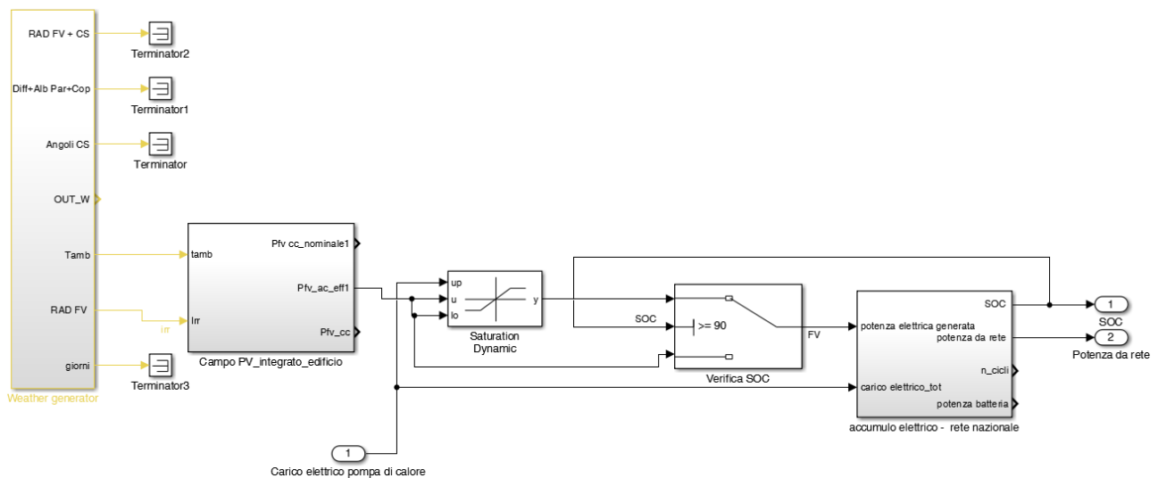
Figura 2.33. Integrazione modello impianto FV – accumulo elettrico con sistema di gestione flussi di potenza – connessioni in isola tipo B
