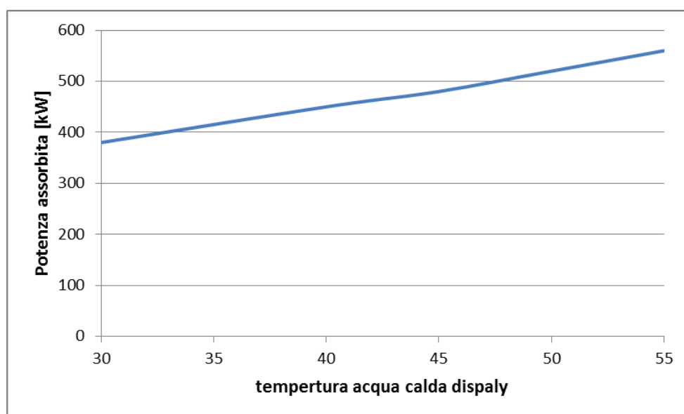
Figura 2.23. Assorbimento elettrico della pompa di calore vs temperatura acqua accumulo – da misure sperimentali
