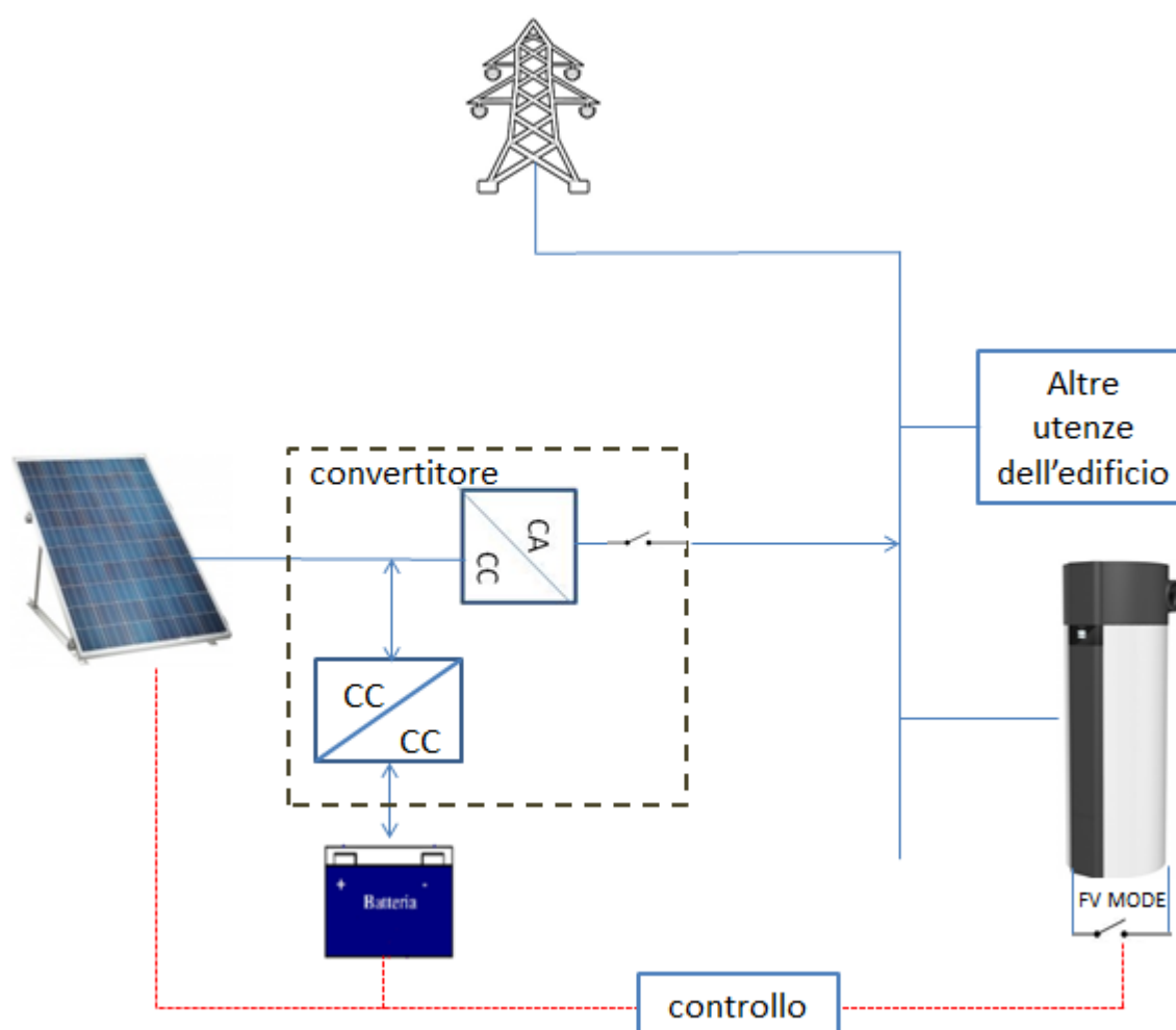
Figura 2.34. Schema connessione impianto PV-pompa di calore con accumulo – modalità grid connected
