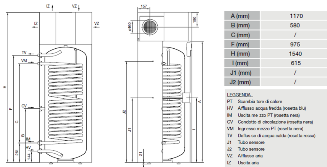
Figura 2.22. Schema e principali dimensioni della Pompa di calore oggetto di studio
