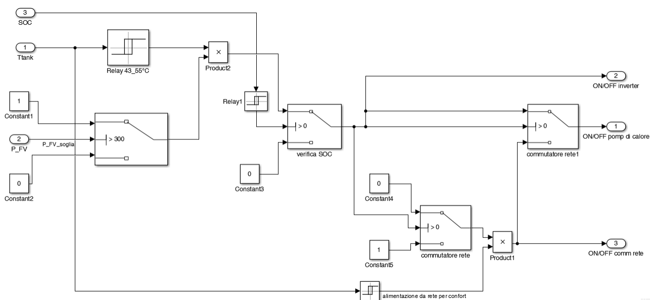
Figura 2.28. Dettaglio modello “termostato inseguimento FV” per gestire l’alimentazione della pompa di calore da inverter FV o da rete
