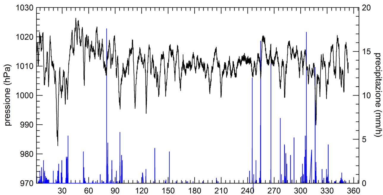
Figura 5.1. Evoluzione dei valori medi orari di pressione atmosferica (curva nera) e precipitazione (curva blu) misurati all'Osservatorio Climatico di Lampedusa durante il 2019
