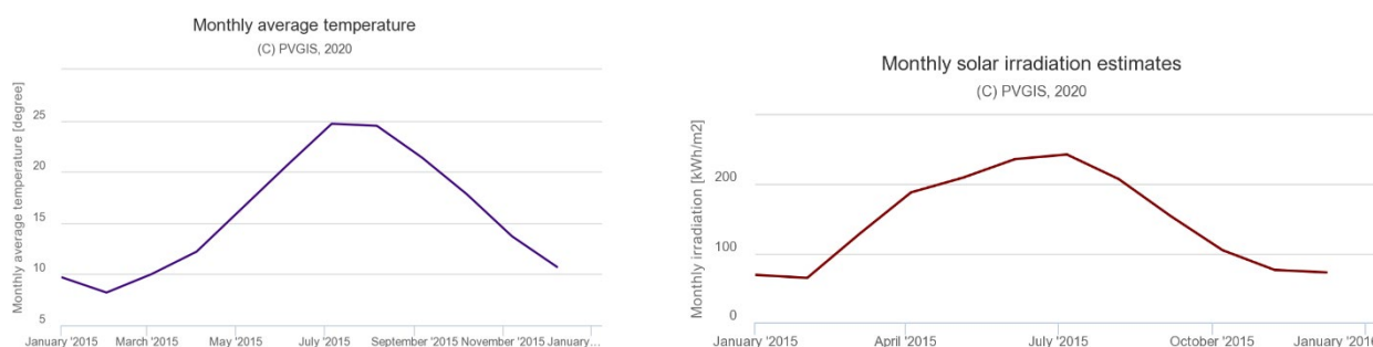
Figura 3.16. Andamento medio mensile della temperatura e della radiazione sul piano orizzontale, Isola di Marettimo, anno 2015. Fonte: PVGIS-SARAH
