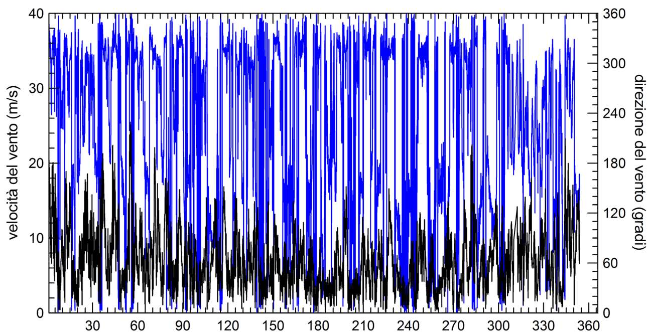
Figura 5.3. Evoluzione dei valori medi orari di velocità (curva nera) e direzione (curva blu) del vento misurati all'Osservatorio Climatico di Lampedusa durante il 2019
