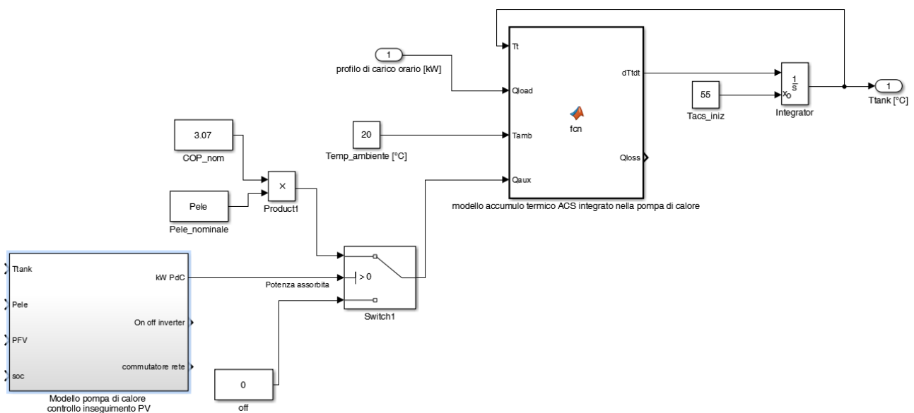
Figura 2.25. Modello pompa di calore e accumulo termico integrato – dettaglio blocchi per calcolo potenza termica Quax fornita all'accumulo integrato
