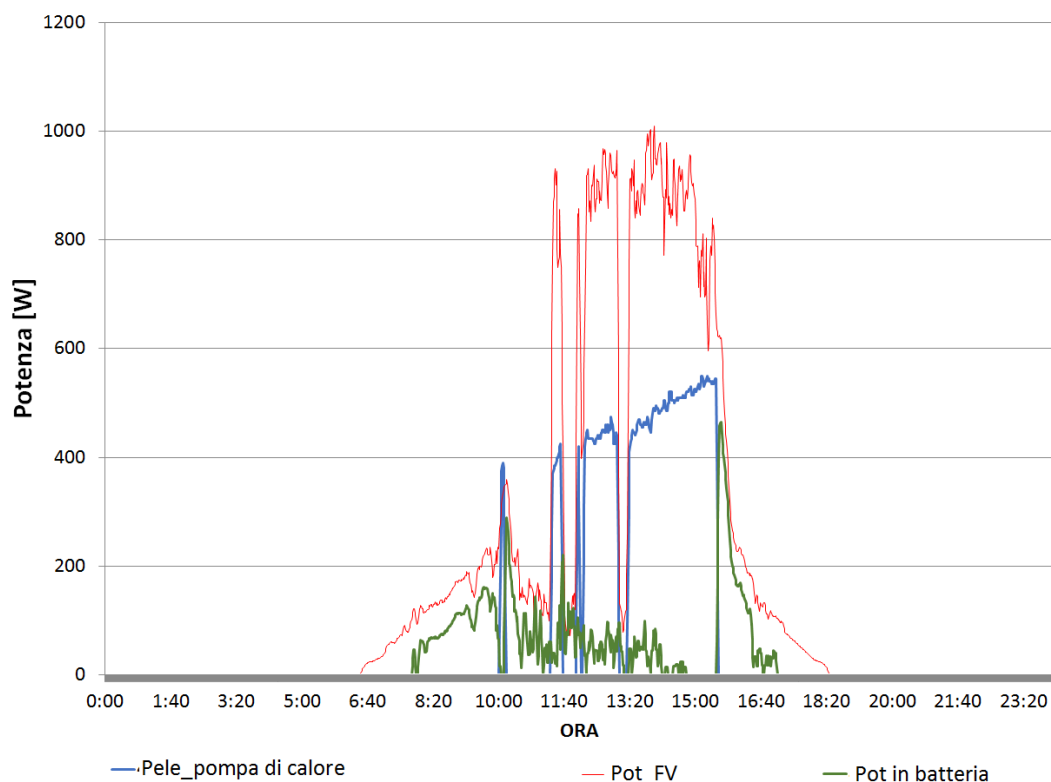
Figura 2.13. Prova sperimentale – misura grandezze elettriche giorno 2
