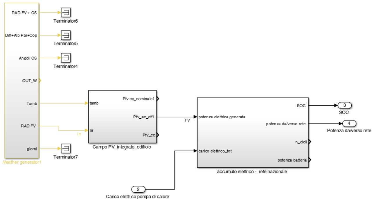
Figura 2.36. Integrazione modello impianto FV – accumulo elettrico con sistema di gestione flussi di potenza scambiati con la rete -- connesine grid connected
