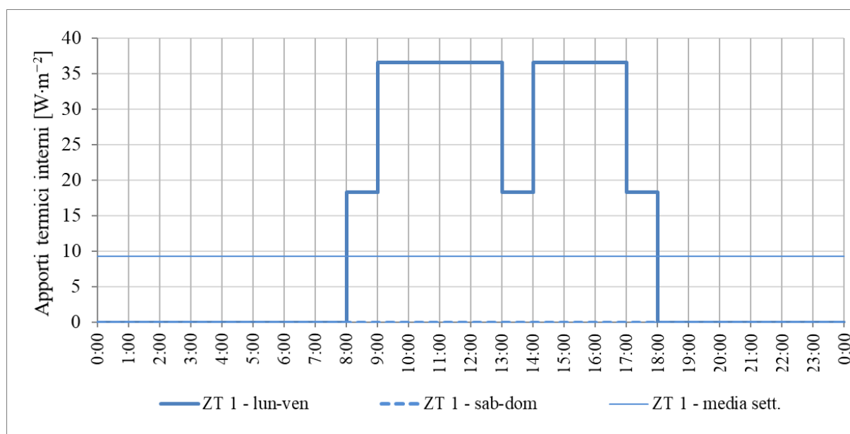
Figura 40. Profilo orario degli apporti interni di calore (quota sensibile) dovuti a occupanti, apparecchiature e illuminazione. Esempio per la zona termica 1.
