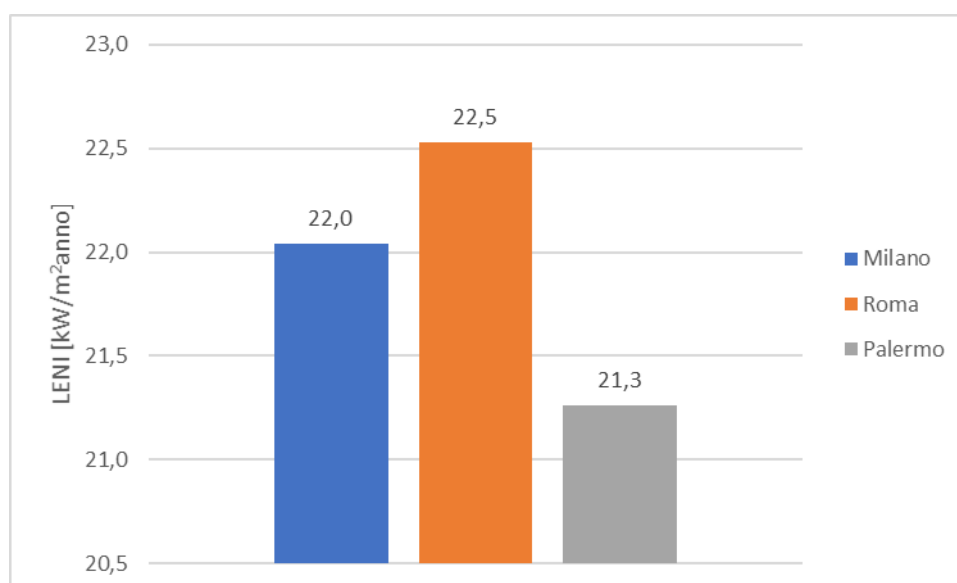
Figura 82. Calcolo del LENI per le località considerate
