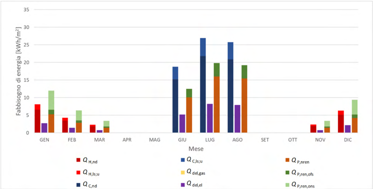
Figura 70. Fabbisogno di energia primaria per riscaldamento e raffrescamento - Roma (regime intermittente) Soluzione 2
