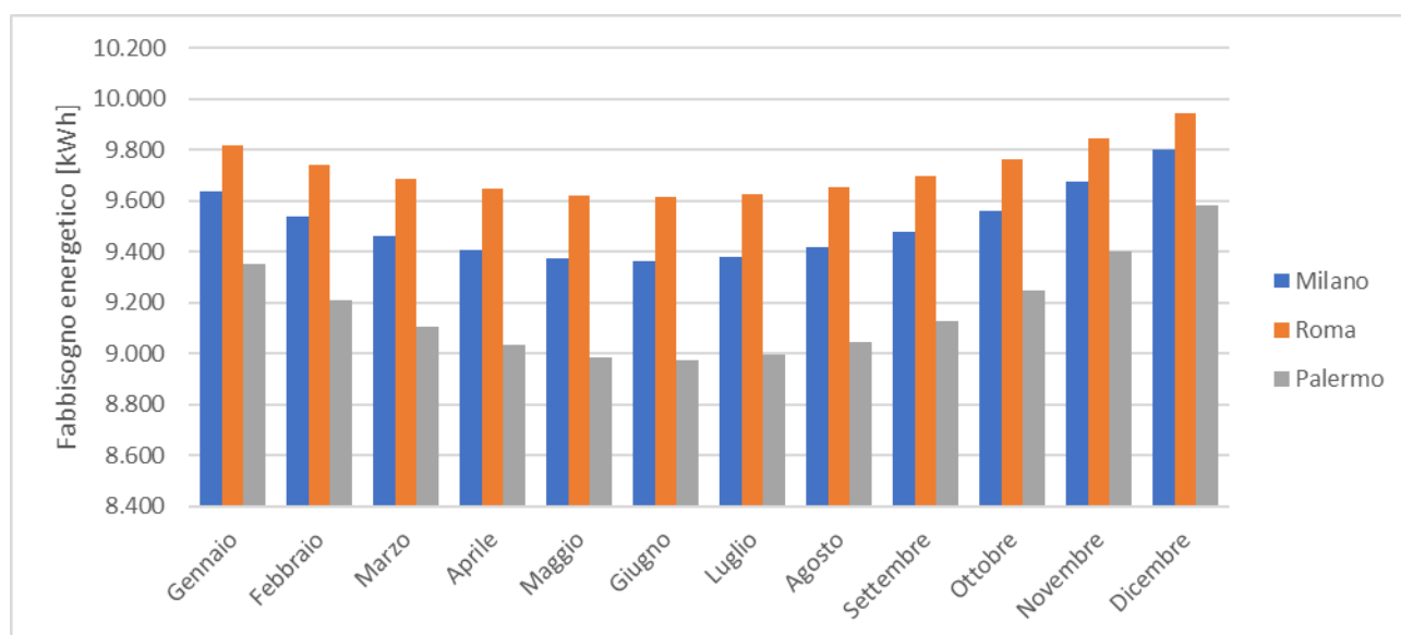
Figura 81. Fabbisogno energetico annuo per l'illuminazione
