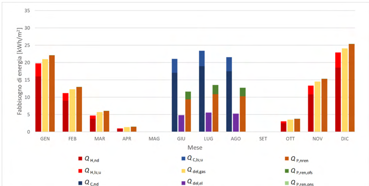
Figura 63. Fabbisogno di energia termica, erogata e primaria per riscaldamento e raffrescamento - Milano (regime continuo) Soluzione 1
