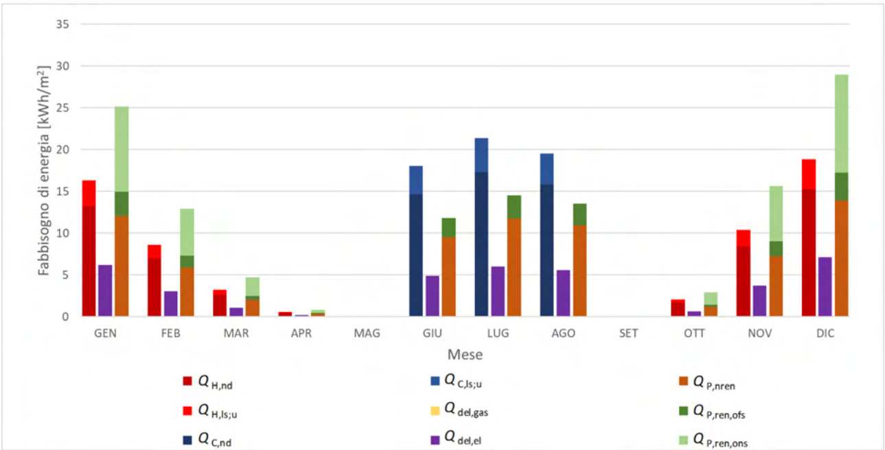
Figura 66. Fabbisogno di energia primaria per riscaldamento e raffrescamento - Milano (regime intermittente) Soluzione 2
