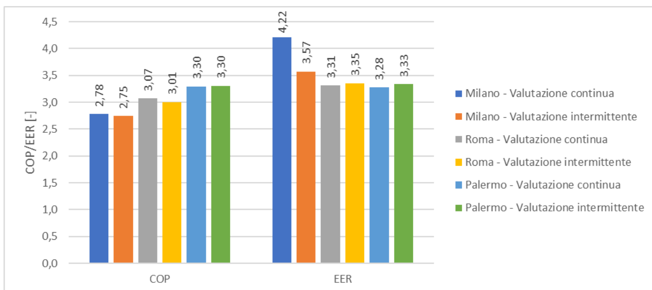
Figura 79. Valori di COP ed EER – Risultati annuali
