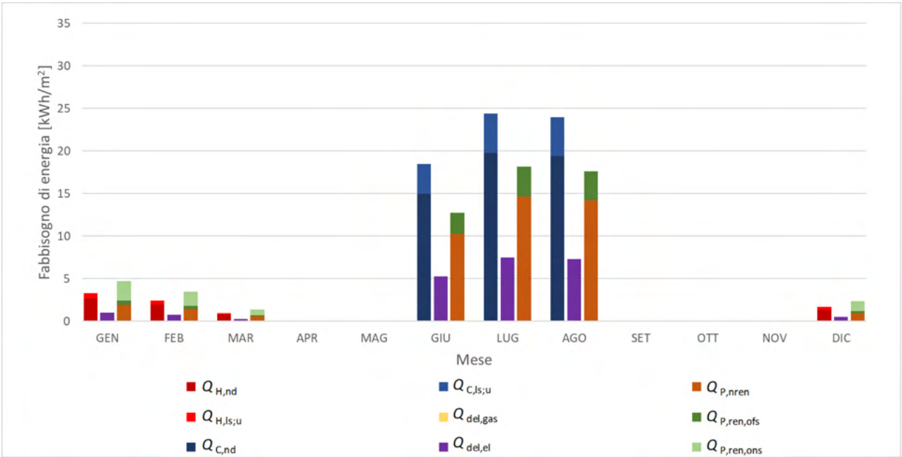
Figura 74. Fabbisogno di energia primaria per riscaldamento e raffrescamento - Palermo (regime intermittente) Soluzione 2
