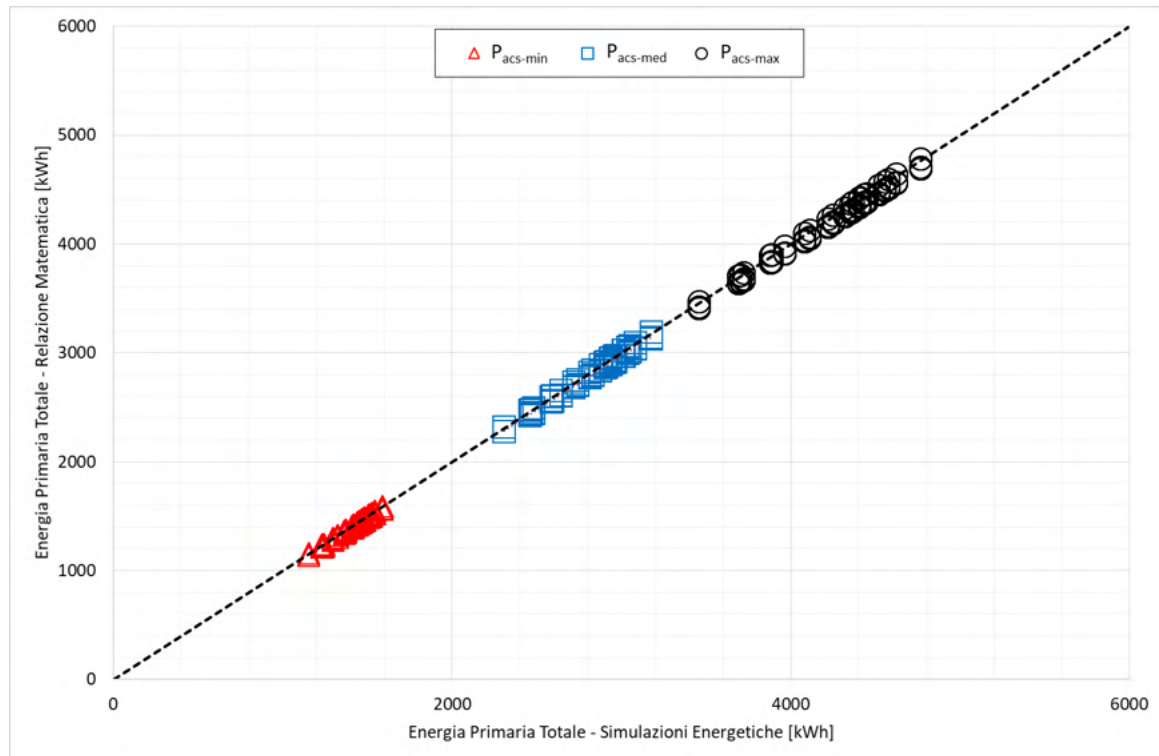
Figura 55 – Confronto tra l'energia primaria restituita per i tre profili di utilizzo nelle simulazioni energetiche e quella calcolata a partire dall'Equazione 2.
