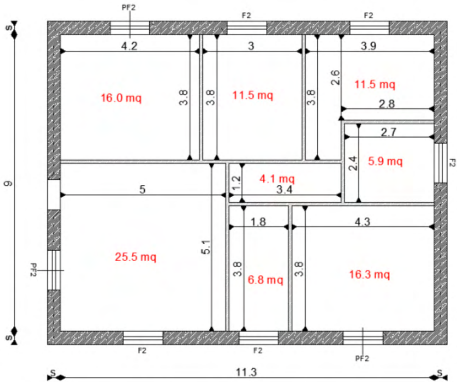
Figura 11 – Pianta geometrica del caso studio E1.i.U.1: edificio isolato unifamiliare di superficie di circa 100 m².
