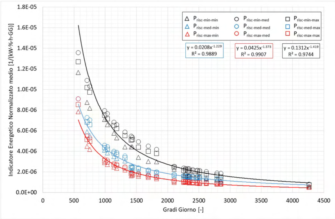
Figura 88 – Trend dell’indicatore energetico normalizzato medio tailored rispetto i Gradi Giorno: edifici in cemento armato con livello di isolamento Liv-Iso-0.
