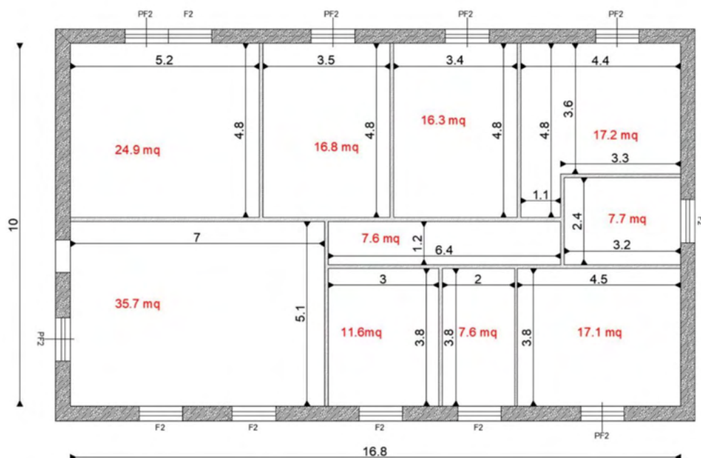
Figura 14 – Pianta geometrica del caso studio E1.i.U.3: edificio isolato unifamiliare di superficie di 168 m 2 .
