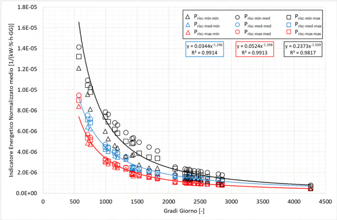
Figura 87 – Trend dell’indicatore energetico normalizzato medio tailored rispetto i Gradi Giorno: edifici in muratura portante con livello di isolamento Liv-Iso-0.
