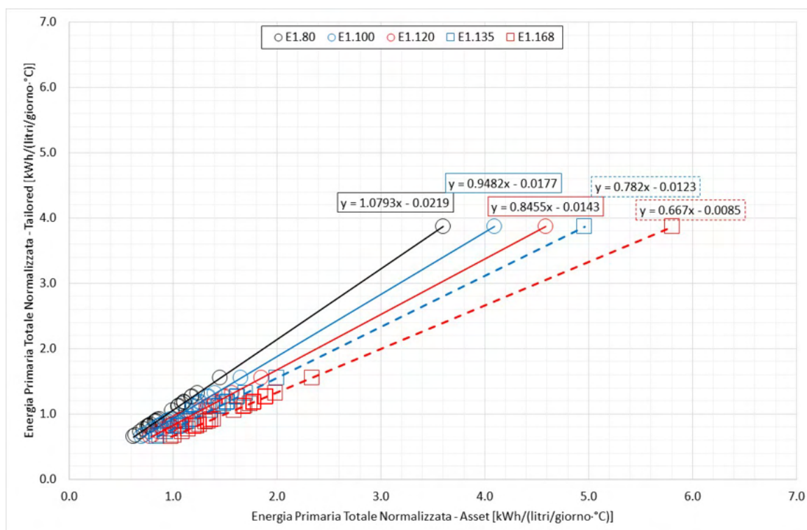
Figura 51 – Confronto dell'energia primaria per la produzione acqua calda sanitaria normalizzata rispetto al volume di acqua consumato e la temperatura media annuale: asset rating vs tailored rating.
