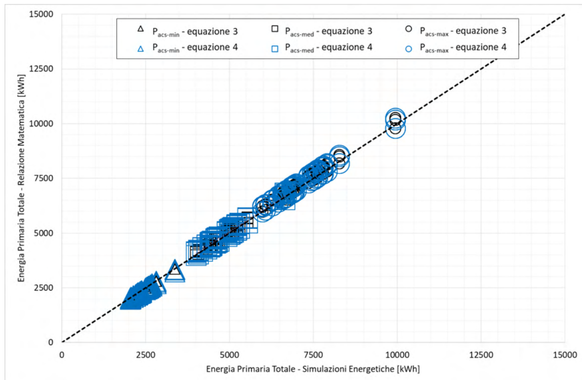
Figura 46 – Confronto tra l'energia primaria restituita per i tre profili di utilizzo nelle simulazioni energetiche e quella calcolata a partire dall'Equazione 3 e dall'Equazione 4.
