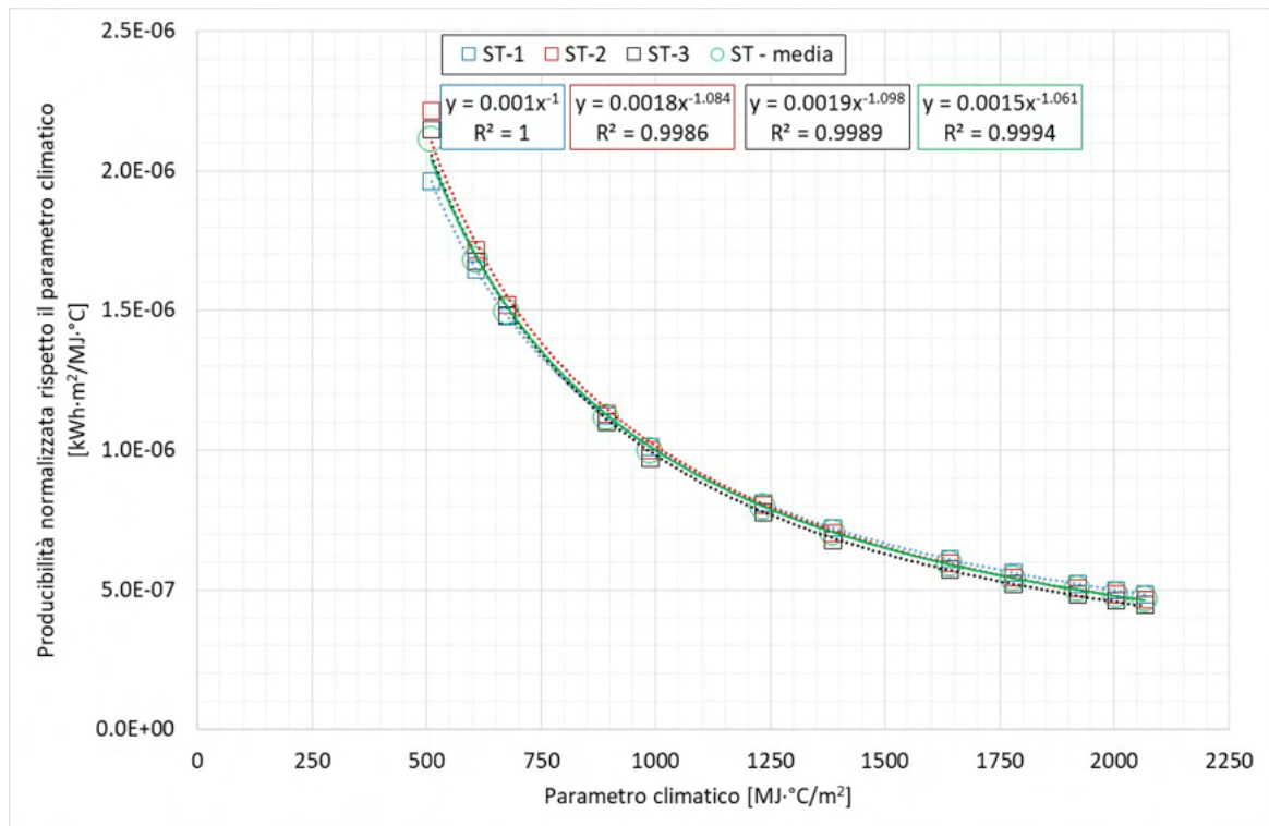
Figura 58 – Producibilità normalizzata in funzione del parametro climatico.
