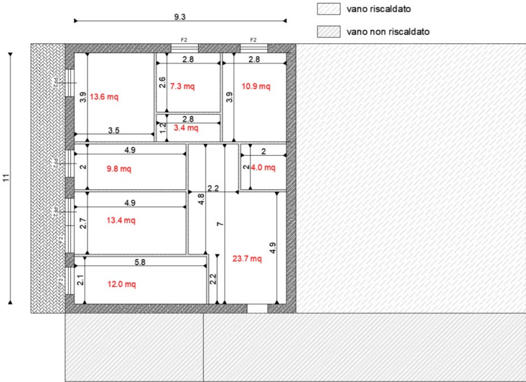
Figura 20 – Pianta geometrica dei casi studio E2.t.PT.2, E2.t.PI.2 ed E2.t.PU.2: unità immobiliari in un edificio a torre di superficie pari 100 m².
