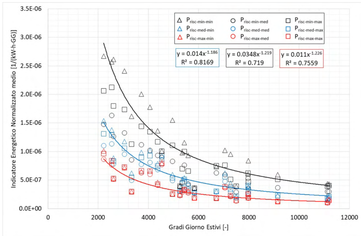
Figura 111 – Trend dell'indicatore energetico normalizzato medio tailored rispetto i Gradi Giorno Estivi: edifici caratterizzati da un livello di isolamento Liv-Iso-1.
