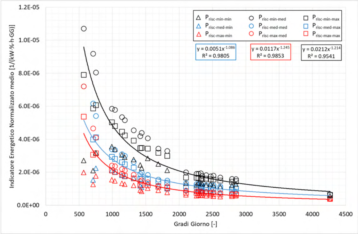
Figura 89 – Trend dell’indicatore energetico normalizzato medio tailored rispetto i Gradi Giorno: edifici con livello di isolamento Liv-Iso-02.
