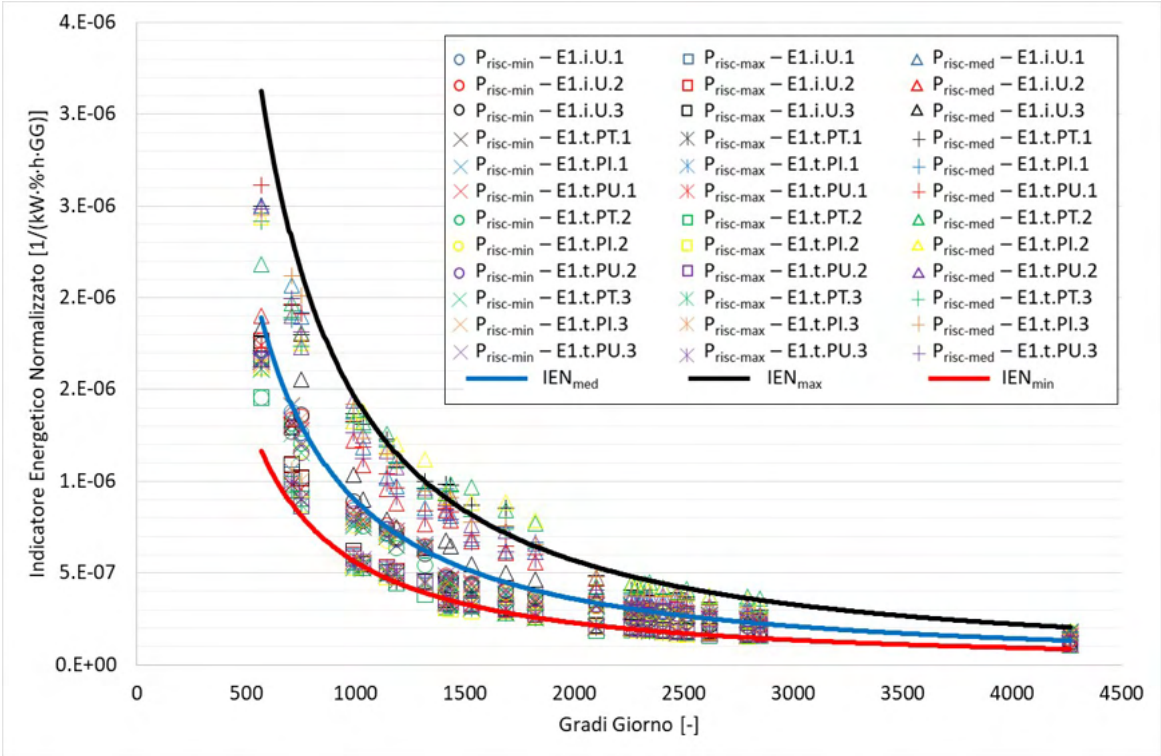
Figura 100 – Trend dell’indicatore energetico normalizzato tailored rispetto i Gradi Giorno: edifici caratterizzati da un livello di isolamento Liv-Iso-3.
