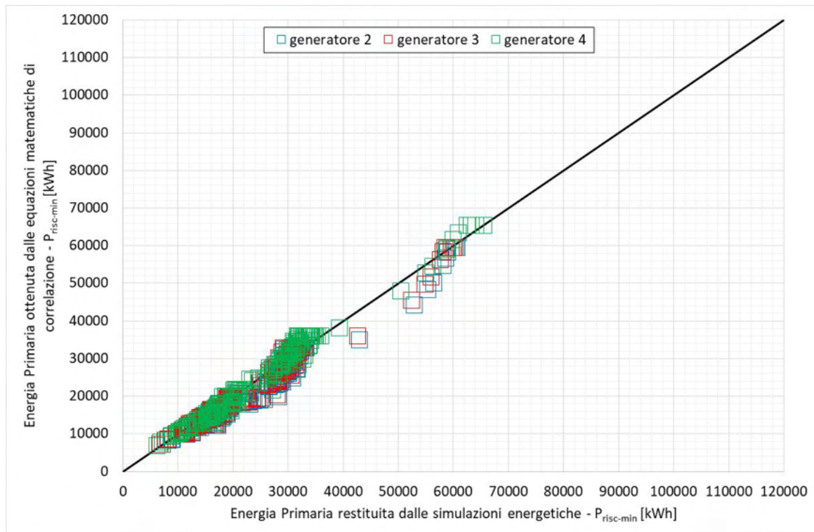
Figura 84 – Confronto tra energia primaria simulata e quella restituita dall'Equazione 12 con il profilo P_{risc-min} per i generatori di calore 2, 3 e 4 operanti ad alta temperatura: casi studio E1.i ed E1.t con livello di isolamento Liv-Iso-0.
