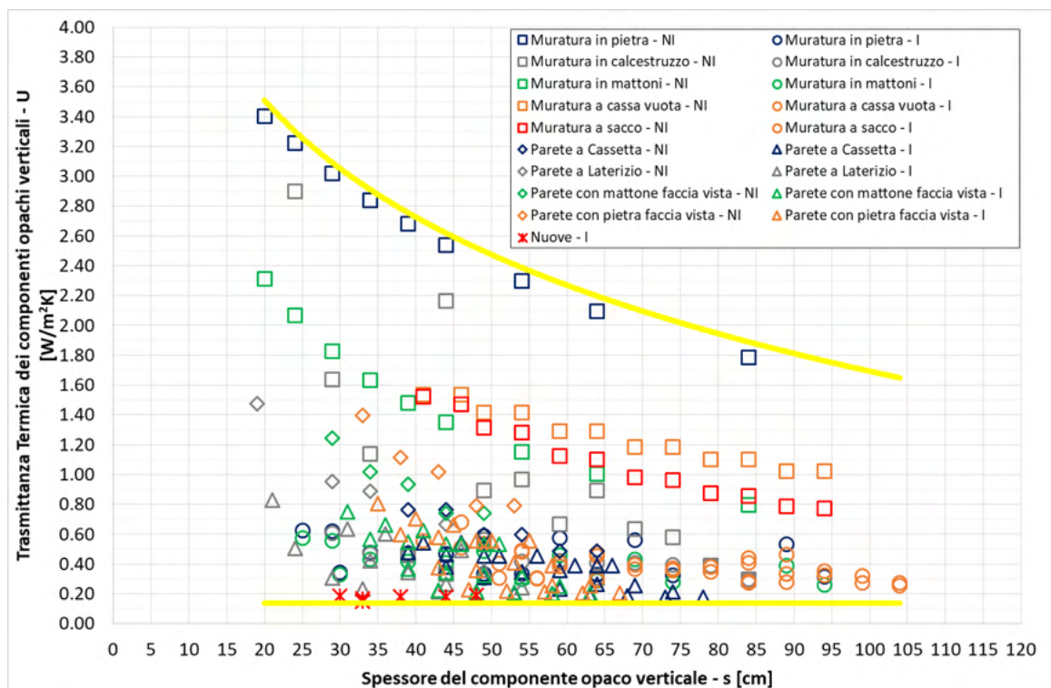
Figura 25 – Analisi delle caratteristiche termiche medie delle componenti opache verticali selezionate in [1].
