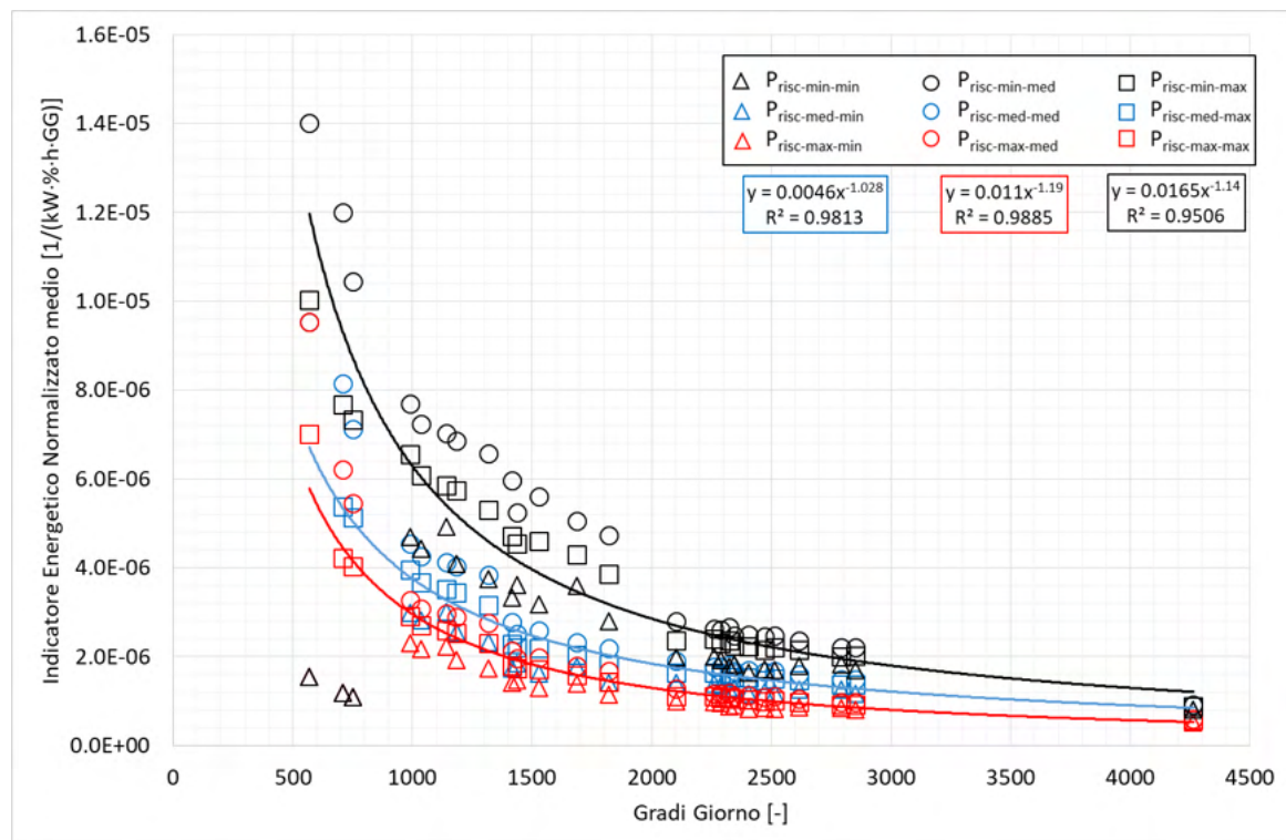
Figura 76 – Trend dell'indicatore energetico normalizzato medio tailored rispetto i Gradi Giorno: edifici caratterizzati da un livello di isolamento Liv-Iso-2.
