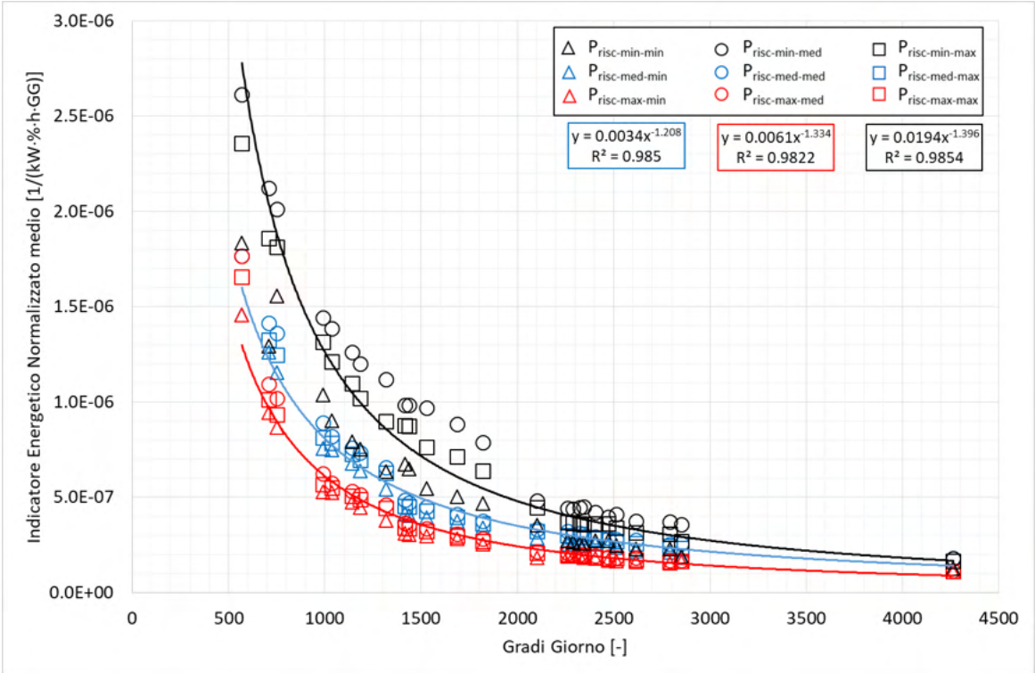
Figura 101 – Trend dell’indicatore energetico normalizzato medio tailored rispetto i Gradi Giorno: edifici caratterizzati da un livello di isolamento Liv-Iso-3.
