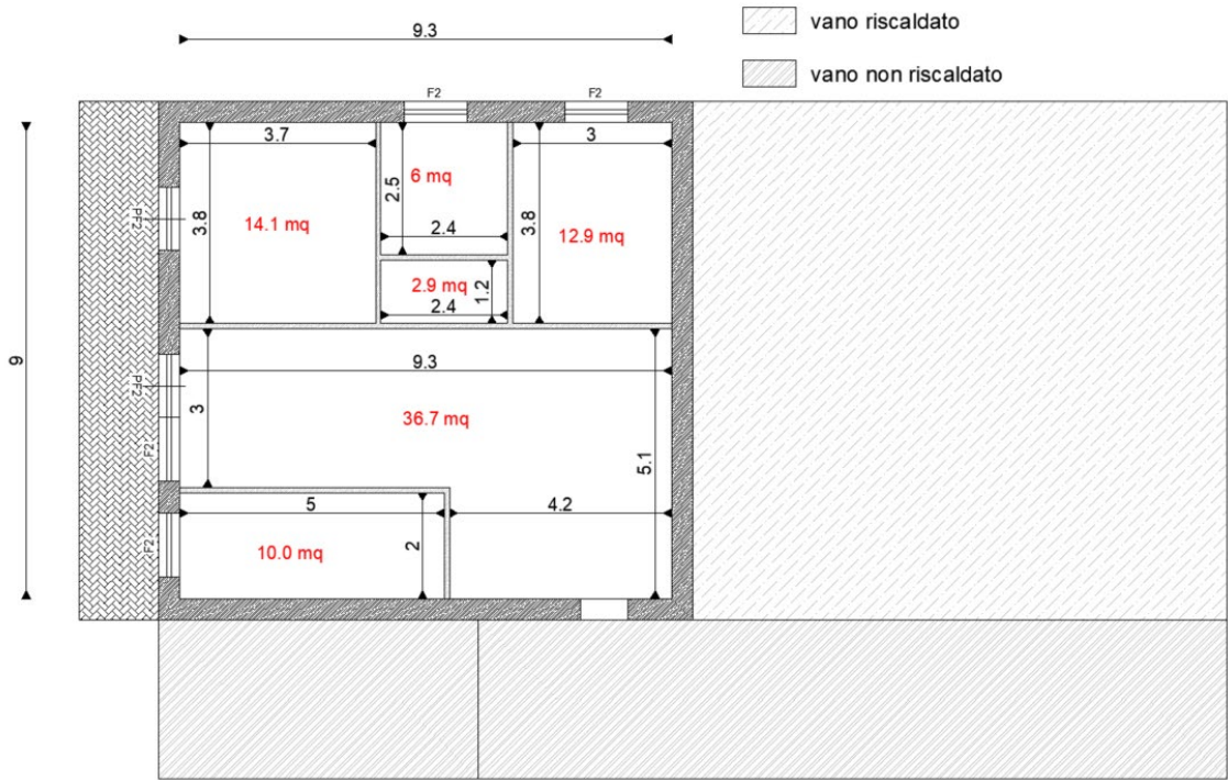
Figura 15 – Pianta geometrica dei casi studio E1.t.PT.1, E1.t.PI.1 ed E1.t.PU.1: unità immobiliari in un edificio a torre plurifamiliare di superficie pari a 80 m².
