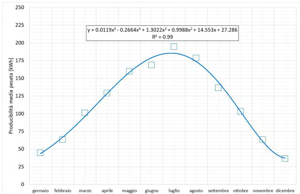
Figura 59 – Producibilità media pesata del solare termico.
