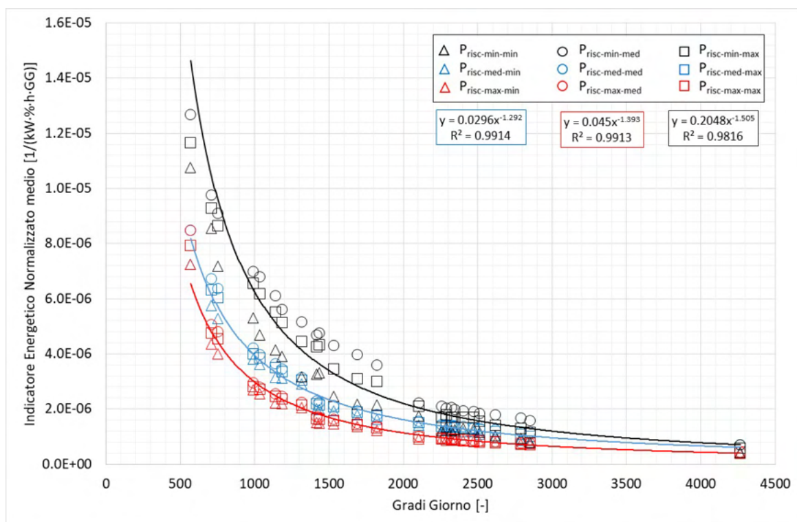
Figura 91 – Trend dell'indicatore energetico normalizzato medio tailored rispetto i Gradi Giorno: edifici con livello di isolamento Liv-Iso-03.
