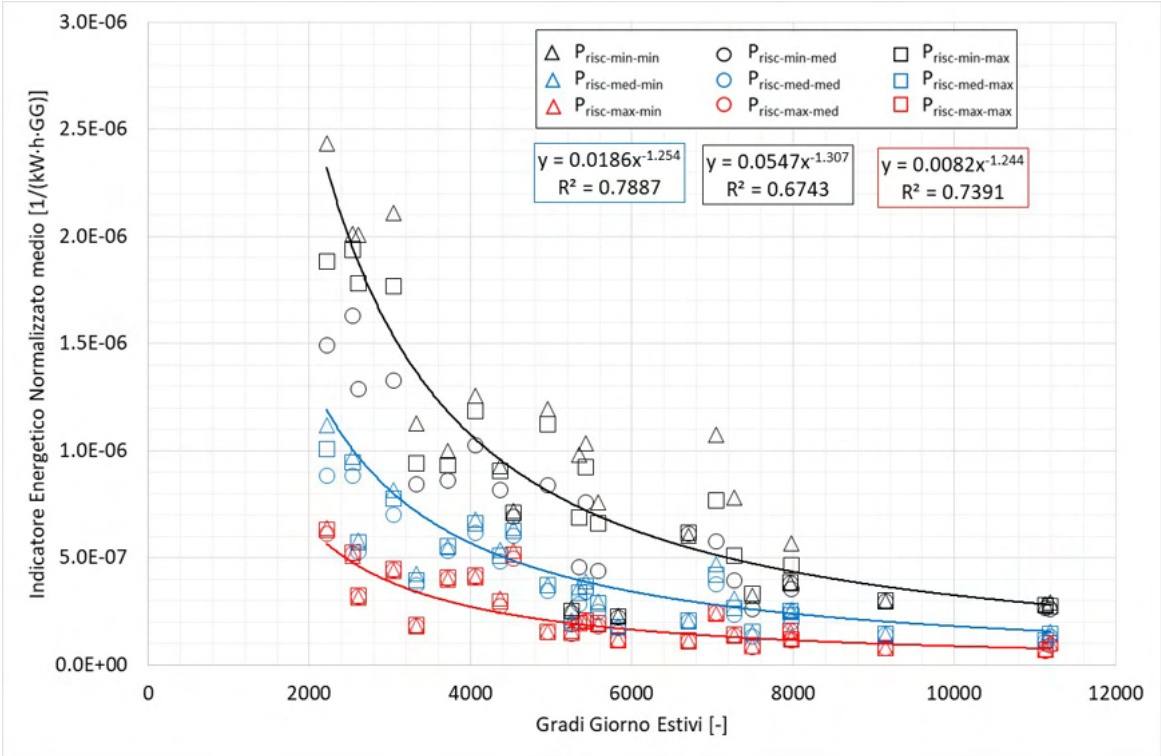
Figura 112 – Trend dell’indicatore energetico normalizzato medio tailored rispetto i Gradi Giorno Estivi: edifici caratterizzati da un livello di isolamento Liv-Iso-2.
