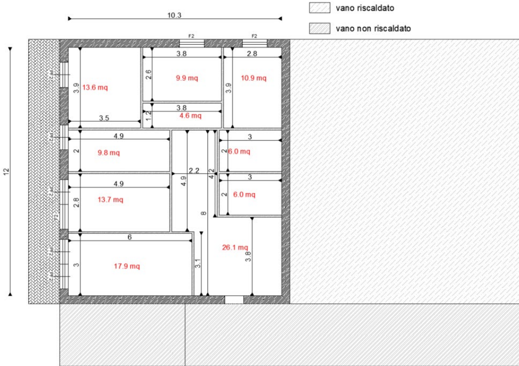
Figura 21 – Pianta geometrica dei casi studio E2.t.PT.3, E2.t.PI.3 ed E2.t.PU.3: unità immobiliari in un edificio a torre di superficie pari 120 m².
