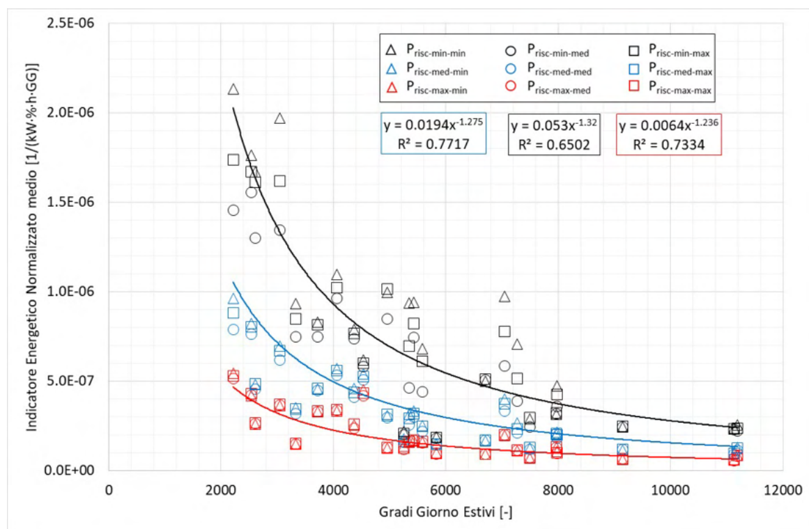
Figura 113 – Trend dell'indicatore energetico normalizzato medio tailored rispetto i Gradi Giorno Estivi: edifici caratterizzati da un livello di isolamento Liv-Iso-3.
