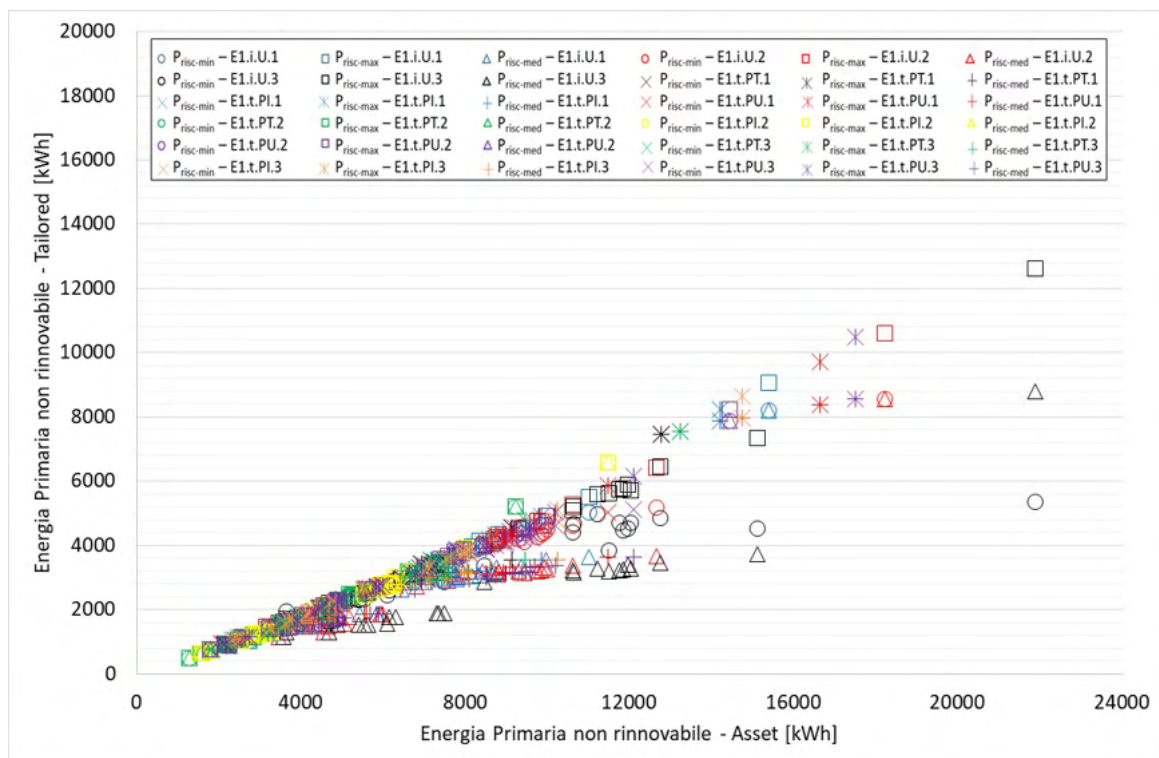
Figura 99 – Confronto tra energia primaria calcolata con il profilo asset e quella restituita con i tre profili tailored: edifici caratterizzati da un livello di isolamento Liv-Iso-3.
