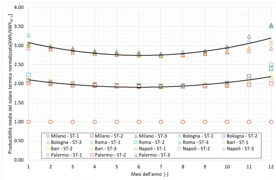
Figura 57 – Produttività del solare termico normalizzata rispetto la configurazione ST-1.
