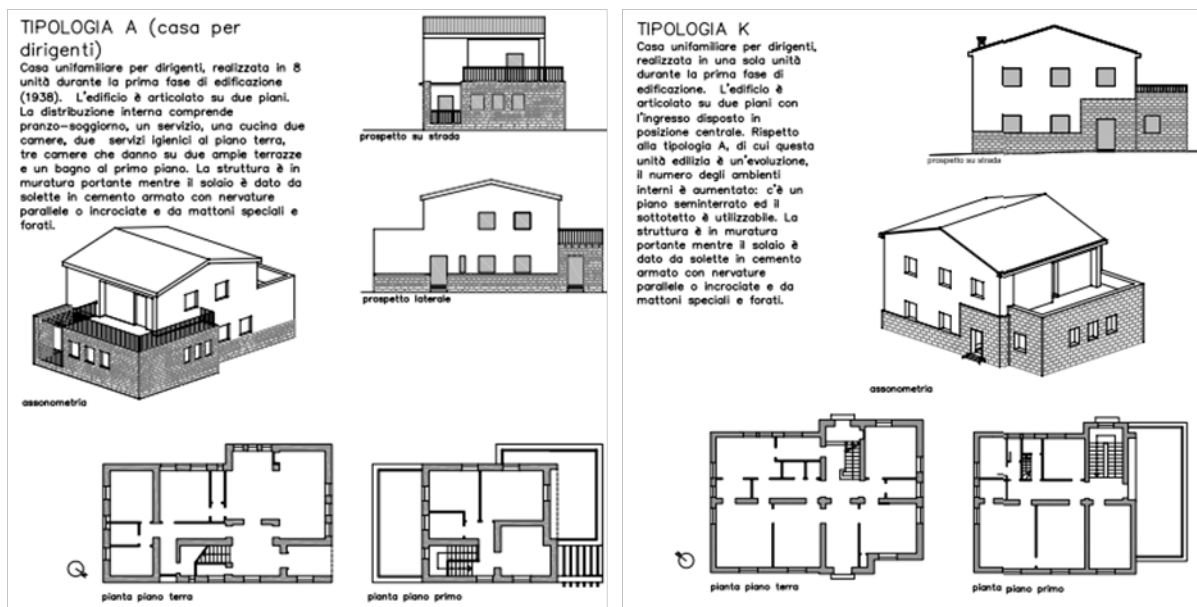
Figura 10 - Tipo generico della Fondazione "Gen_Fond_2", case unifamiliari della fondazione su due livelli: tipo A, Tipo K
