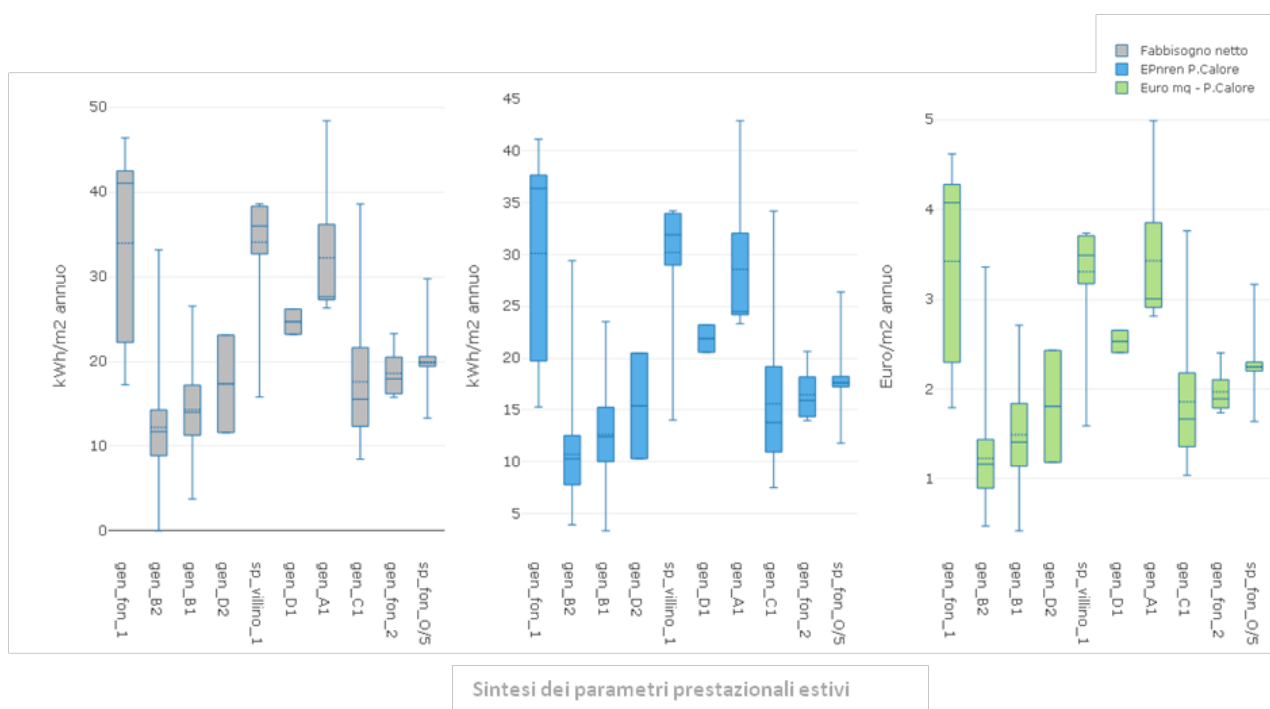
Figura 4.74 – Sintesi del fabbisogno per raffreddamento e delle performance con i sistemi più diffusi
