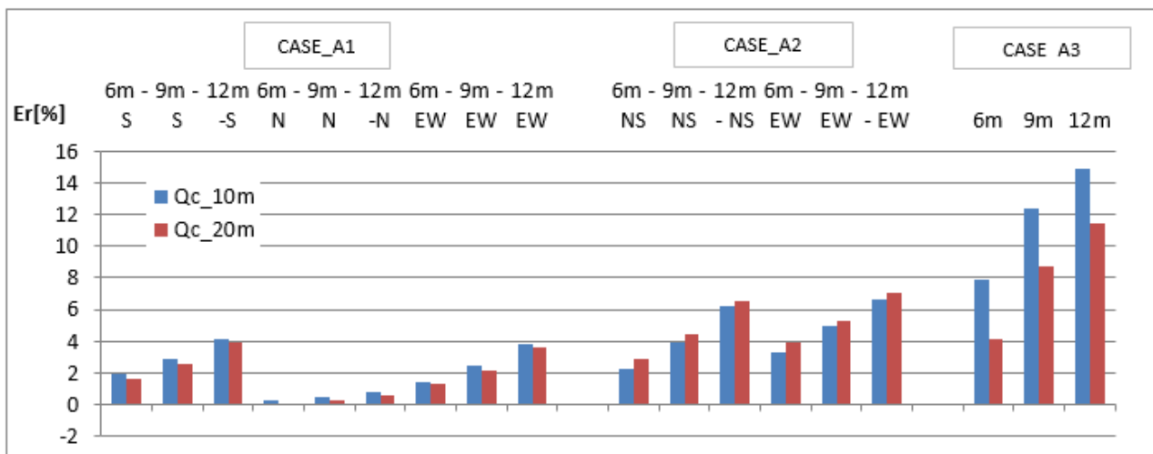
Figura 4.75 - Casi A, variazione [%] del Qh e del Qc stimati da UBEP_11300 e DOCET3 nei casi CASE_A
