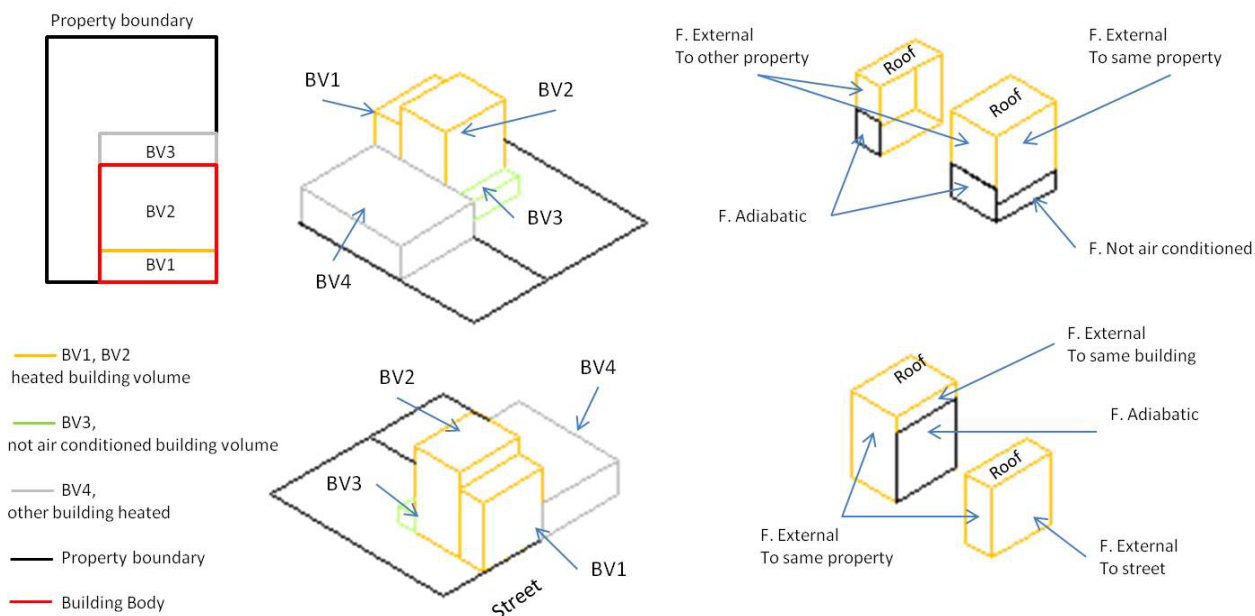
Figura 3.6 – Definizione dei volumi edilizi (VE) e delle Unità Edilizie (BB)
