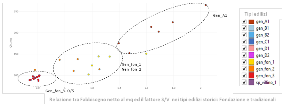
Figura 4.69 – Relazione fattore forma S/V e fabbisogno netto
