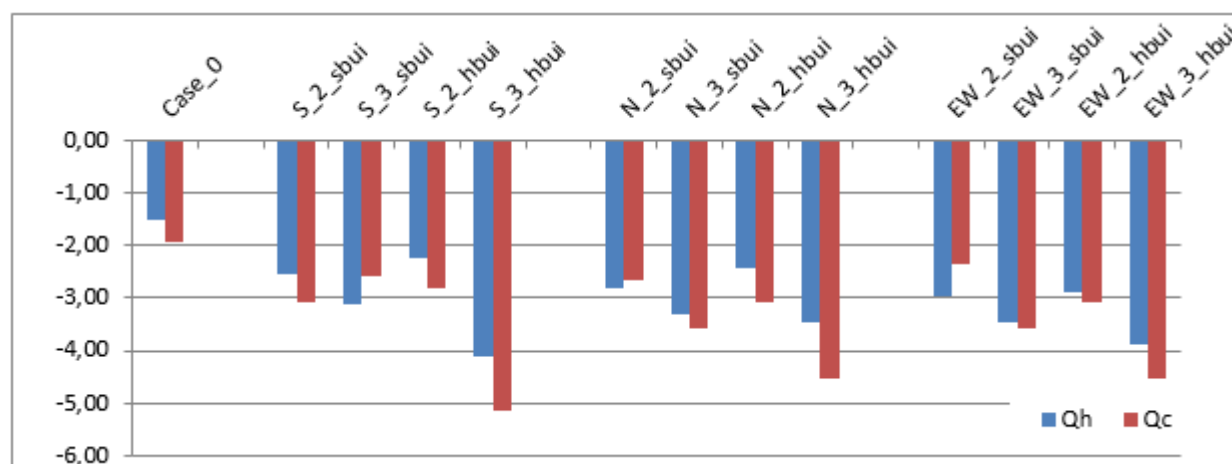
Figura 4.78 - CASO_C, Confronto del Fabbisogno netto al mq estivo ed invernale ( Q_h , Q_c )
