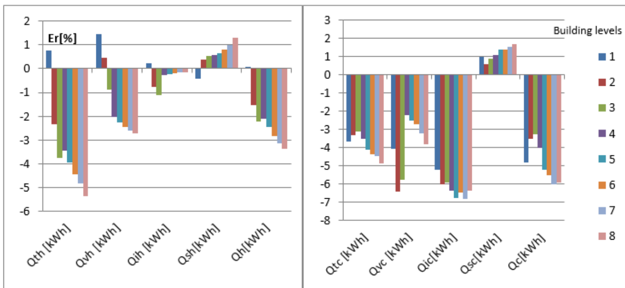
Figura 4.77 - Comparazione tra i fattori delle (1) e (2) calcolati da UBEP_11300 and DOCET3 (CASO_B)
