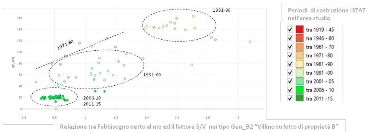
Figura 4.70 – Relazione fattore forma S/V e fabbisogno netto nelle tipologie storiche e negli edifici isolati Gen_B1, Gen_b2
