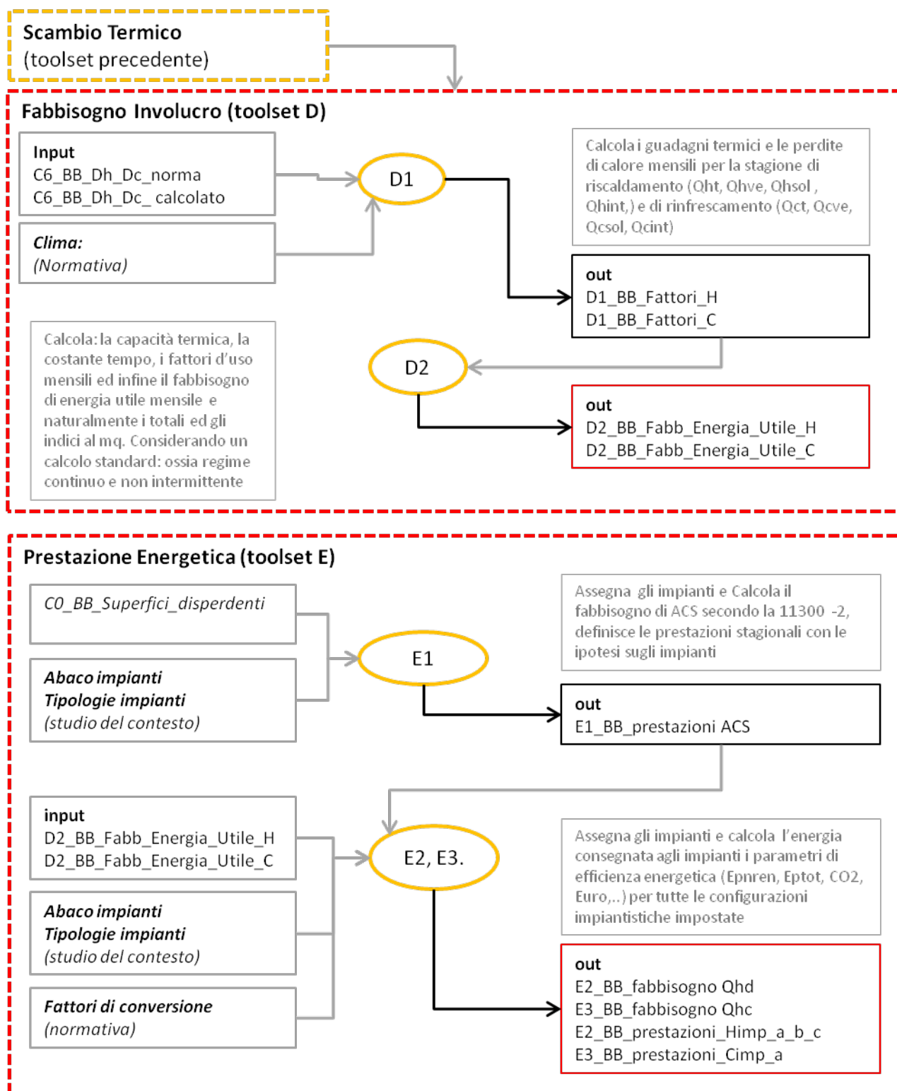
Figura 3.16 – Struttura dei toolset D ed E per il calcolo dei fabbisogni energetici
