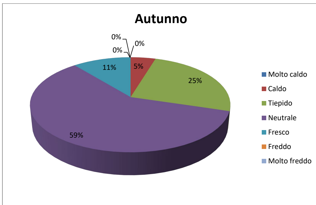
Figura 4.51 - Sensazione termica percepita all'interno dell'abitazione durante la stagione autunnale
