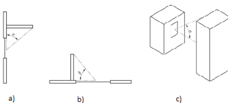
Figura 3.9 – Definizione dell'angolo di ostruzione: a) e b) ostruzioni orizzontali e verticali dell'edificio, c) ostruzioni esterne.
