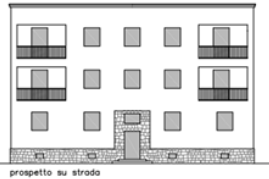
prospetto su strada
