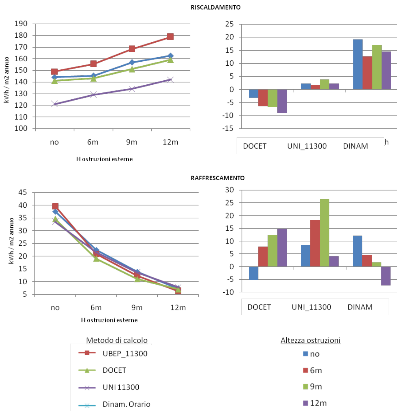
Figura 4.71 - Confronti del Fabbisogno netto ( Q_h , Q_c ) con i diversi software di controllo nel caso A3 ( D=10 )
