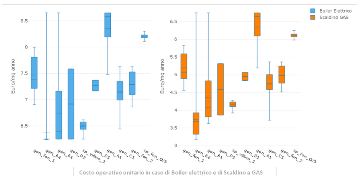
Figura 4.73 – Sintesi del fabbisogno per ACS, e delle performance con i sistemi più diffusi
