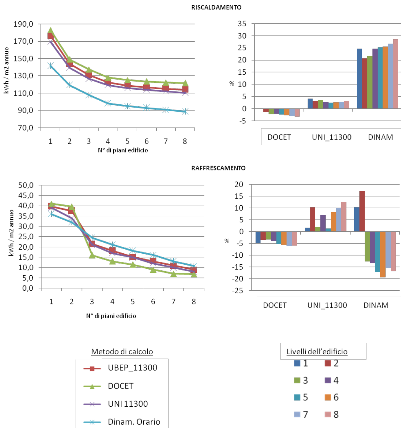
Figura 4.72 - Confronto del Fabbisogno netto (Qh, Qc) con i diversi software di controllo nel Caso B
