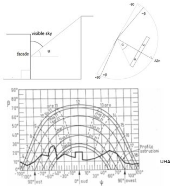
Figura 3.11 - Generica ostruzione di estensione angolare +/- \alpha , angolo di ostruzione u e vista di estensione +/- \beta
