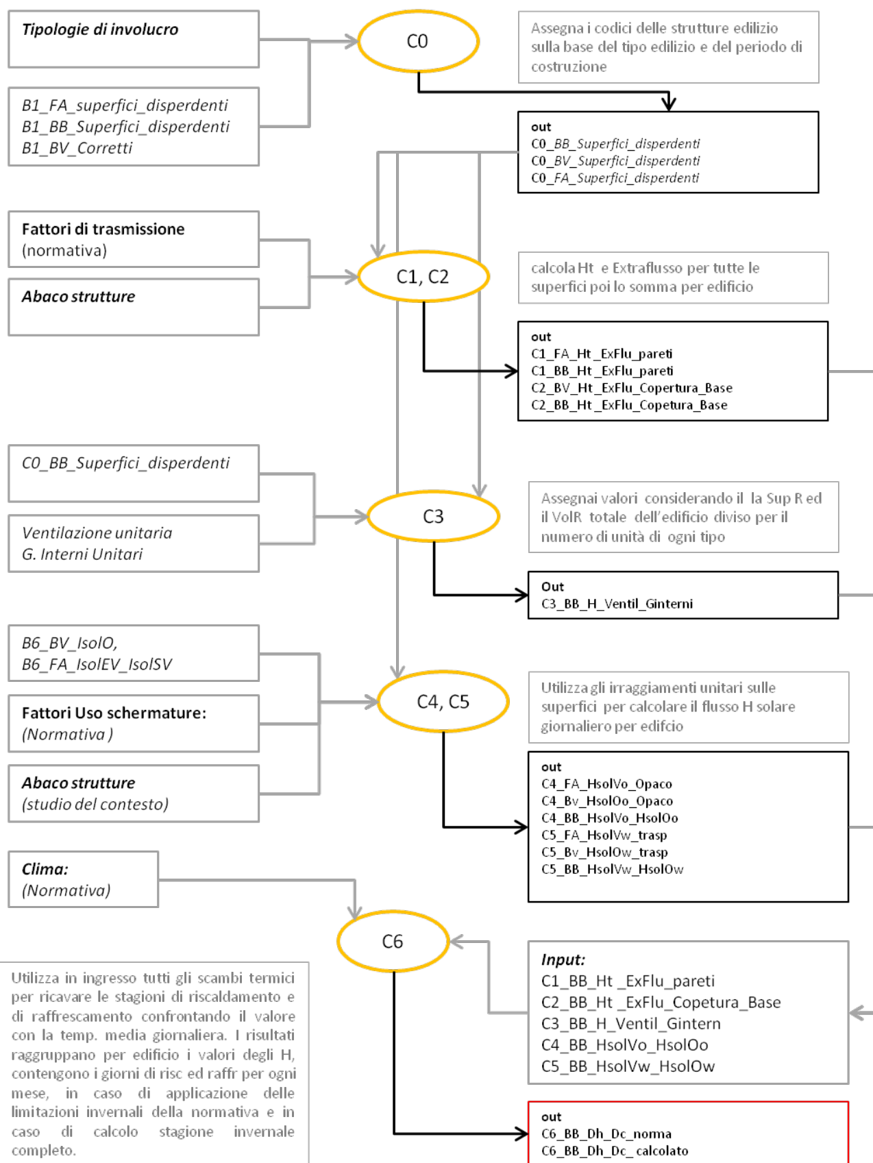
Figura 3.15 – Struttura del toolset C per il calcolo degli scambi termici
