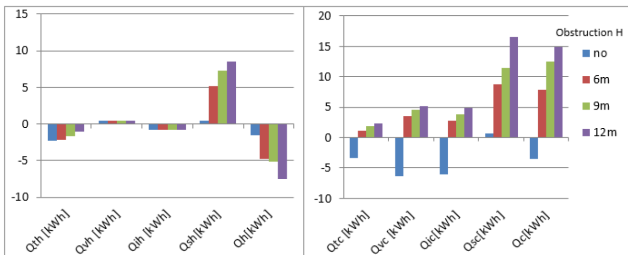
Figura 4.76 - Comparazione tra i fattori delle (1) e (2) calcolati da UBEP_11300 and DOCET3 (CASE_A3, D 10m)
