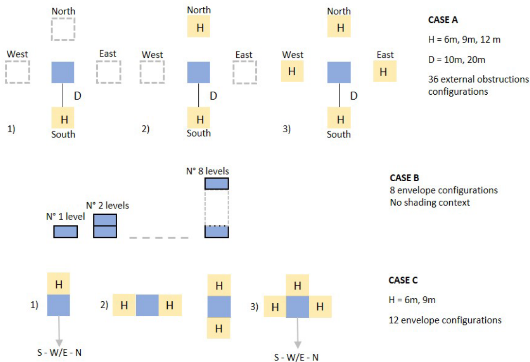
Figura 3.17 – Configurazione dei casi ideali utilizzati per la validazione
