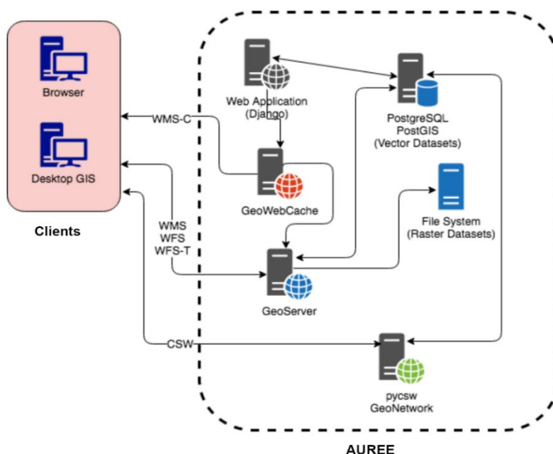
Figura 5.2 – Architettura AUREE
