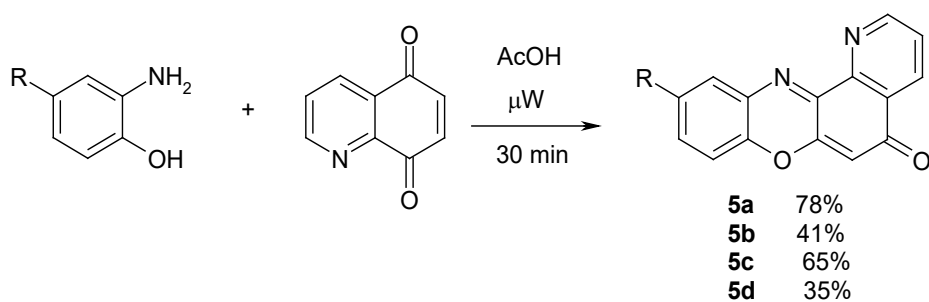
Figura 34. Procedura sintetica ottimizzata per la preparazione dei derivati piridofenossazinonici 5a-d.
