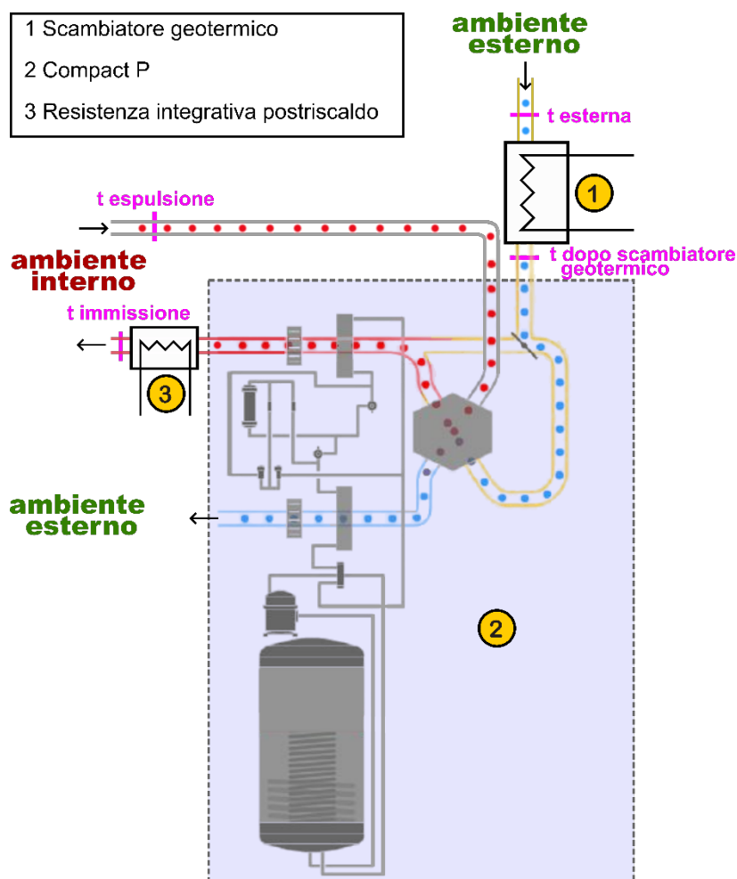
Figura 4-7 Schema impiantistico in cui sono evidenziate i punti in cui le temperature sono misurate
