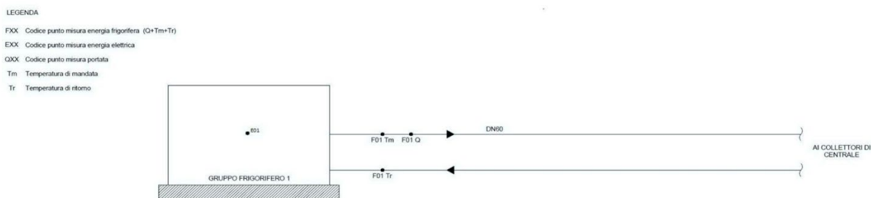
Figura 5-9 Schema funzionale della centrale frigorifera del condominio Corte Sara
