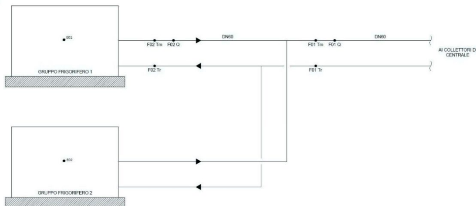
Figura 5-7 Schema funzionale della centrale frigorifera del condominio Corte Veronica
