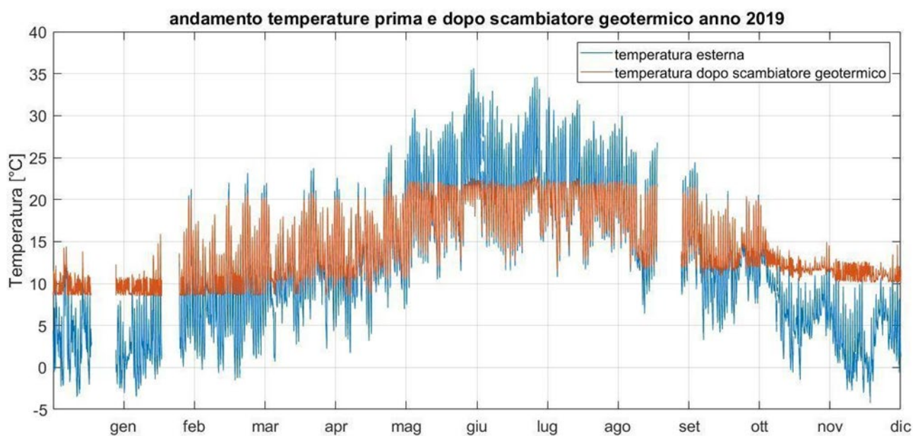
Figura 4-4 Andamento annuale delle temperature prima e dopo lo scambiatore geotermico
