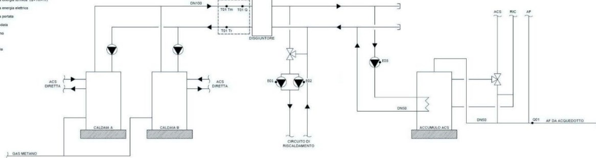
Figura 5-8 Schema funzionale della centrale termica del condominio Corte Sara
