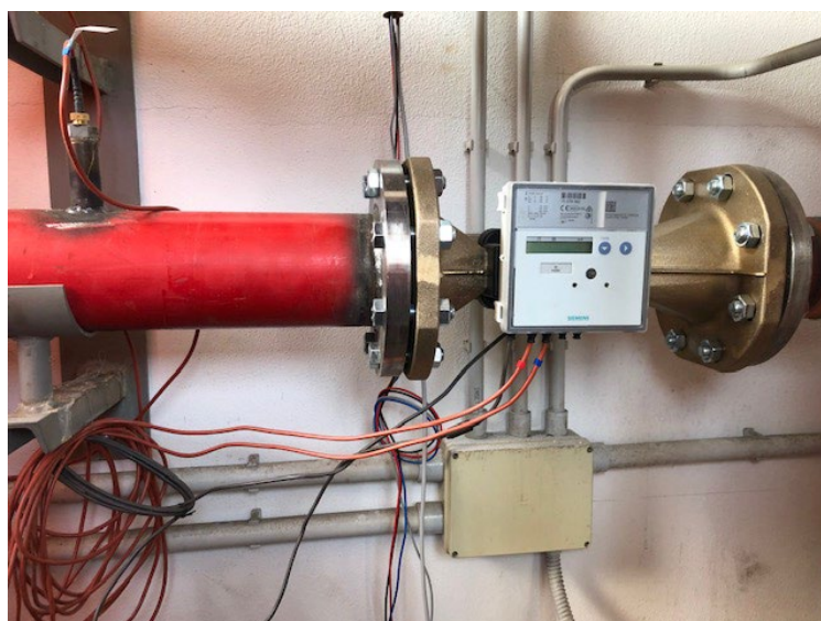
Figura 5-13 Sensore Siemens installati all'interno della centrale termica di Corte Sara a monte del disgiuntore (T01)
