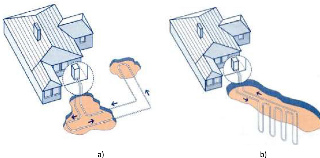
Figura 1-3 Impianto geotermico ad assetto (a) orizzontale e (b) verticale
