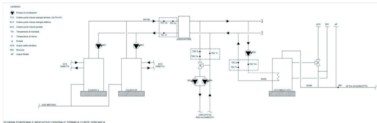
Figura 5-3 Schema funzionale dell'impianto di riscaldamento del condominio Corte Veronica
