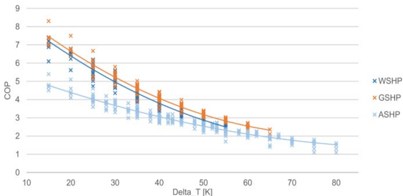
Figura 2-6 Stima delle curve COP. Le regressioni quadratiche vengono eseguite sui dati del produttore distinguendo tra pompe di calore aerotermiche (ASHP), pompe di calore geotermiche (GSHP) e pompe di calore idrotermiche (WSHP)
