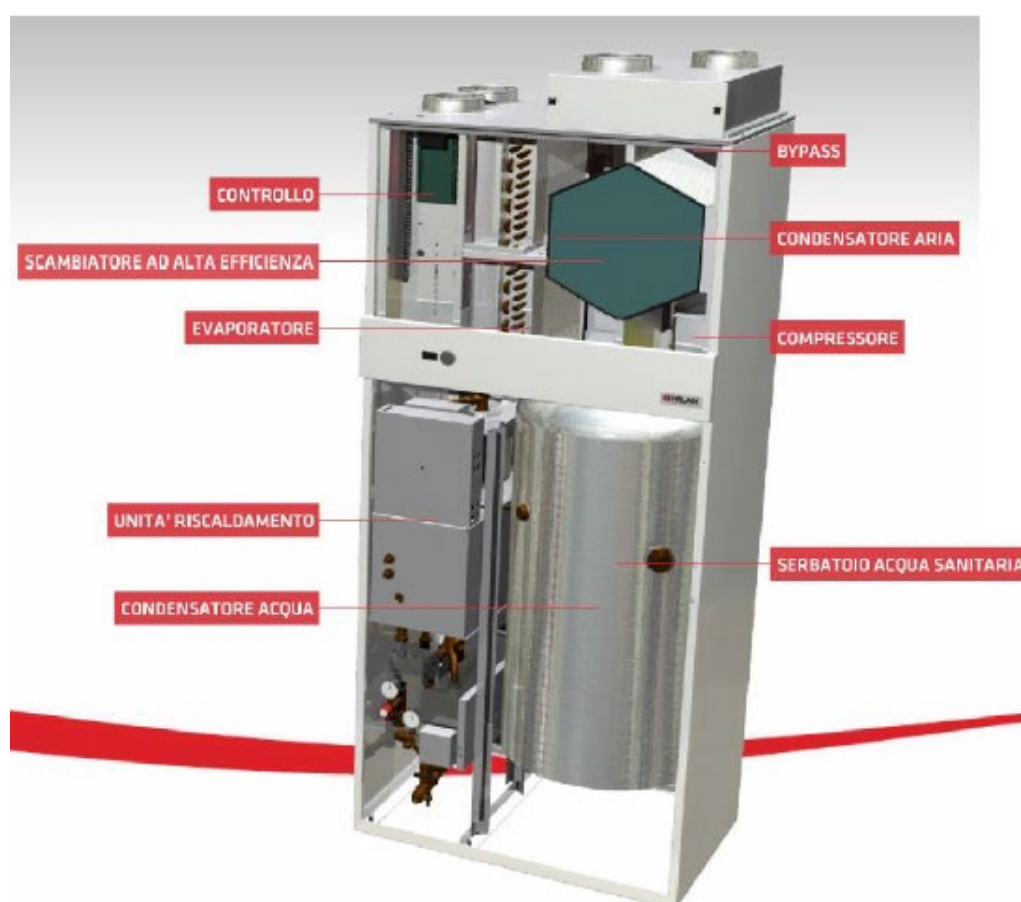
Figura 4-5 Dettaglio dei componenti costituenti l'unità Compact P
