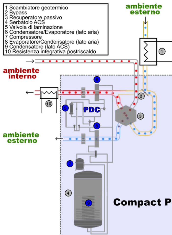
Figura 4-6 Schema di dettaglio dei componenti interni del Compact P
