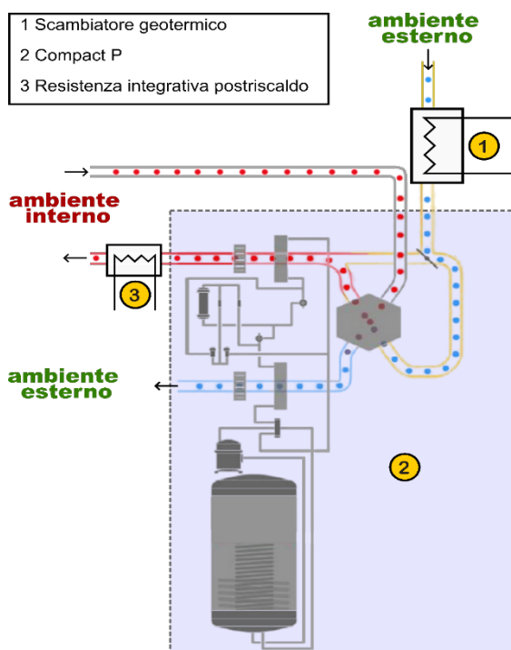
Figura 4-3 Schema dell'impianto di condizionamento, ventilazione e produzione di ACS
