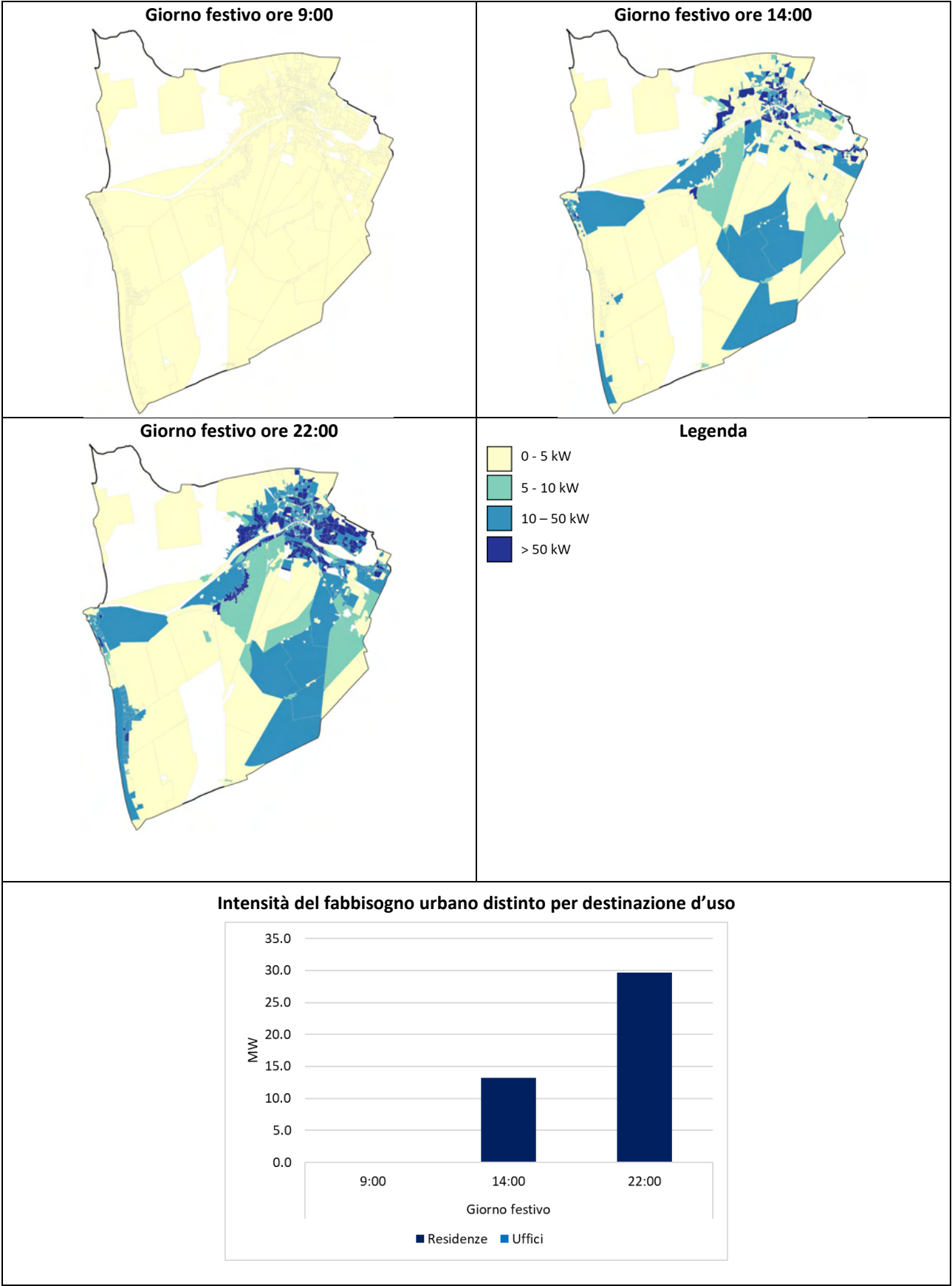
Figura 45. Intensità del fabbisogno termico di raffrescamento in un giorno festivo di luglio.
