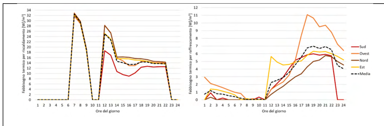
Figura 14. Profili di densità di fabbisogno termico per riscaldamento (sinistra) e raffrescamento (destra) per una ZTT residenziale degli anni '60-'80.
