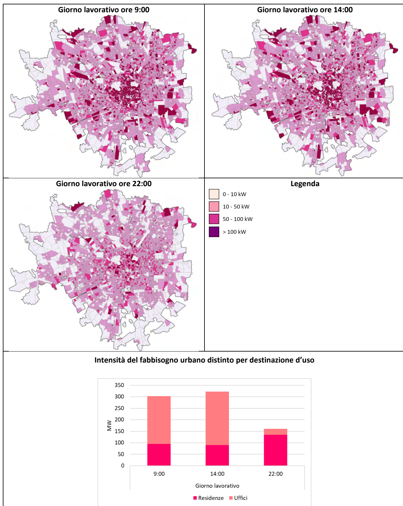
Figura 68. Intensità del consumo di energia finale di elettricità in un giorno lavorativo di luglio.
