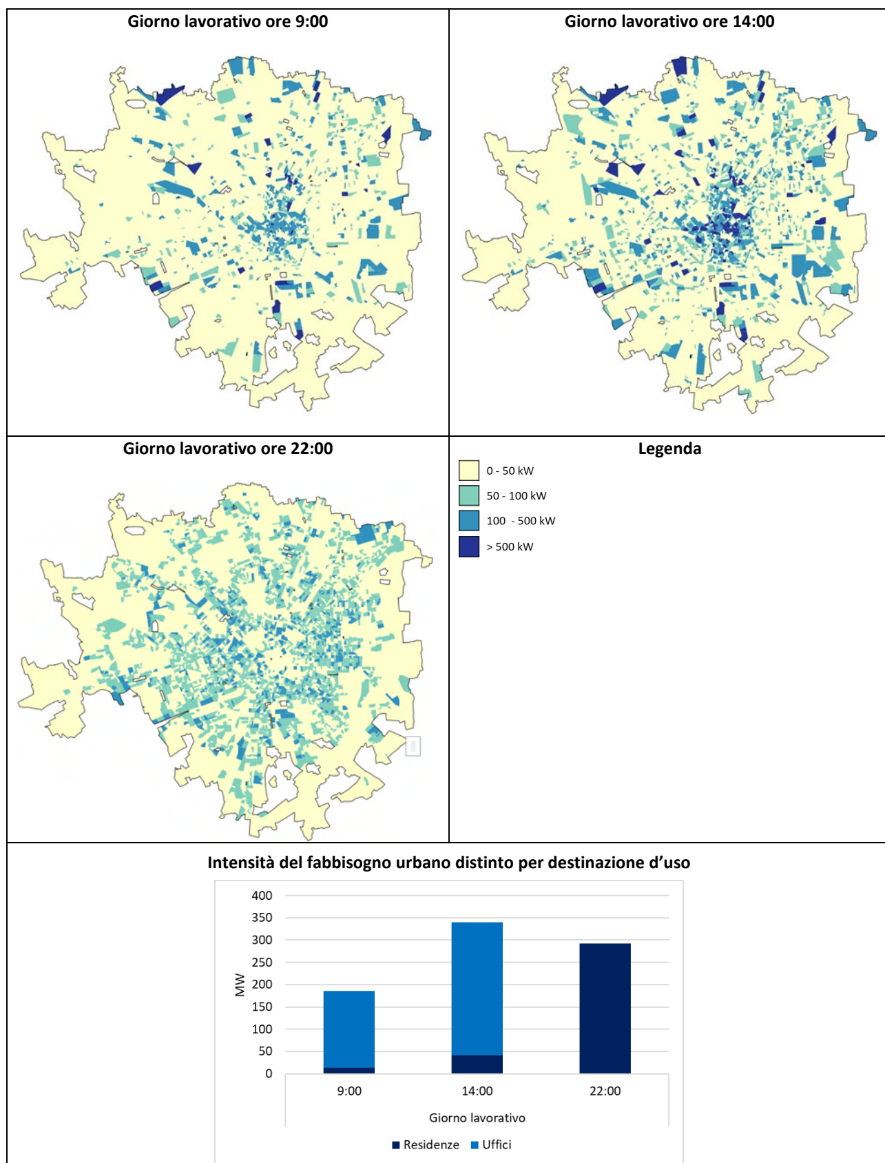
Figura 28. Intensità del fabbisogno termico per raffrescamento in un giorno lavorativo di luglio.
