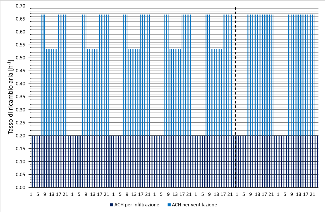
Figura 5. Profilo settimanale del tasso di ricambio aria per gli edifici ad uso residenziale da ISO 17772.
