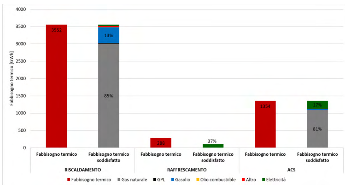
Figura 70. Fabbisogni termici del volume costruito ad uso residenziale ripartiti per fonte energetica.
