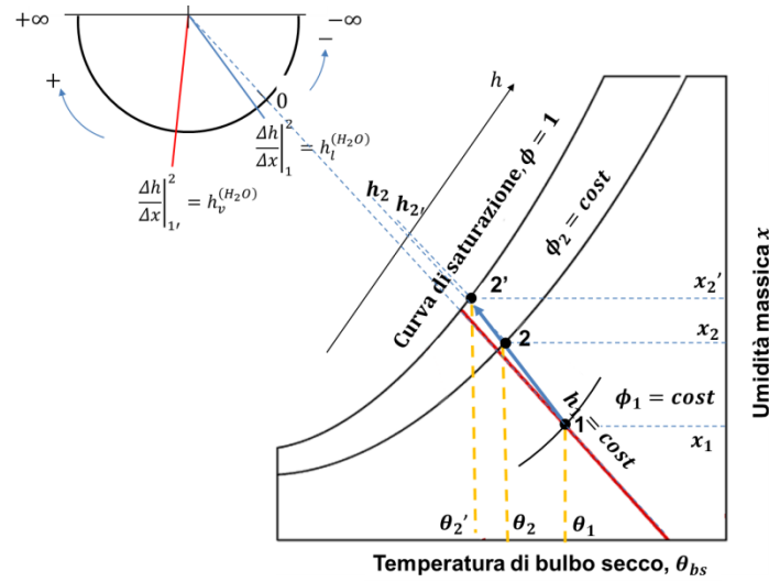
Figura 2 – Trasformazione di saturazione adiabatica di un'aria umida
