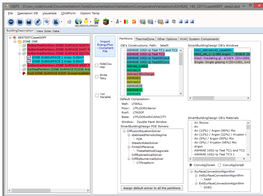
Figura 6 - Interfaccia grafica utente: GUI
