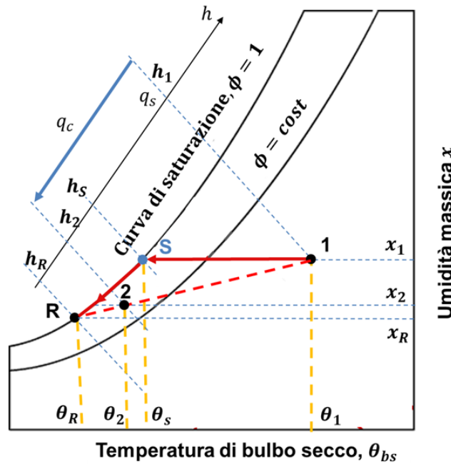
Figura 3 – Trasformazione raffreddamento con deumidificazione di un'aria umida
