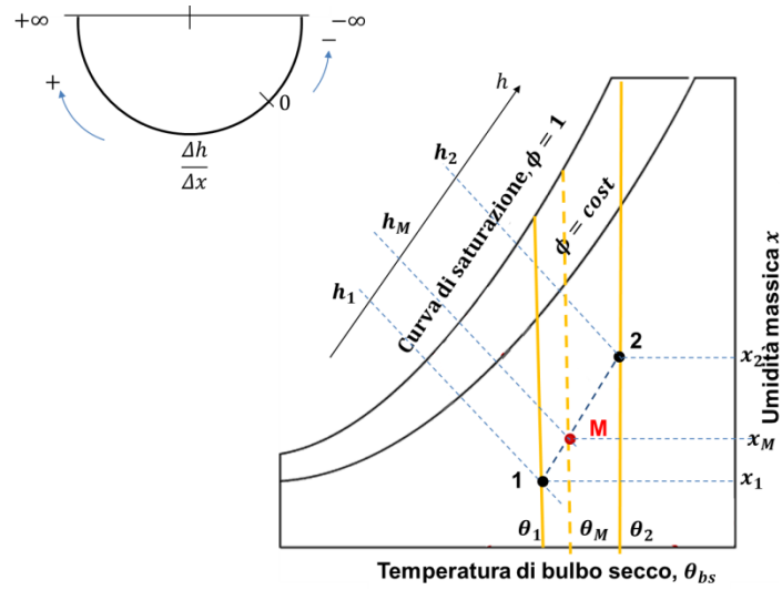
Figura 1 – Trasformazione miscelazione adiabatica di due arie umide
