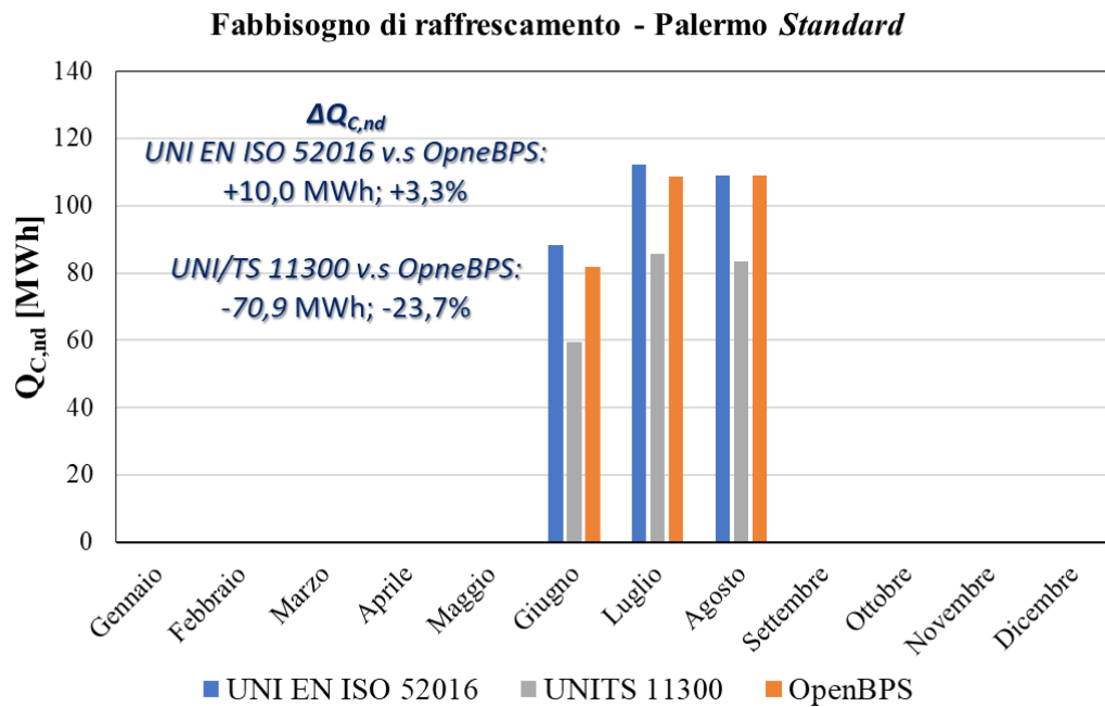
Figura 50. Fabbisogno di raffreddamento, UNI TS 11300, UNI EN ISO 52016, OpenBPS (V2) – valutazione Standard , Palermo.
