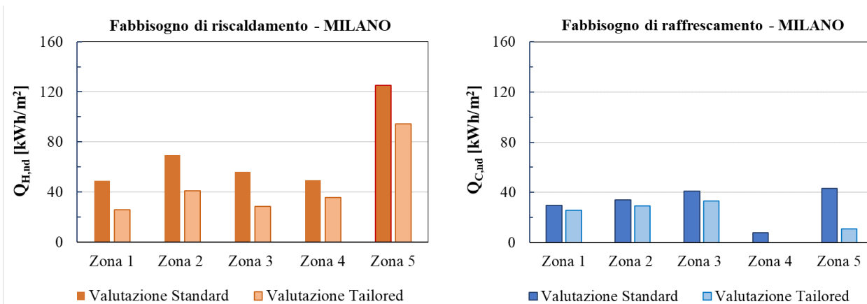
Figura 17. Fabbisogno di riscaldamento (sinistra) e raffrescamento (destra) relativo alle singole zone termiche e all'intero edificio – Milano, UNI TS 11300.
