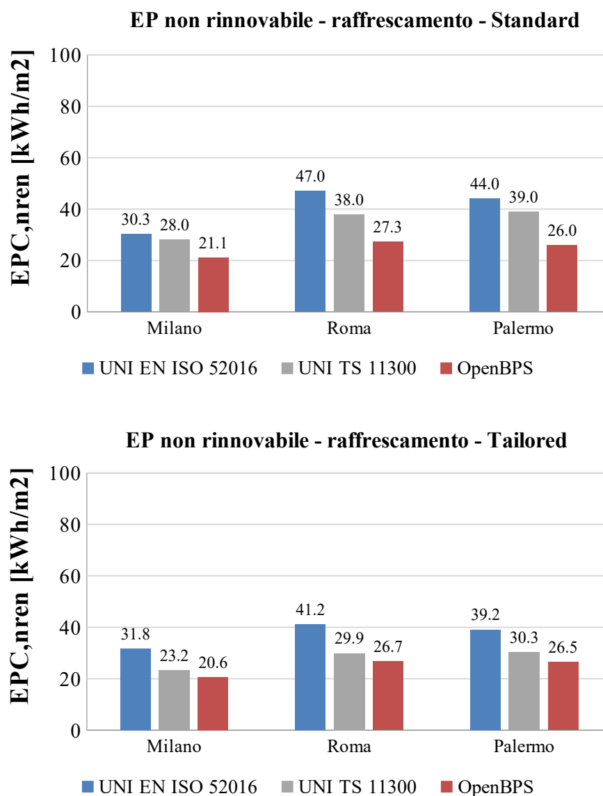
Figura58. Energia primaria non rinnovabile per raffrescamento - UNI TS 11300, UNI EN ISO 52016 ed OpenBPS (V2) – valutazione Standard e Tailored. Scenario 1/2: PdC reversibile.
