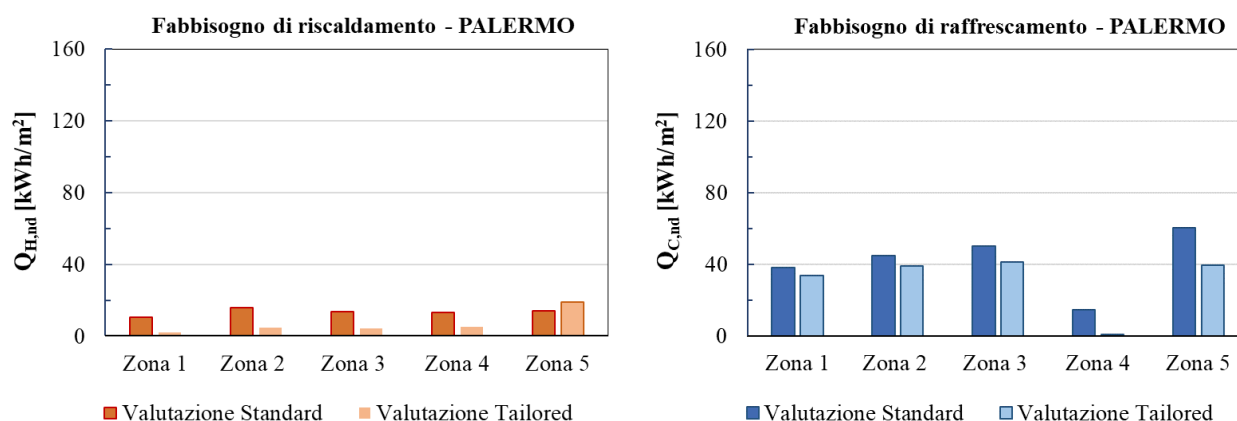
Figura 19. Fabbisogno di riscaldamento (sinistra) e raffrescamento (destra) relativo alle singole zone termiche e all'intero edificio – Palermo, UNI TS 11300.
