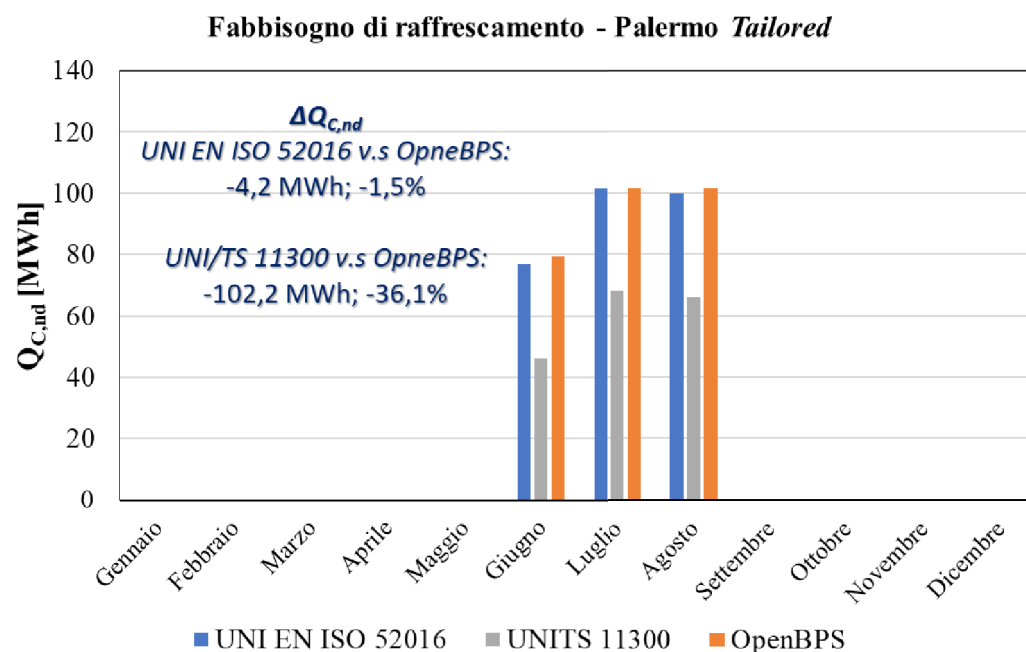
Figura 47. Fabbisogno di raffrescamento, UNI TS 11300, UNI EN ISO 52016, OpenBPS (V1) – valutazione Tailored , Palermo.
