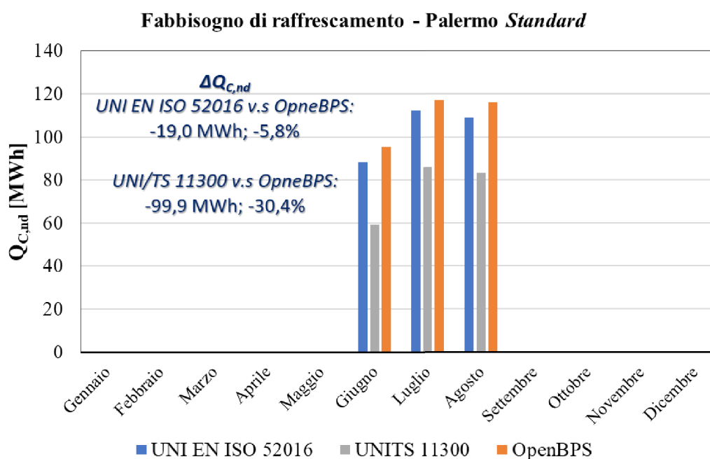
Figura 46. Fabbisogno di raffrescamento, UNI TS 11300, UNI EN ISO 52016, OpenBPS (V1) – valutazione Standard , Palermo.
