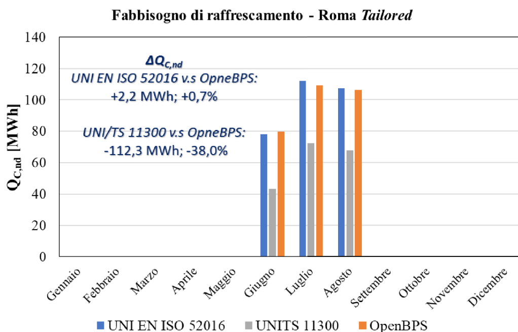
Figura 35. Fabbisogno di raffrescamento, UNI TS 11300, UNI EN ISO 52016, OpenBPS (V1) – valutazione Tailored, Roma
