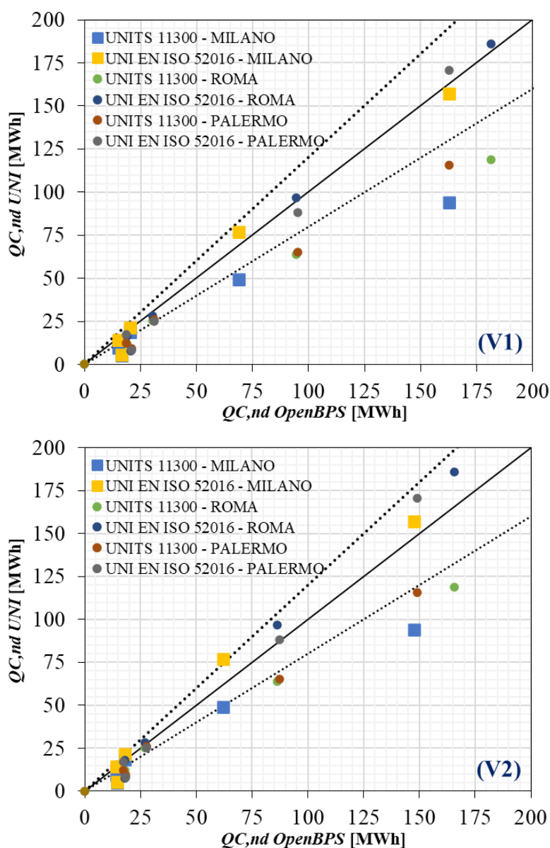
Figura 60. Fabbisogni di energia termica utile per il raffreddamento Q_{C,nd} : risultati delle norme UNI (TS 11300 e EN ISO 52016) verso quelli di OpenBPS (V1 e V2) – valutazione Standard.
