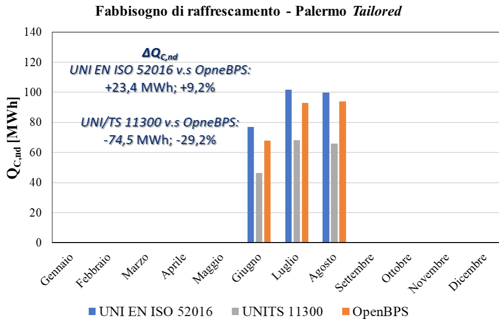
Figura 51. Fabbisogno di raffreddamento, UNI TS 11300, UNI EN ISO 52016, OpenBPS (V2) – valutazione Tailored , Palermo.
