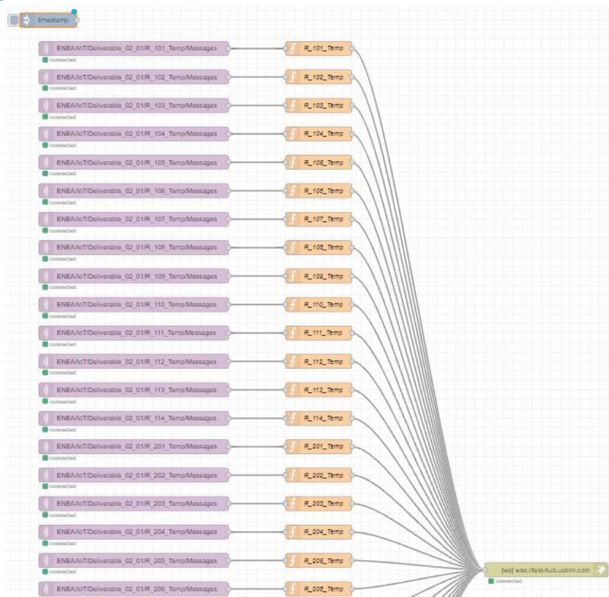
Figura 22. Brano del flow implementato in Node-RED.
