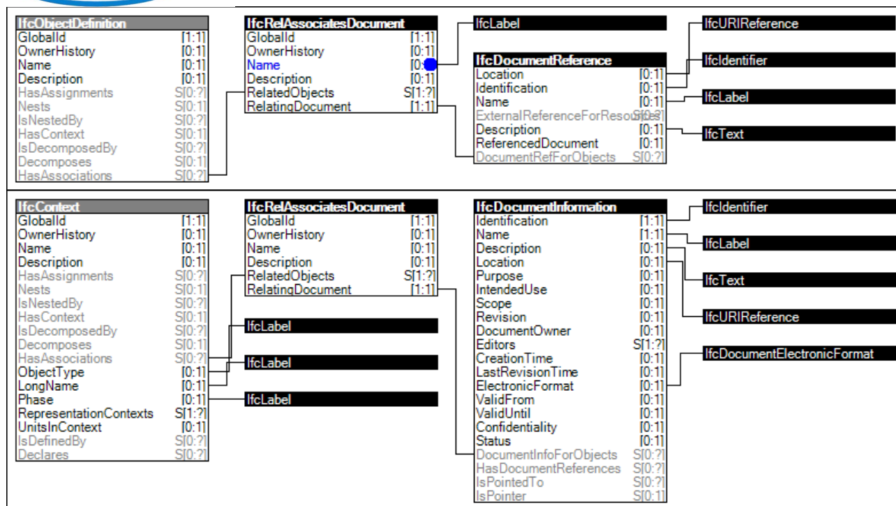
Figura 4. Assegnazione di un riferimento di documento ad un oggetto (in alto) o al progetto (in basso) in IFC.
