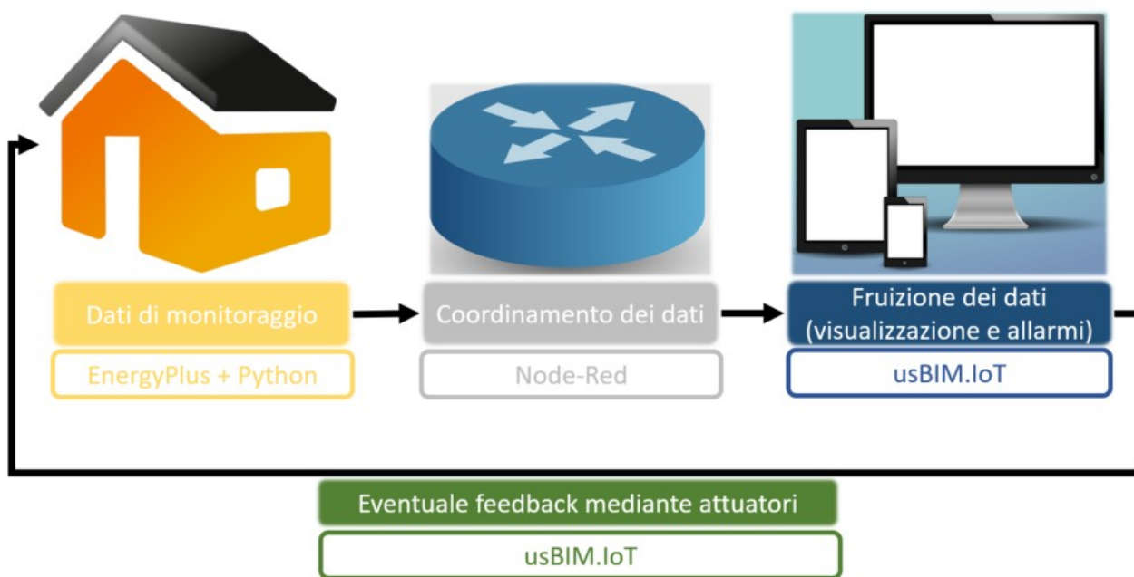
Figura 18. Workflow dell'esperienza di coordinamento e fruizione di dati di monitoraggio attraverso piattaforma BIM aperta.
