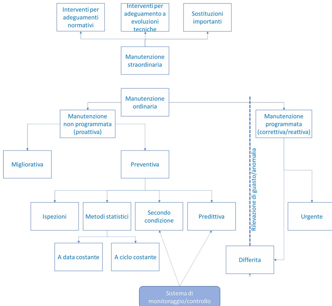
Figura 1. Principali tipi di manutenzione.
