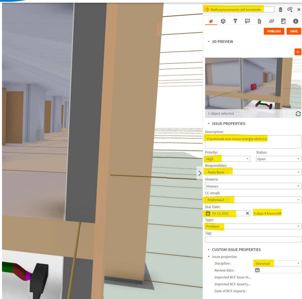
Figura 6. Inserimento di una richiesta di intervento di manutenzione secondo standard BCF.
