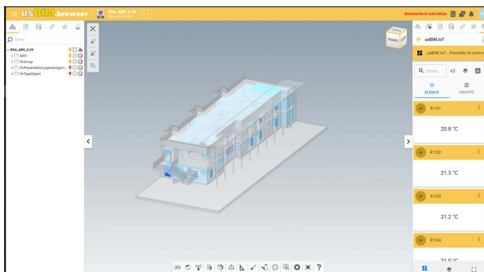
Figura 20. Esempio di visualizzazione dei correnti valori dei parametri monitorati, su modello tridimensionale e tile, in usBIM IoT.
