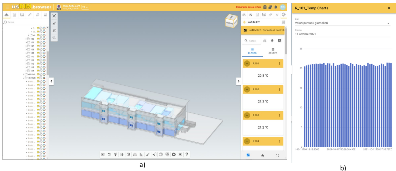
Figura 33. Esempio di visualizzazione dei dati rilevati mediante cromia su modello tridimensionale (a, sezione centrale), tile (a, sezione destra) e grafico (b).
