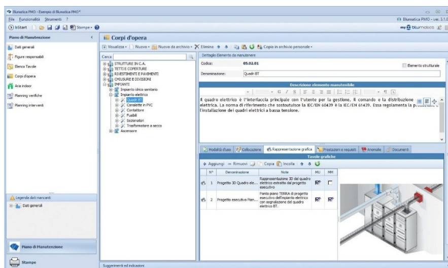
Figura 12. Inserimento degli elementi da mantenere in Blumatica PMO.
