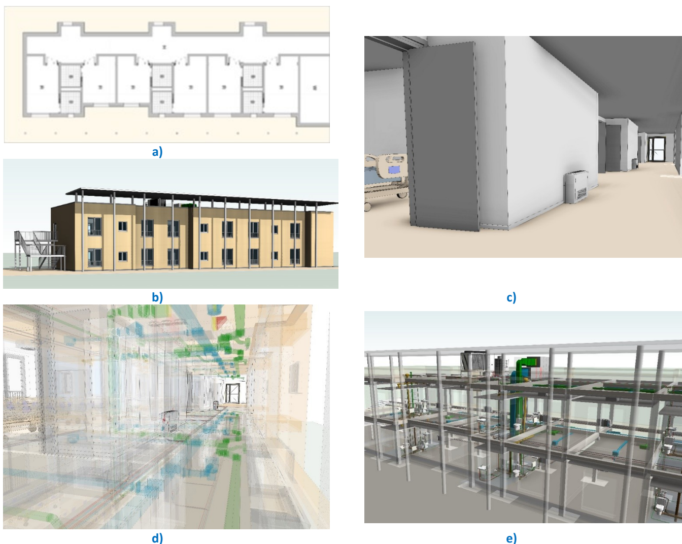
Figura 45. L'edificio oggetto dell'esperienza di comparazione tra progettazione convenzionale e progettazione BIM: pianta del piano tipo (a), vista esterna (b), vista interna (c), vista interna tramite trasparenze (d) e vista esterna con modello architettonico in trasparenza (e).
