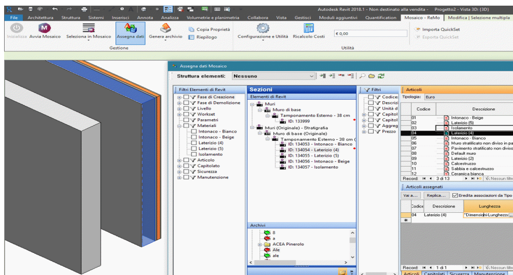
Figura 11. ReMo: esempio di applicazione degli interventi manutentivi a elementi del modello.
