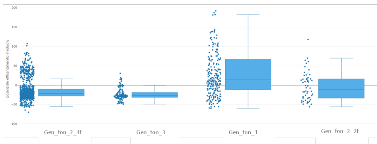
Figura 3.28 - Potenziale teorico di efficientamento estivo dell'involucro delle tipologie della Fondazione.
