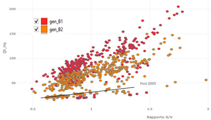
Figura 3.17 - Relazione tra fabbisogno netto riscaldamento e S/V per le tipologie isolate (villettes) gen_B1 e gen_B2.
