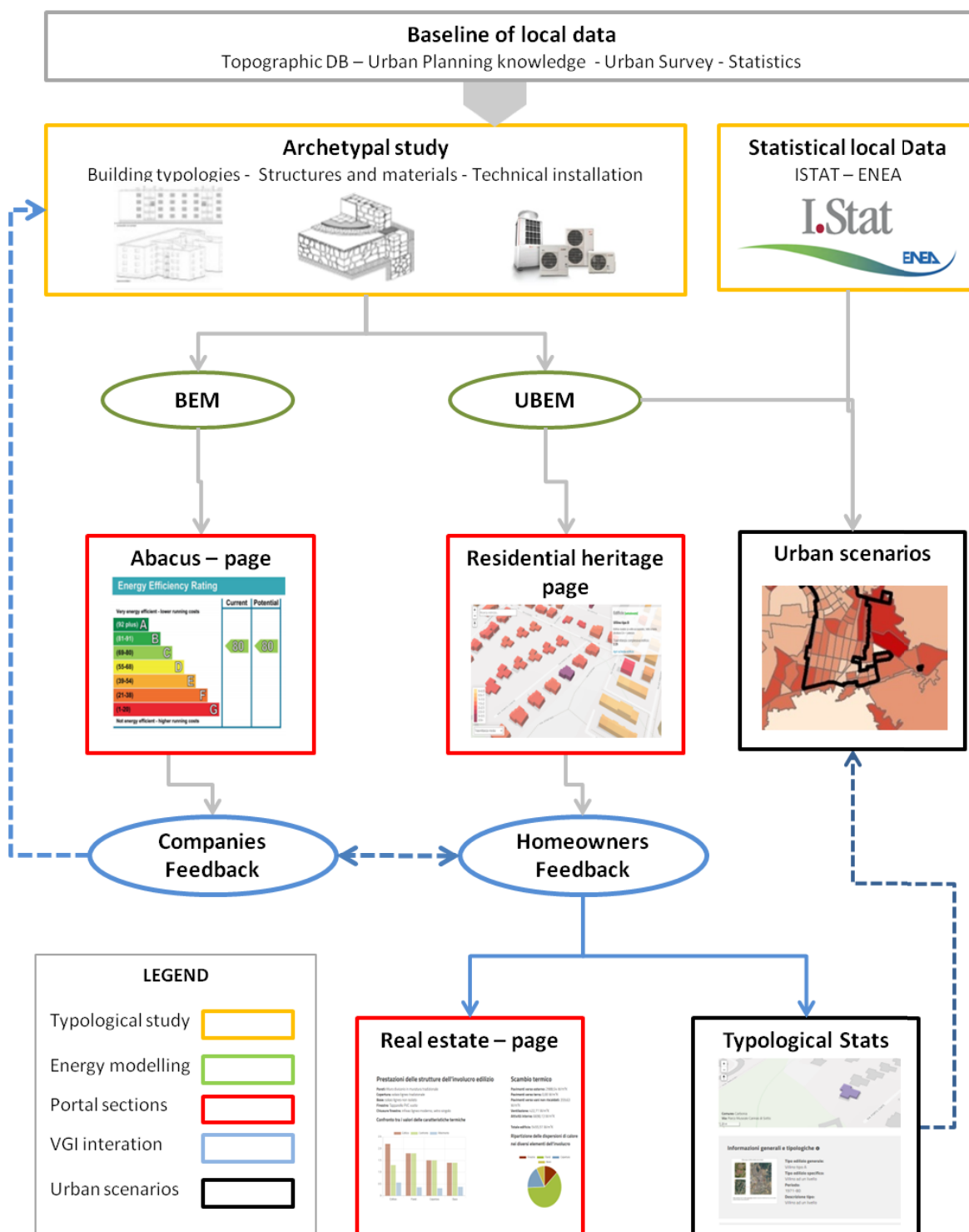
Figura 2.5 - Diagramma generale delle interazioni tra UBE M e sezioni del portale.
