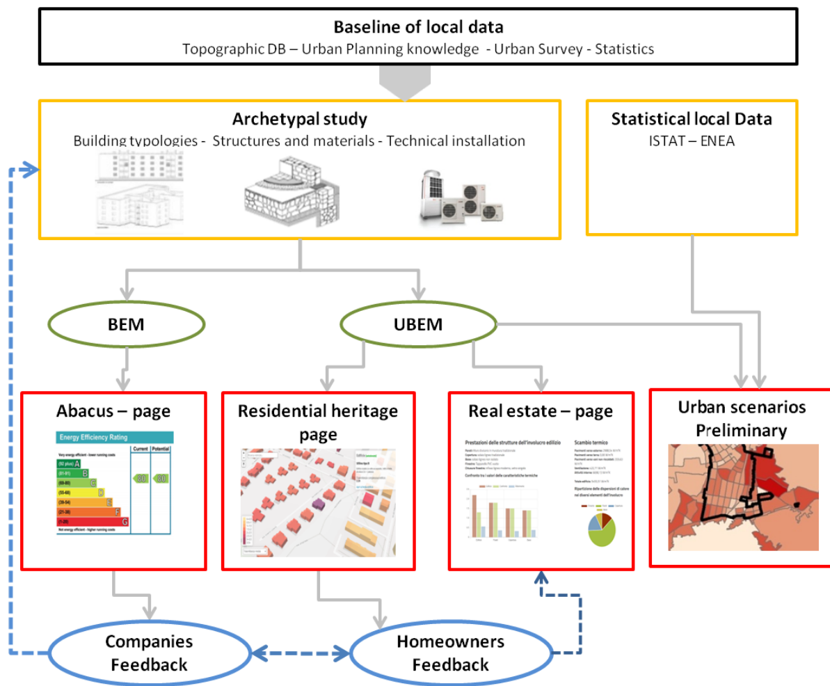
Figura 1. Schema di UBEU sviluppato nel progetto.
