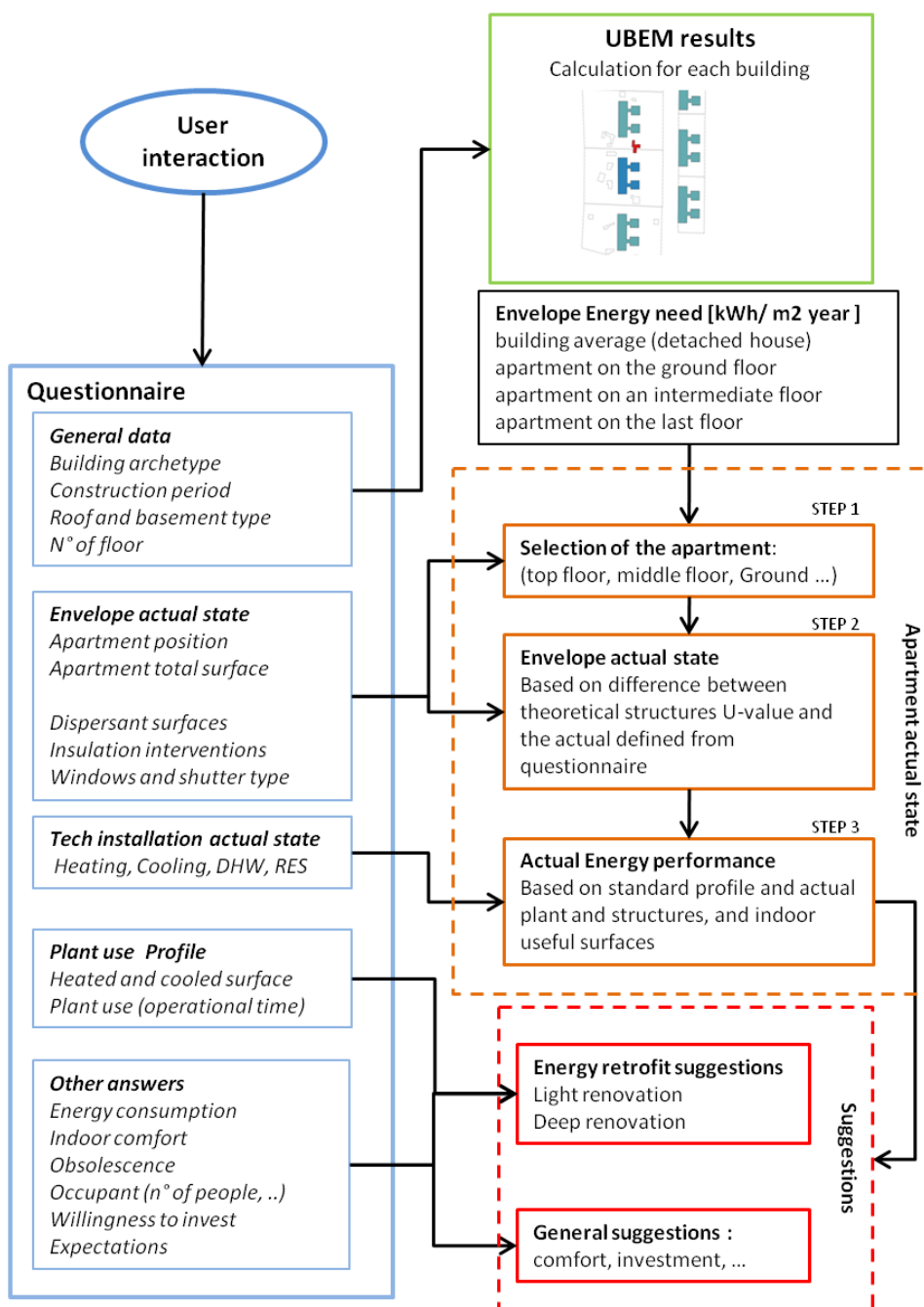
Figura 4. Diagramma della scheda unità immobiliare.
