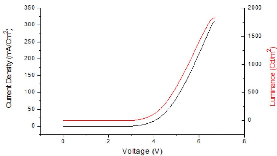
Figura 4: Caratteristiche I-V, EL-V di un OLED luminescente nel bianco
