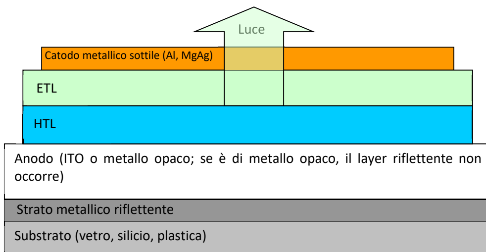
Figura 2: struttura non invertita per l'OLED top-emitting.
