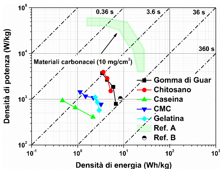
Figura 31. Diagramma di Ragone della potenza specifica rispetto all'energia specifica per gli elettrodi studiati rispetto ad altri SC simmetrici a base di carbonio ecosostenibili con elettrolita acquoso. I riferimenti bibliografici [A] e [B] corrispondono rispettivamente a [27] e [28].
