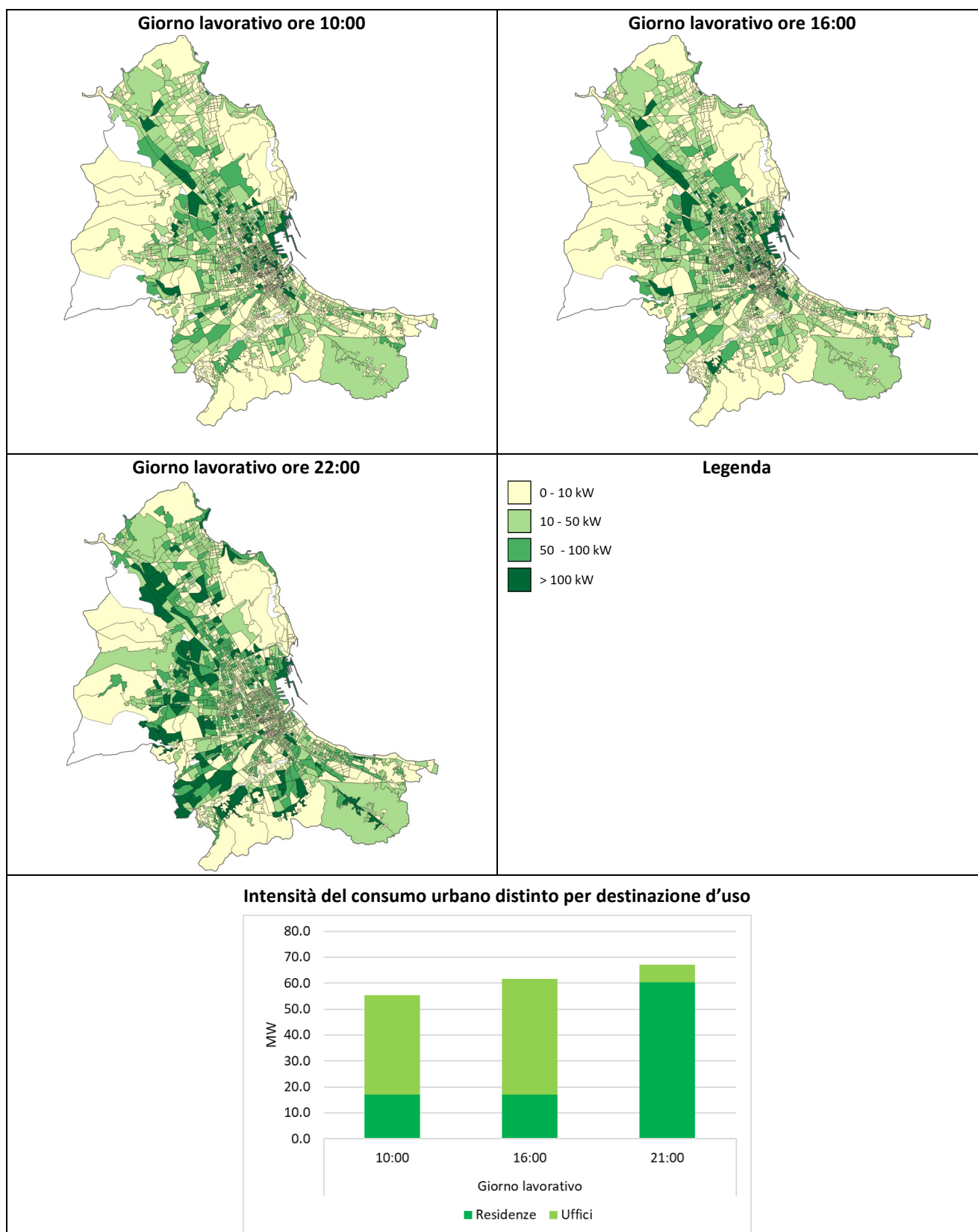
Figura 21. Intensità del consumo di elettricità per apparecchiature ed illuminazione artificiale in un giorno lavorativo dell'anno.
