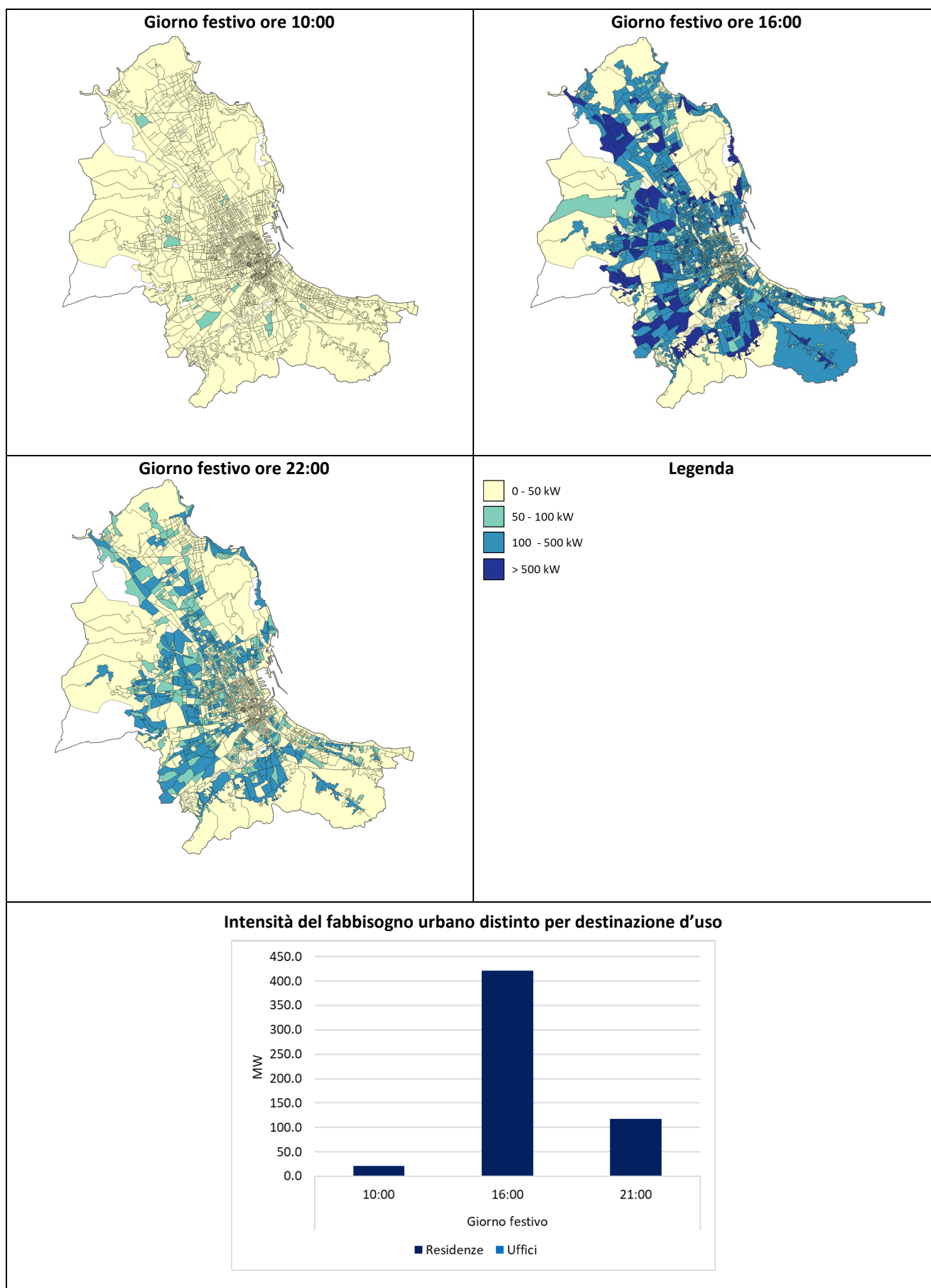
Figura 20. Intensità del fabbisogno termico per raffrescamento in un giorno festivo di luglio.
