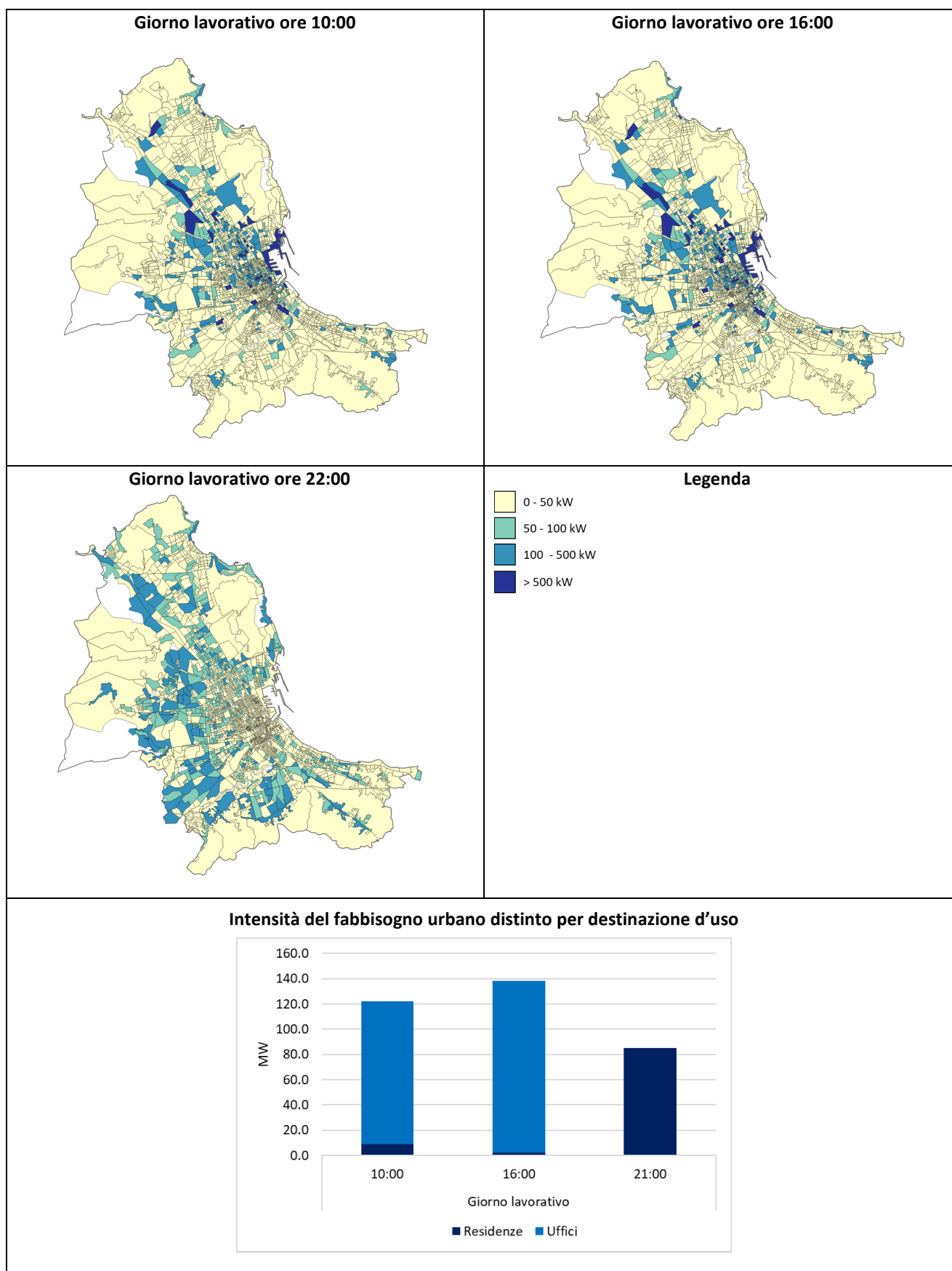
Figura 19. Intensità del fabbisogno termico per raffrescamento in un giorno lavorativo di luglio.
