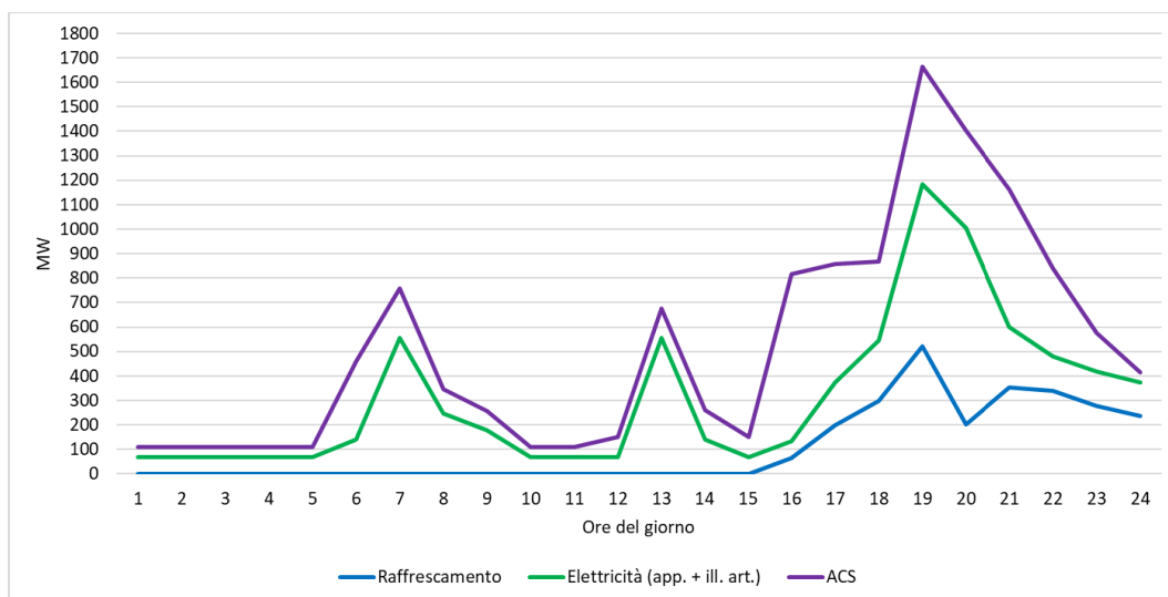
Figura 33. Selezione di un'area urbana (sopra) e determinazione del relativo profilo orario dei consumi di elettricità, in un giorno lavorativo estivo, per raffrescamento, ACS, apparecchiature ed illuminazione (sotto).
