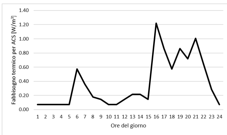
Figura 32. Profilo di densità di fabbisogno termico per ACS per un giorno tipo.
