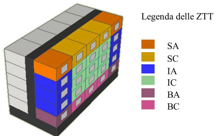
Figura 2. Modello tridimensionale del Building Energy Concept e delle Zone Termiche Tipo.
