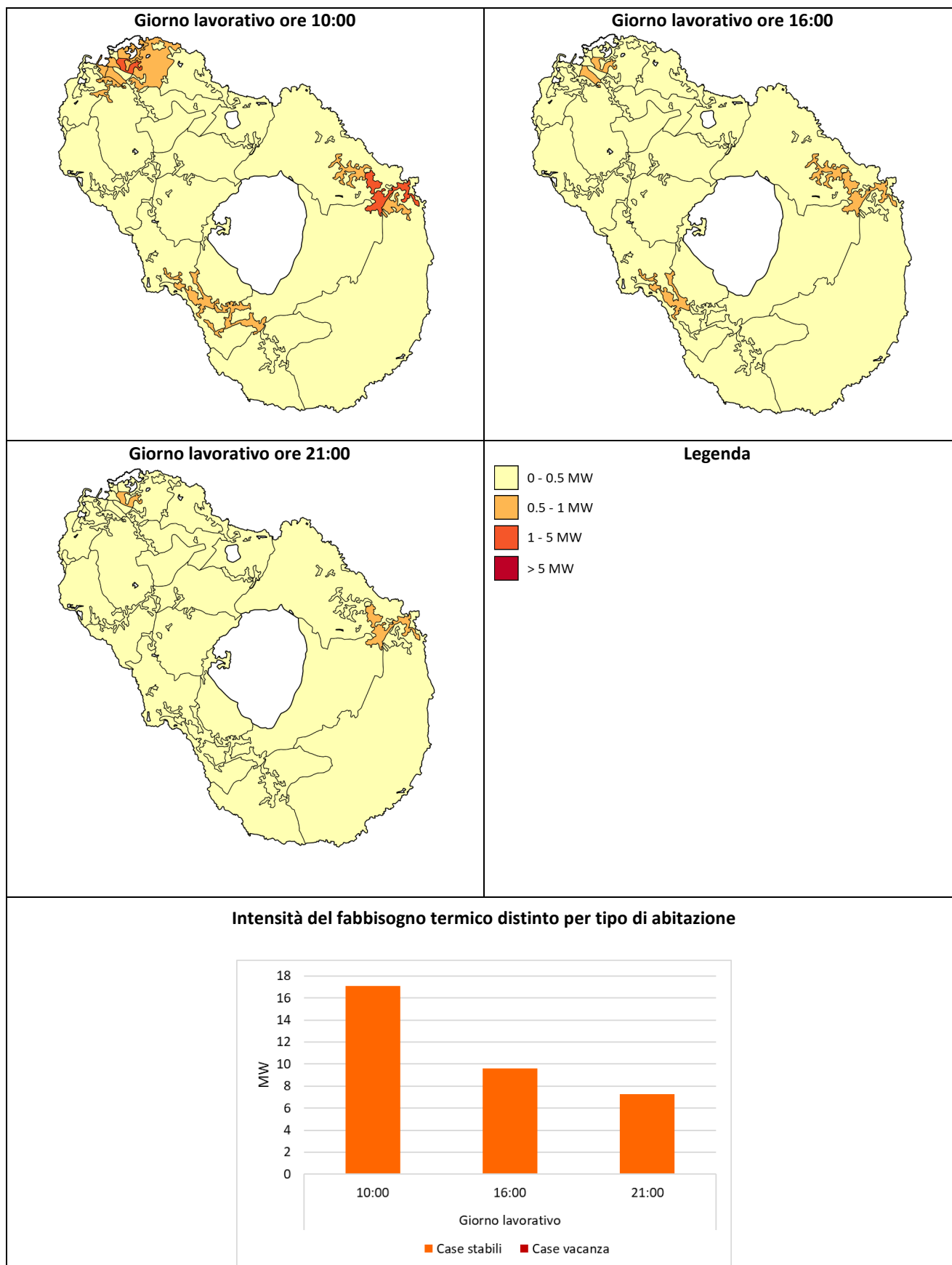
Figura 34. Intensità del fabbisogno termico per riscaldamento in un giorno lavorativo di gennaio.
