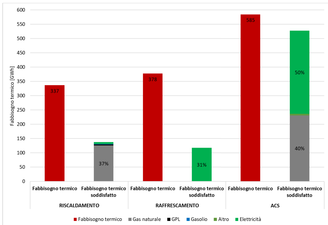
Figura 58. Fabbisogni termici del volume costruito ad uso residenziale ripartiti per fonte energetica.
