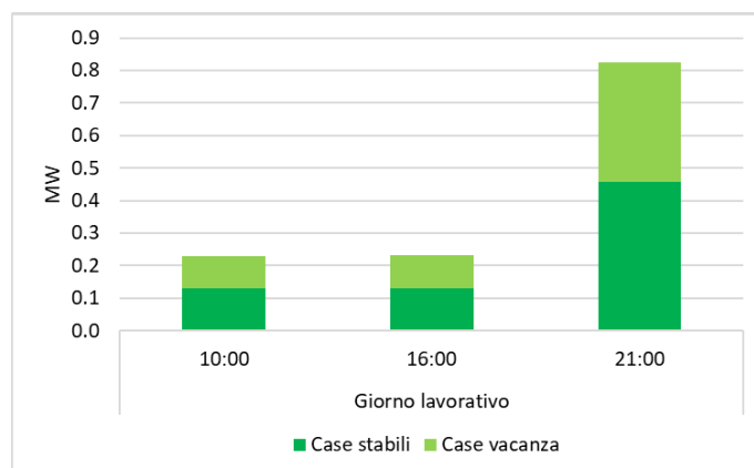
Intensità del consumo di elettricità distinto per tipo di abitazione
