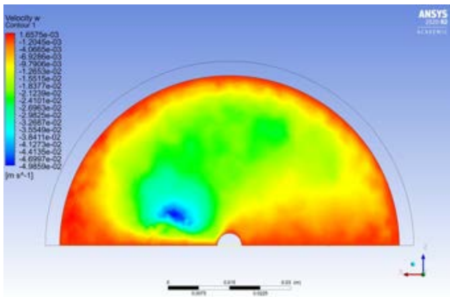
Figura 42-Piano di uscita H2O – Velocità lungo z
