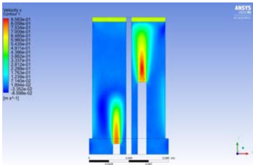
Figura 30-Piano di simmetria – Velocità lungo y del miscuglio gassoso
