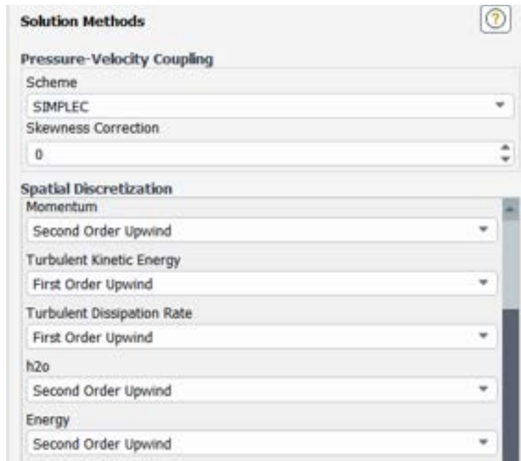
Figura 23-Discretizzazione spaziale
