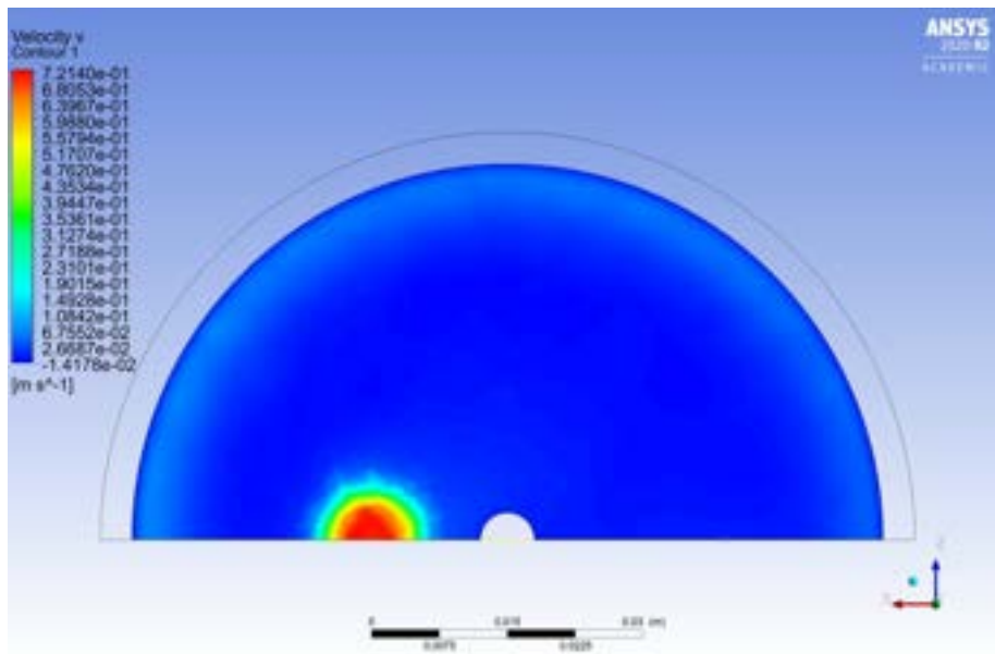
Figura 41-Piano di uscita H2O – Velocità lungo y
