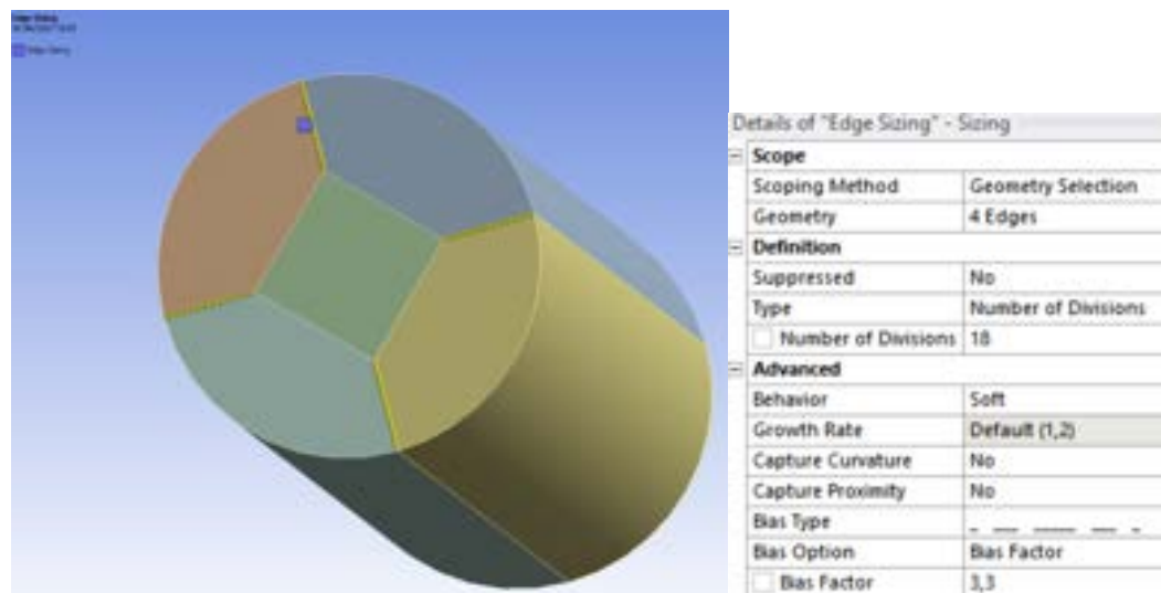
Figura 52-Dimensionamento localizzato radiale
