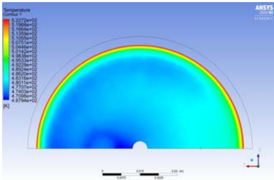
Figura 39-Piano di uscita H2O - Temperatura
