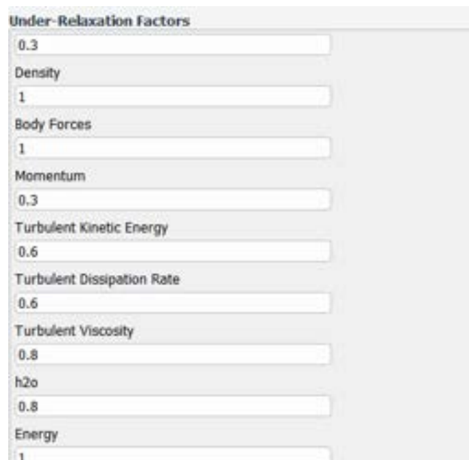
Figura 24-Fattori di sottorilassamento
