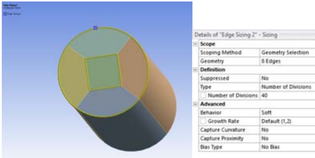
Figura 51-Dimensionamento localizzato circonferenziale
