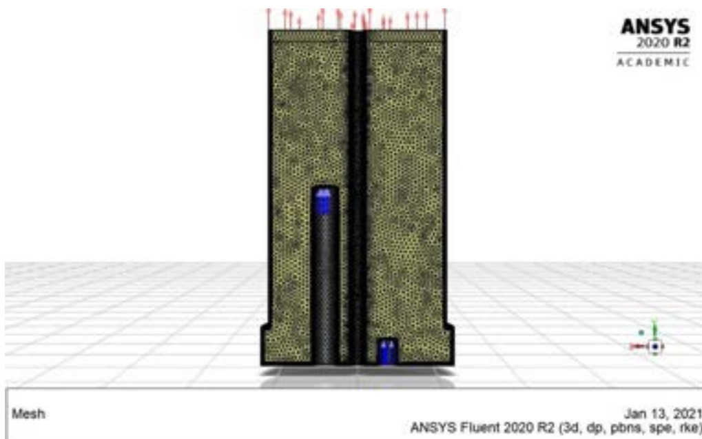
Figura 20-Mesh tetraedrica
