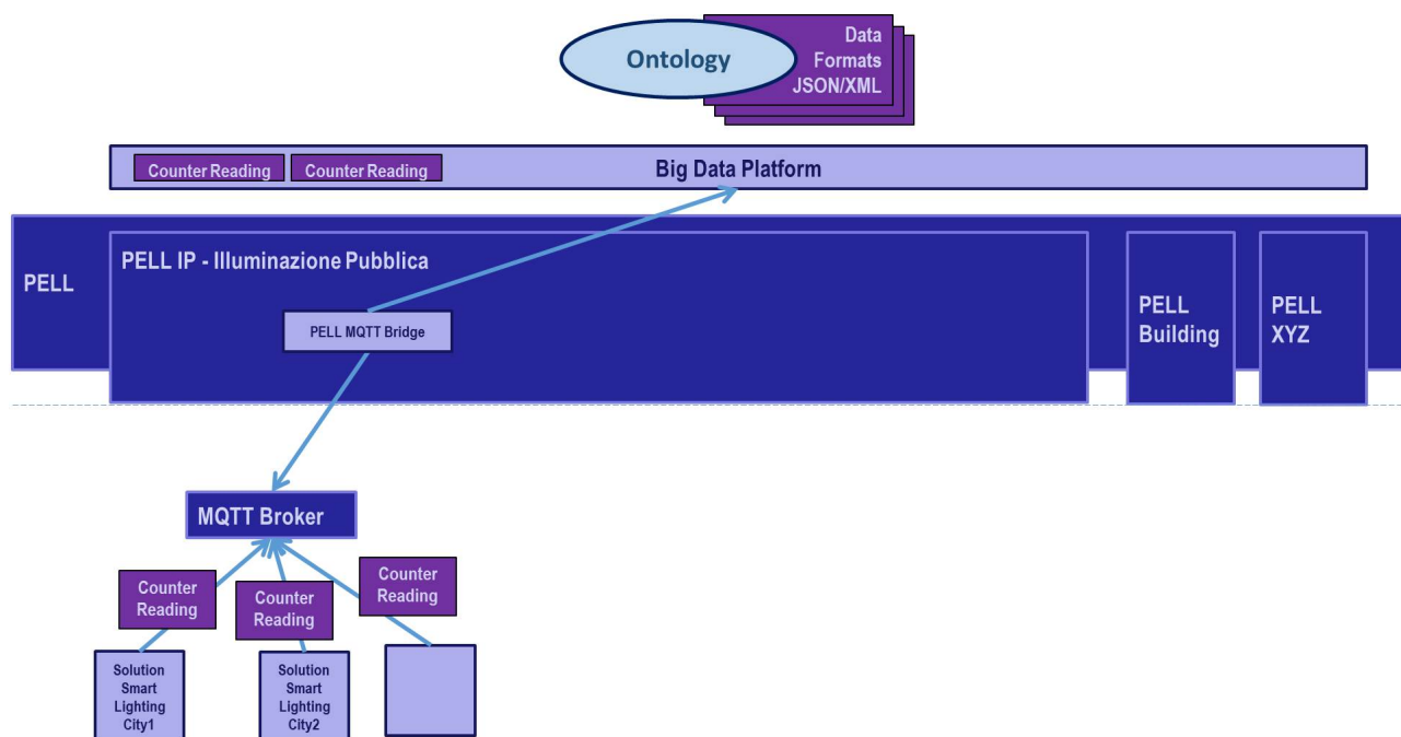
Figura 5. Architettura schematica PELL
