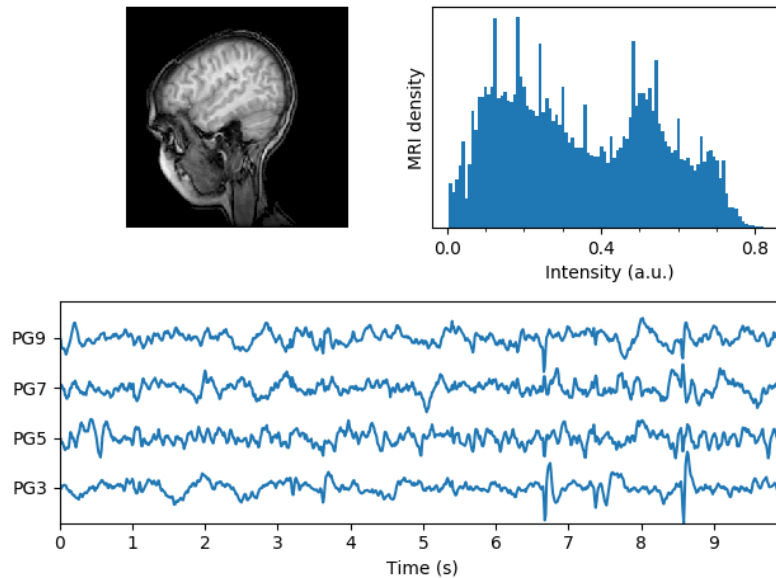
Figura 21. Matplotlib - Esempi
