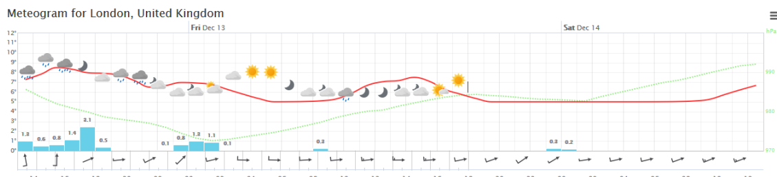
Figura 17. Highcharts – Esempio
