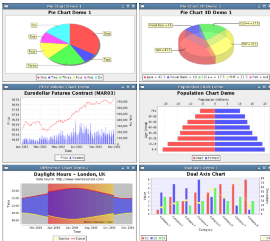
Figura 24. JfreeChart - Esempi
