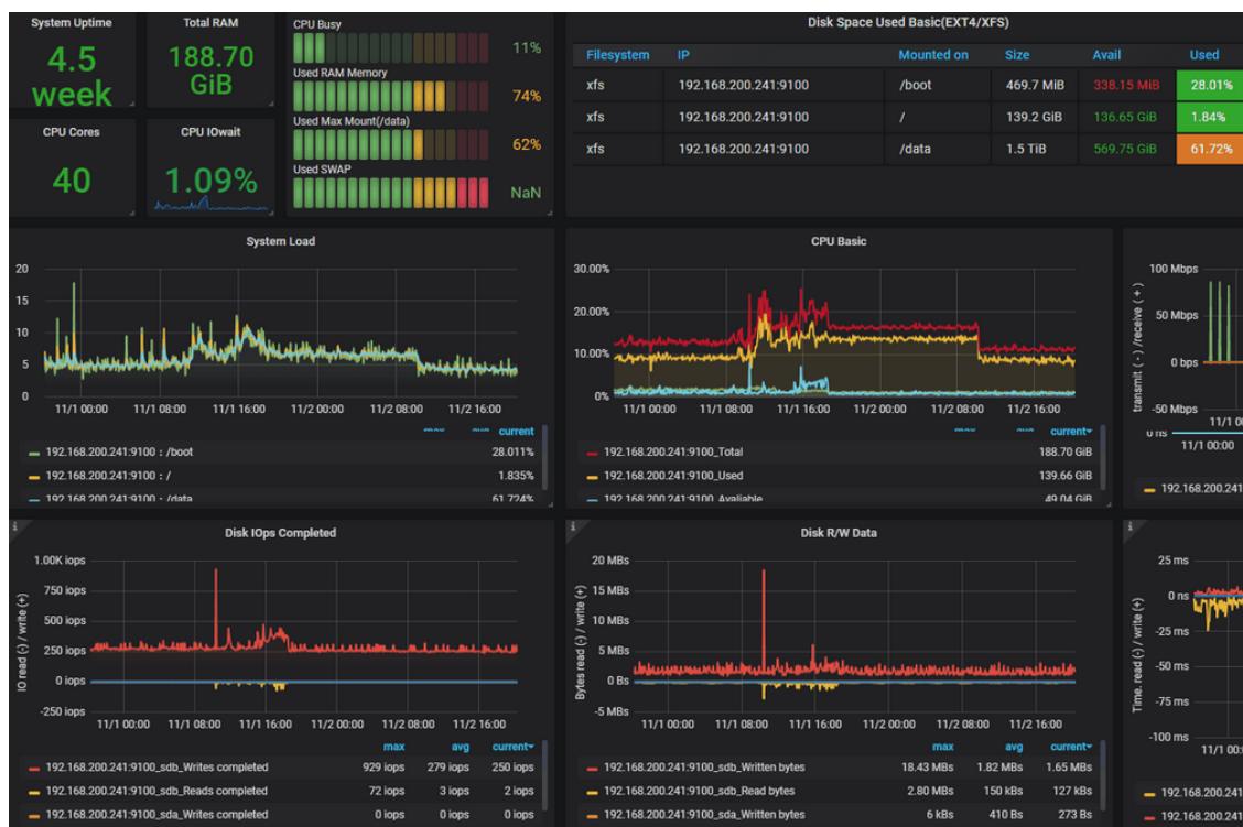
Figura 23. Grafana - Esempio di dashboard
