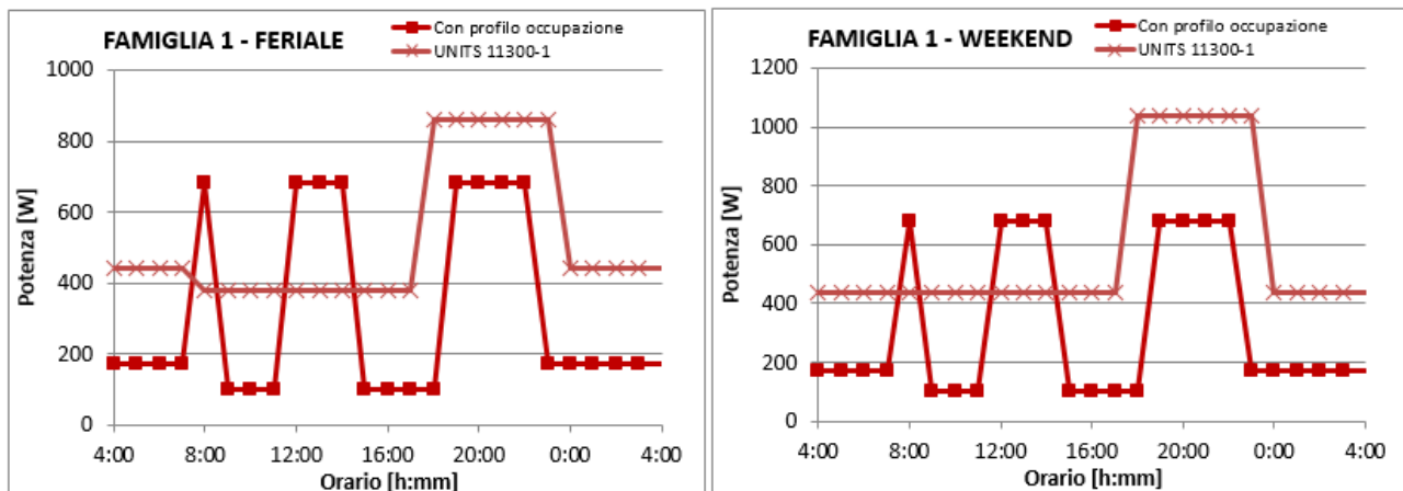
Figura 15 – Profili orari medi di potenza da apporti interni per la famiglia di 1 componente
