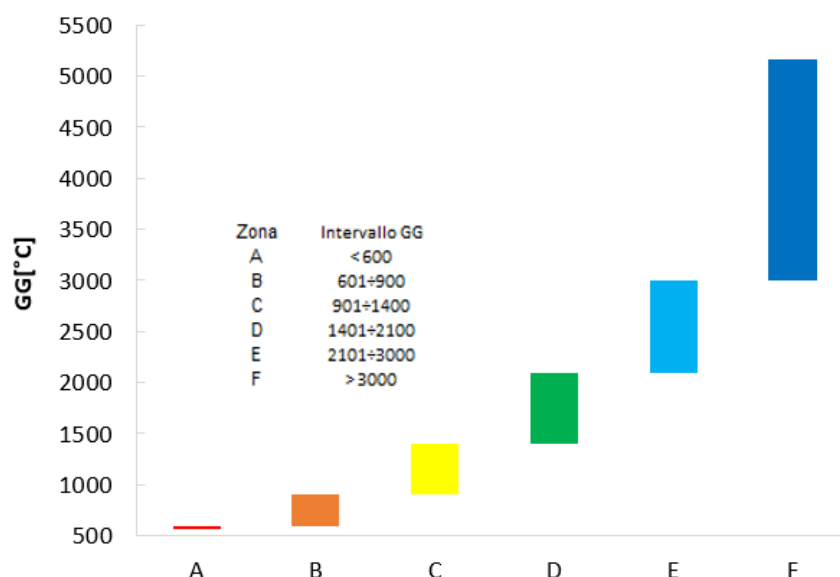
Figura 2 – Definizione delle zone climatiche italiane in base ai gradi-giorno
