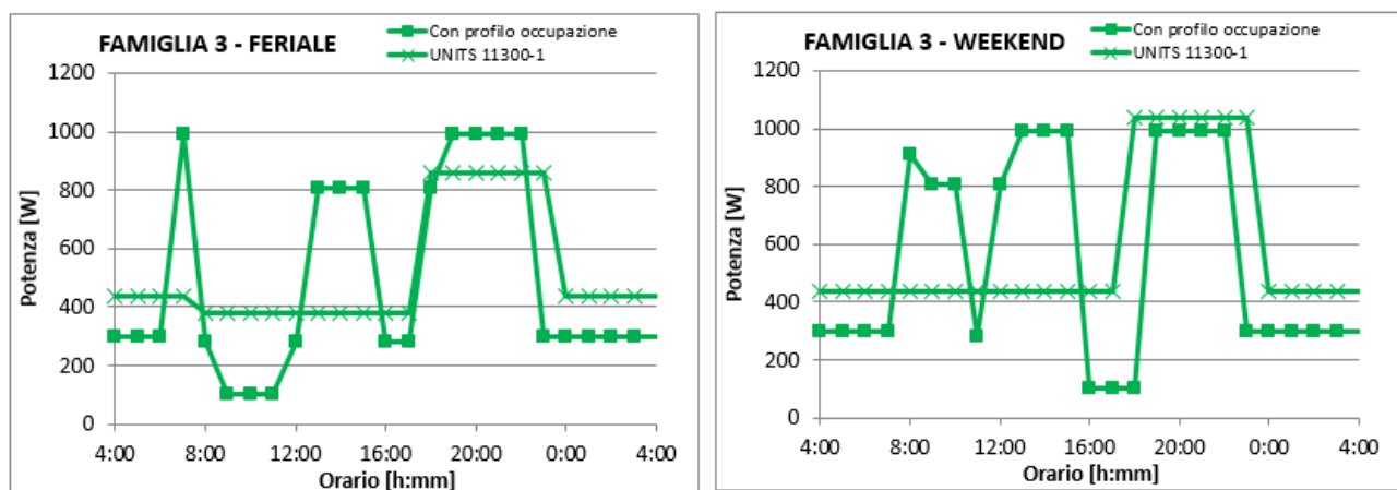
Figura 17 – Profili orari medi di potenza da apporti interni per la famiglia di 3 componenti
