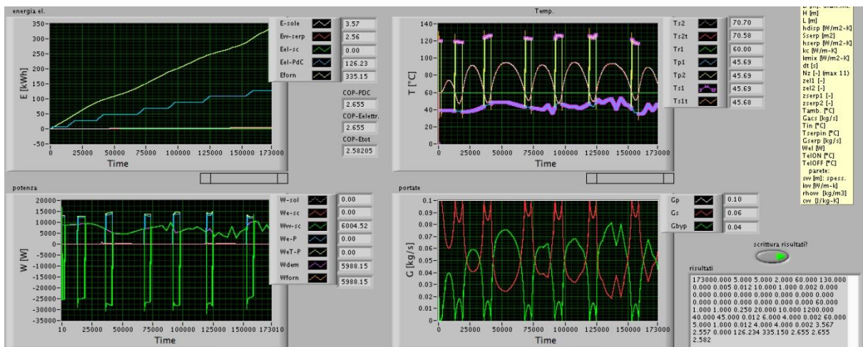
Figura 66 – Esempio di pannello frontale e risultati dopo una simulazione di circa 48 ore per lo schema n.2 (in alto con accumulo a PCM, in basso i soli grafici del caso senza accumulo a PCM)
