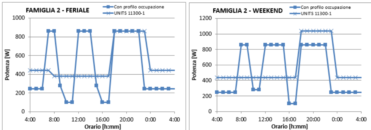
Figura 16 – Profili orari medi di potenza da apporti interni per la famiglia di 2 componenti
