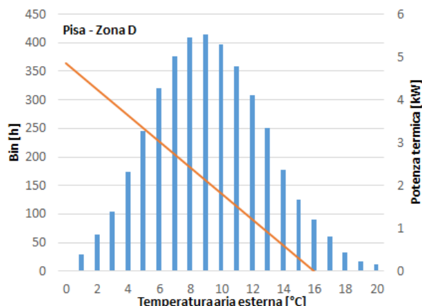
Figura 10b – Calcolo della potenza di progetto. Pisa (zona D)
