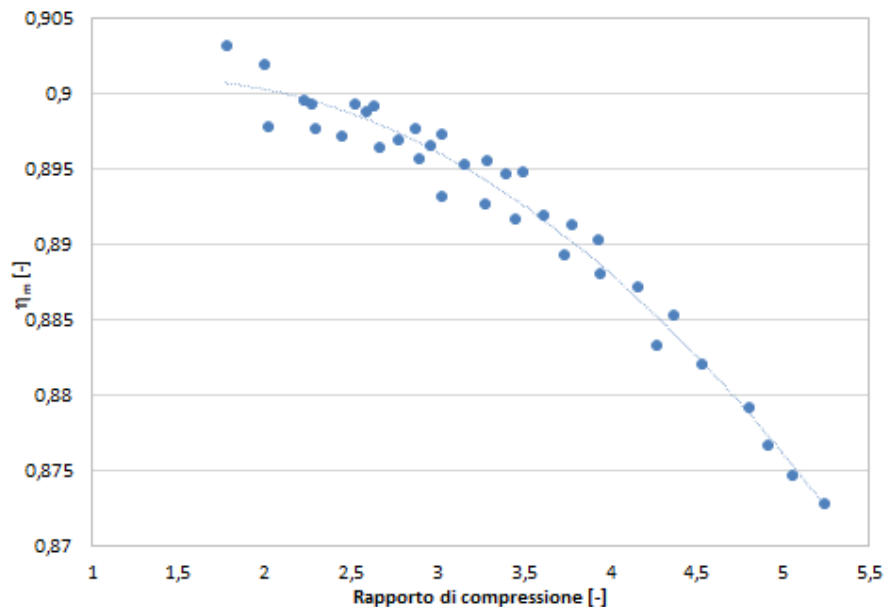
Figura 60 – Rendimento del motore per il compressore Dorin CD-1300 H
