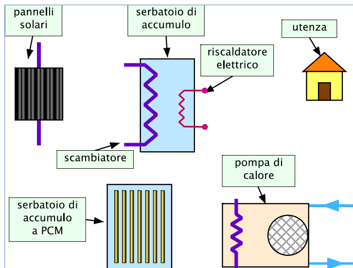
Figura 50 – componenti simulati
