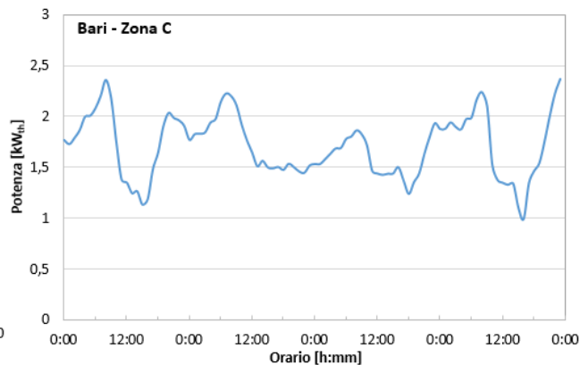
Figura 25 – Profilo di potenza termica per l'abitazione in zona C
