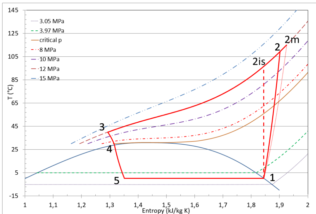
Figura 58 - Diagramma T-s di un ciclo inverso transcrito a CO 2
