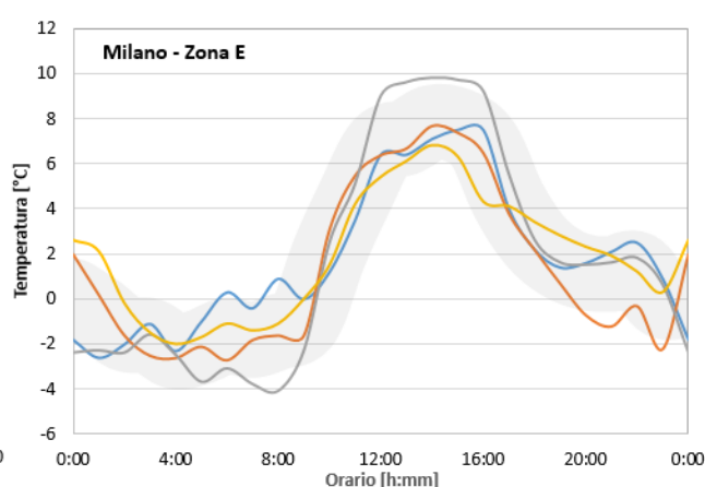
Figura 22 – Profilo giornaliero di riferimento della temperatura dell'aria esterna - zona E
