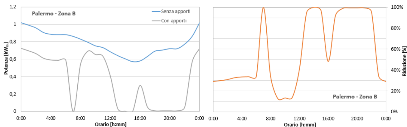
Figura 29 – Influenza dell'occupazione sul profilo giornaliero di potenza termica per l'abitazione in zona B
