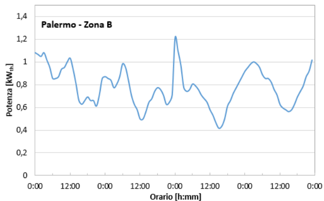
Figura 24 – Profilo di potenza termica per l'abitazione in zona B
