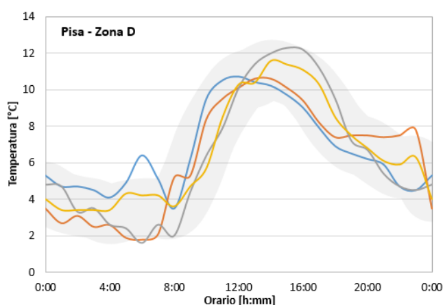
Figura 21 – Profilo giornaliero di riferimento della temperatura dell'aria esterna - zona D
