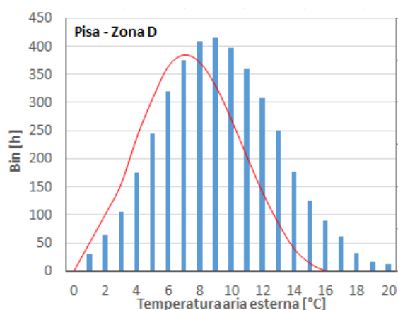
Figura 10a – Fabbisogno energetico in funzione della temperatura esterna. Pisa (zona D)
