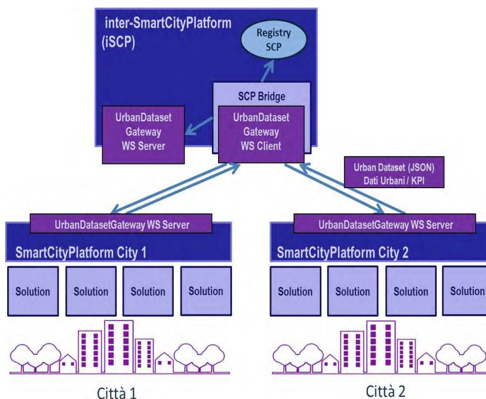
Figura 4 - SCP-Bridge per abilitare comunicazione tra iSCP e SCP (ripresa da LA 1.19)
