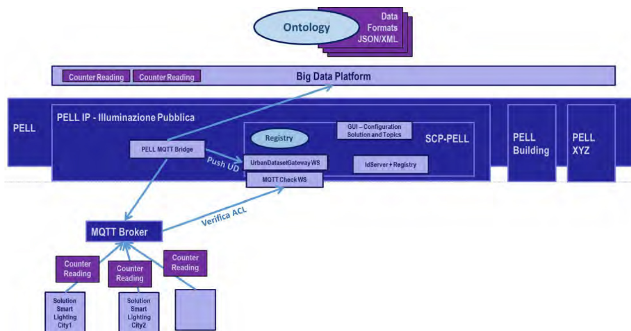
Figura 25 - Architettura PELL IP integrato con SCP-PELL
