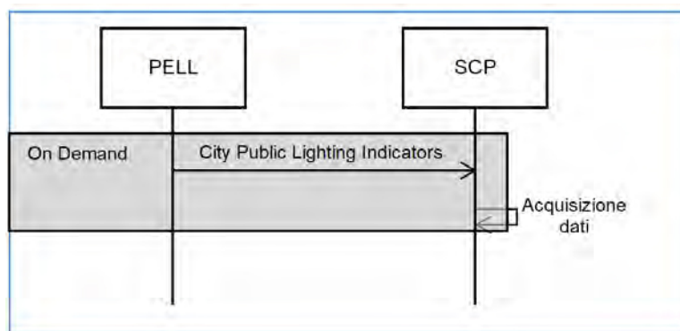
Figura 18 - Diagramma di sequenza UML del caso studio Smart Lighting "PELL" - invio indicatori urbani
