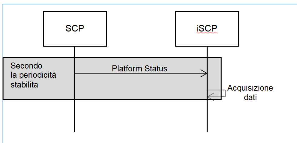
Figura 16 - Diagramma di sequenza UML del caso studio "iSCP"
