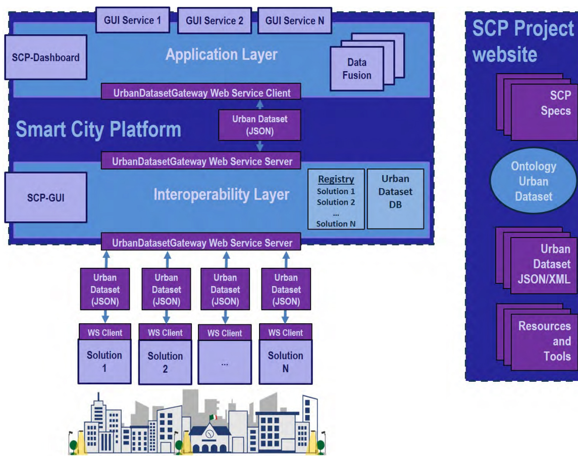
Figura 15 - Architettura di Riferimento SCP
