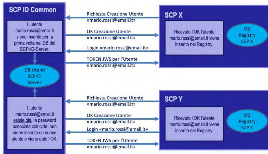
Figura 31 - SCP-ID-Common, illustrazione criticità
