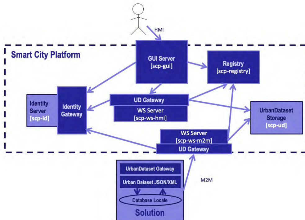
Figura 29 - Architettura Software SCP-Casaccia.
