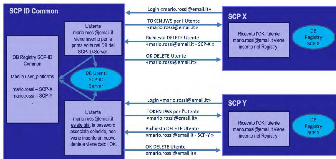
Figura 32 - SCP-ID-Common, risoluzione criticità
