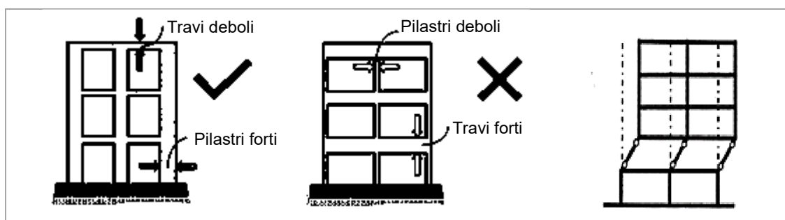
Figura 53. Esempi di gerarchia di resistenza: presenza (pilastrì forti e travi deboli); e assenza (travi forti, pilastrì deboli) che può causare meccanismi di piano soffice in caso di sisma
