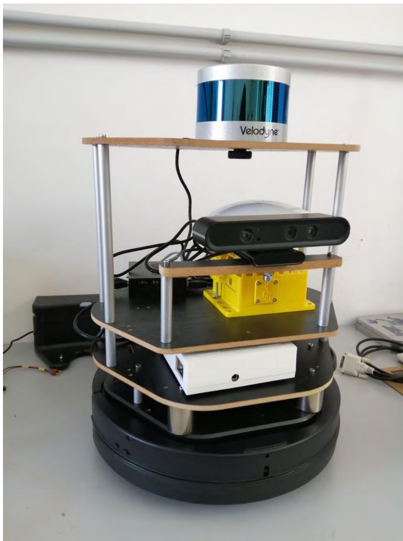
Figura 11. La piattaforma Turtlebot-2 utilizzata in questa fase di sperimentazione in ambiente reale, a cui sono stati aggiunti i sensori LIDAR e GPS-RTK
