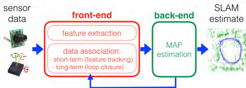
Figura 1. Generica architettura di SLAM
