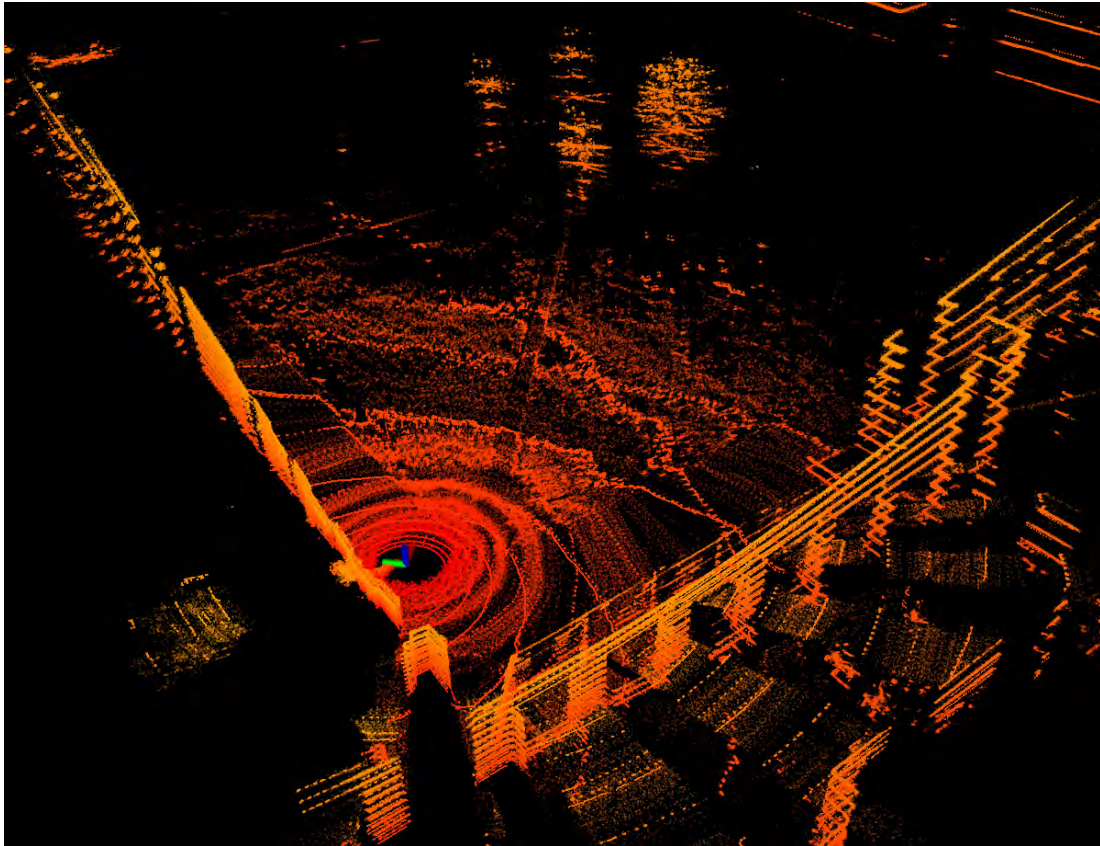
Figura 13. Mappa e posa del robot stimata con il LIO-SAM
