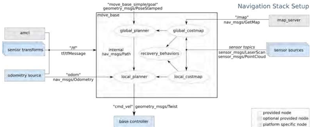
Figura 3. Architettura dello stack di navigazione
