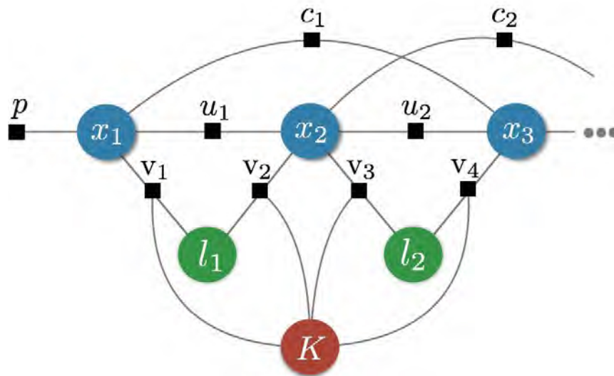
Figura 2. Esempio di rappresentazione a grafo per un problema di SLAM: i nodi blu ( x_1, x_2, x_3 ) rappresentano le pose del robot in istanti successivi, l'arco p rappresenta la dipendenza delle pose del robot con le pose precedenti non rappresentate dal grafo. I nodi in verde ( l_1, l_2 ) rappresentano le posizioni dei landmark, ossia i punti dell'ambiente facilmente riconoscibili (possono essere angoli, spigoli, zone ad alto contrasto visivo, ecc...). gli archi ( u_1, u_2 ) rappresentano i vincoli odometrici e cinematici del robot in posizioni successive. Gli archi ( c_1, c_2 ) rappresentano le chiusure di loop, ossia il fatto che il robot sia tornato in istanti successivi negli stessi punti dell'ambiente esplorato. Gli archi ( v_1, v_2, v_3, v_4 ) rappresenta il fatto che i landmark vengano osservati in specifiche posizioni del robot, infine il nodo in rosso K rappresenta l'insieme dei parametri del sensore o dell'algoritmo che si occupa dell'estrazione dei landmark.
