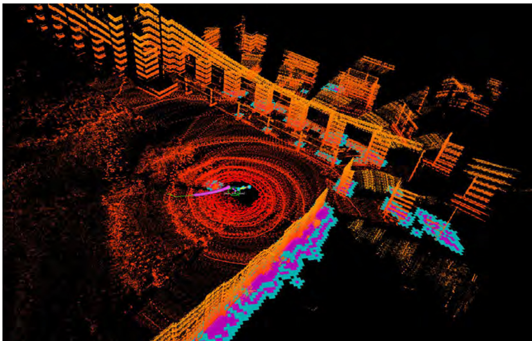
Figura 14. Mappa ottenuta con LIO-SAM, posa ottenuta tramite EKF e coastmap e traiettorie ottenute tramite TEB path planner
