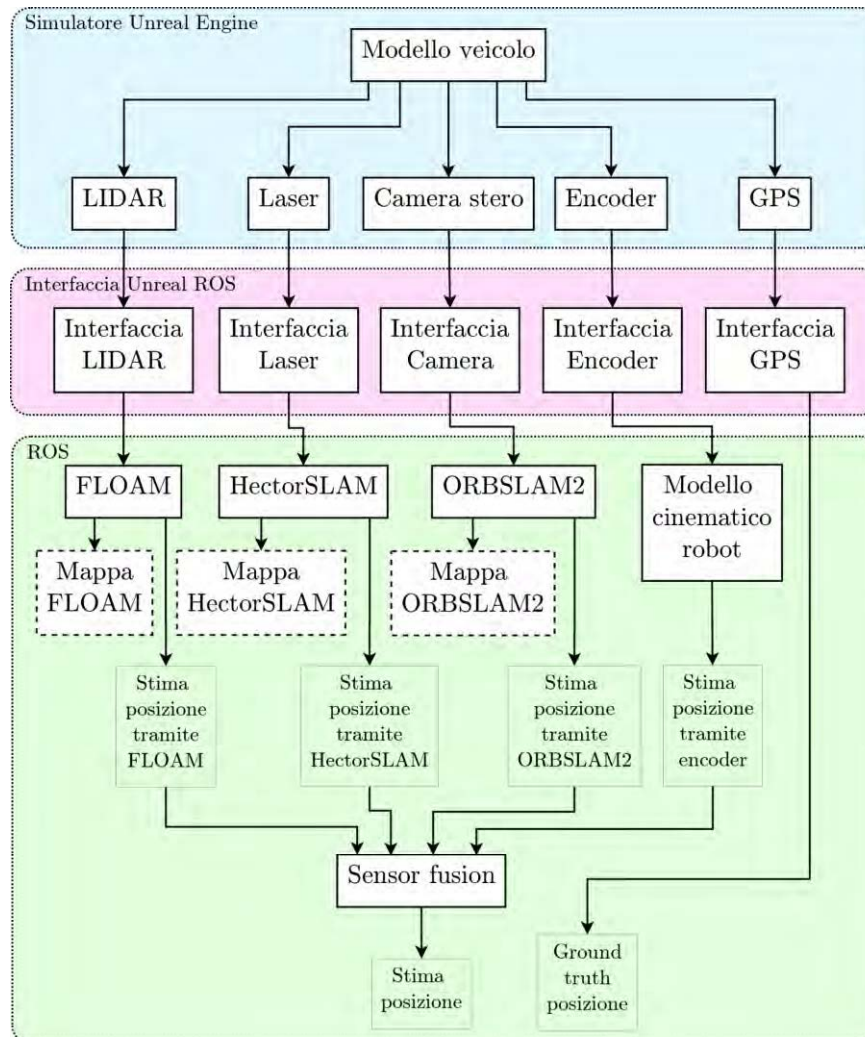
Figura 4. Schema a blocchi del sistema di navigazione implementato e dell'interfaccia verso il simulatore
