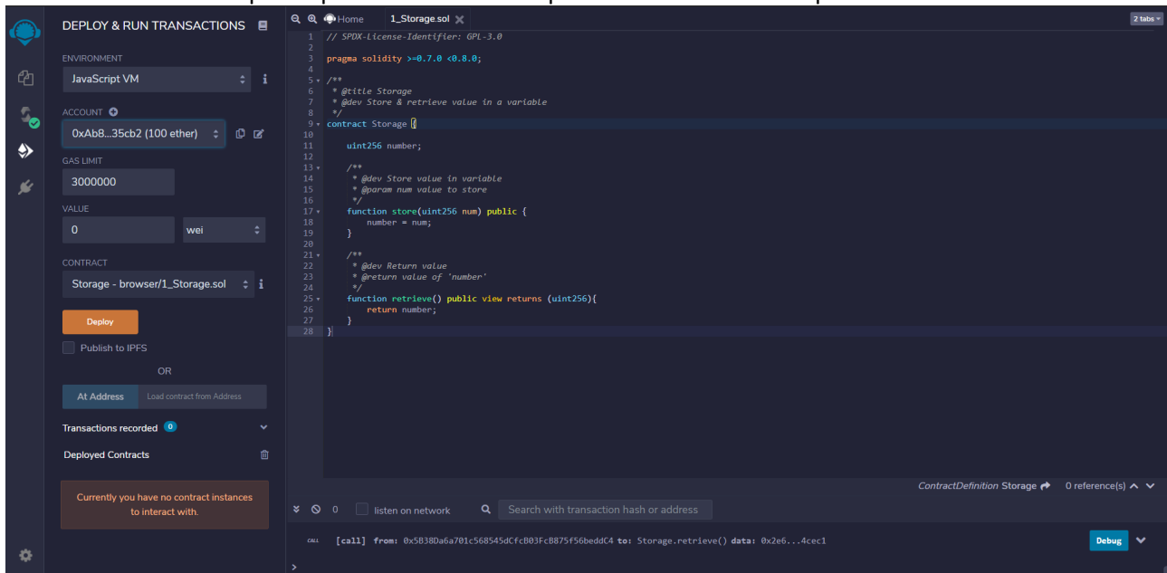
Figura 7. Deploy di un contratto.
