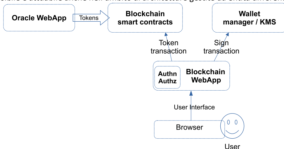
Figura 9 - Gestione Wallet lato infrastruttura con Webapp di gestione dell'accesso intermedia
