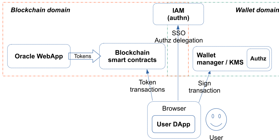
Figura 10 - Gestione Wallet lato infrastruttura con componenti disaccoppiati e DApp
