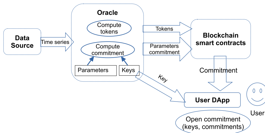
Figura 7 - Flusso dei dati con commitment confidenziale dei parametri di tokenizzazione
