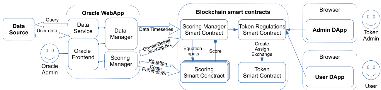
Figura 8 - Architettura di Alto Livello del sistema blockchain con oracolo e distributed applications
