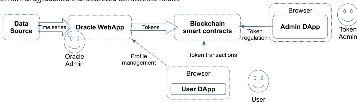
Figura 6 - Schema di alto livello dello scenario e della soluzione di riferimento
