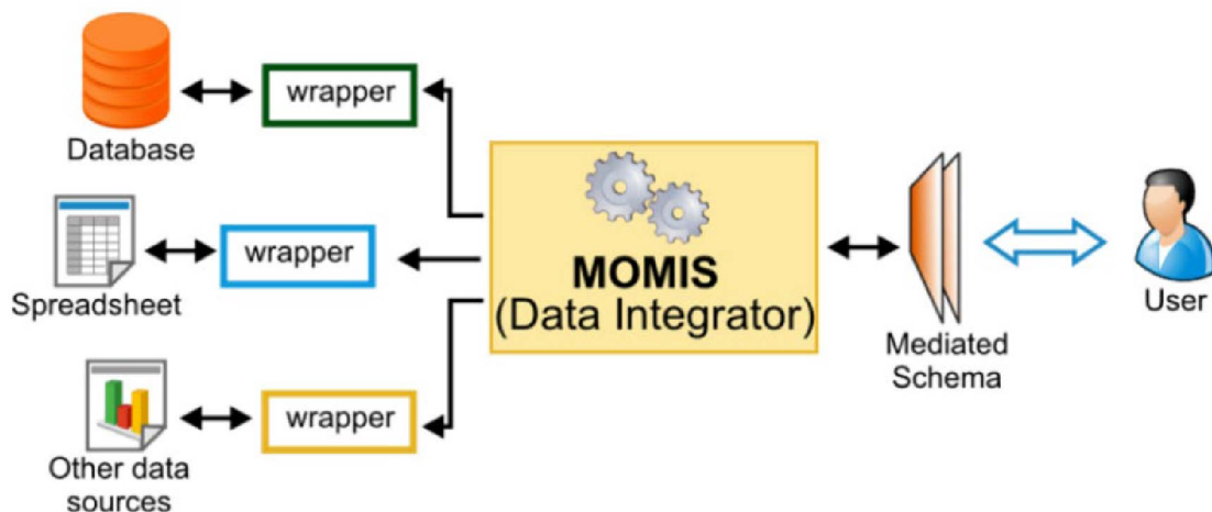
Figura 4 - Il sistema di Data Integration MOMIS
