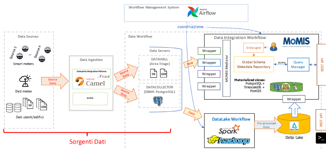
Figura 5 - Variante architettura: Delta Lake come generica sorgente del Data Integration
