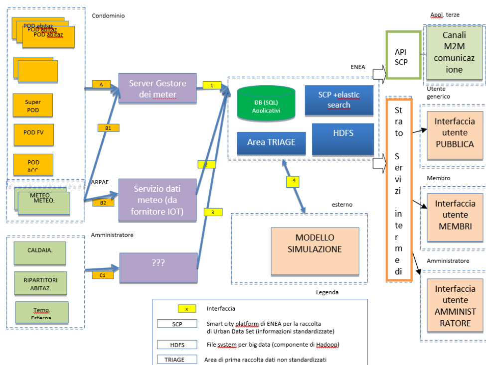
Figura 1 - SelfUser Use case: Architettura generale
