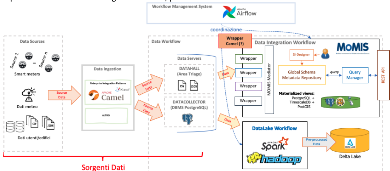
Figura 3 Overview dell'architettura – PRIMA VERSIONE
