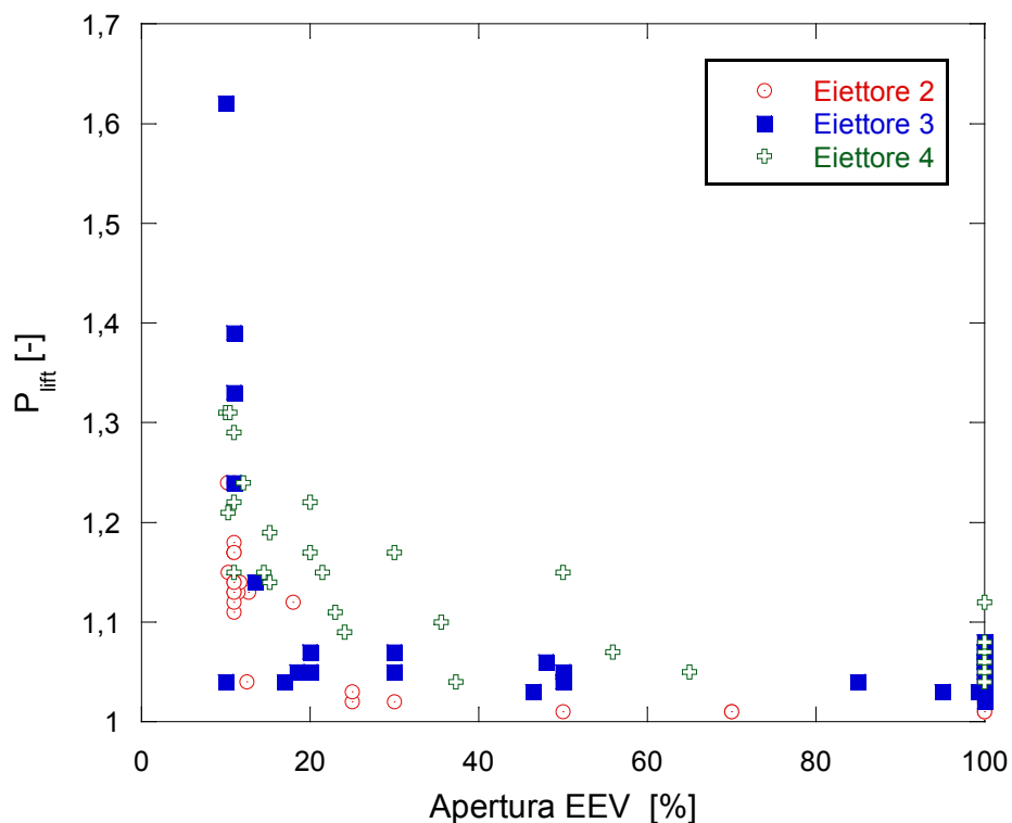
Figura 17 – Pressure lift in funzione del grado di apertura EEV – test riscaldamento/ACS Parametro: eiettore utilizzato
