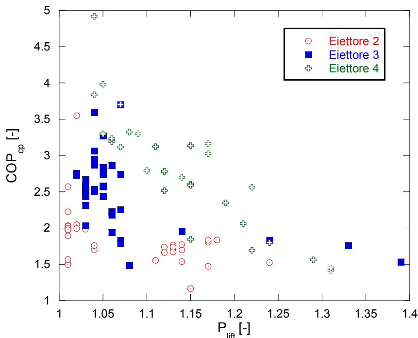
Figura 23 – COP in funzione del pressure lift – test riscaldamento/ACS Parametro: eiettore utilizzato
