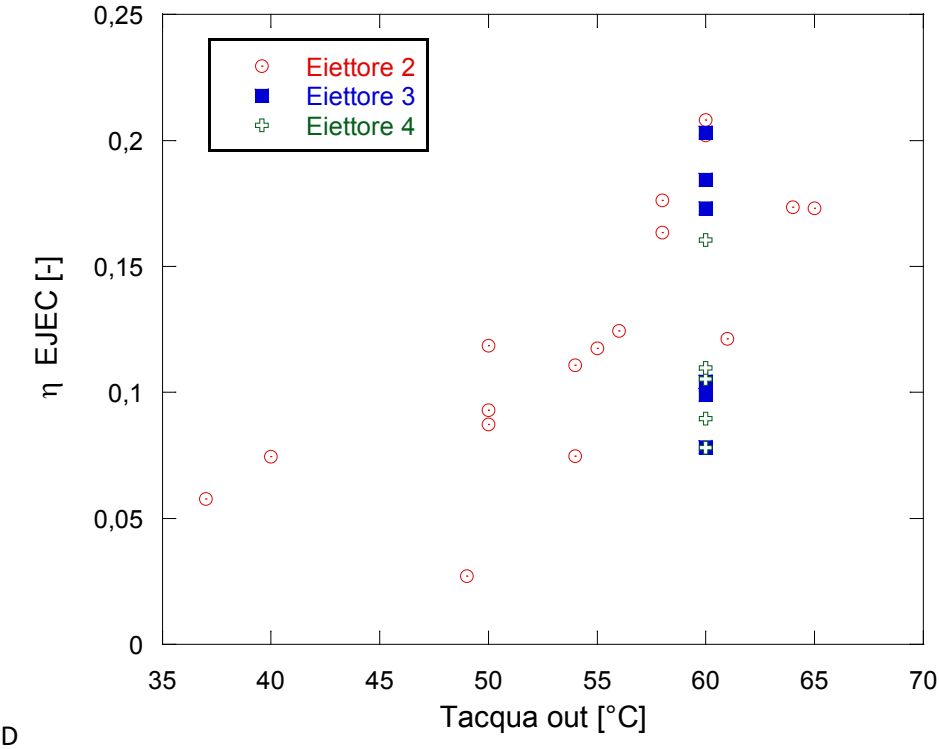
Figura 21 – Rendimento dell’eiettore in funzione della temperatura dell’acqua prodotta – test riscaldamento/ACS con apertura EEV minore del 12% - Parametro: eiettore utilizzato
