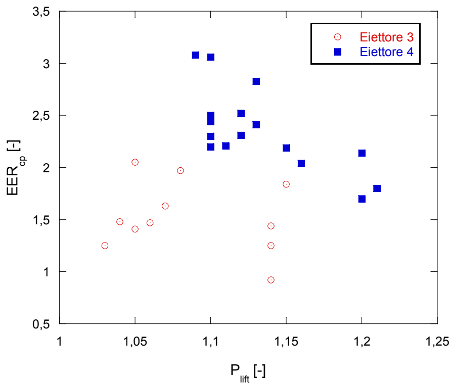
Figura 29 – EER in funzione del pressure lift – test raffreddamento Parametro: eiettore utilizzato
