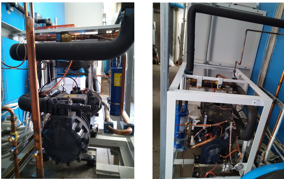
Figura 3 – Gruppo frigorifero potenziato
