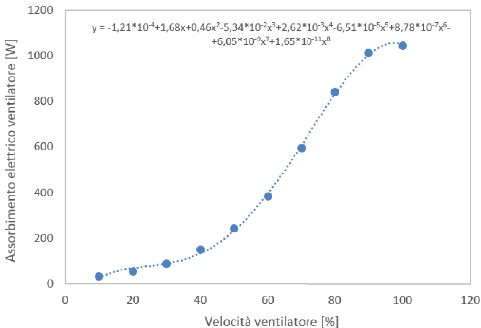
Figura 9 – Assorbimento elettrico ventilatori
