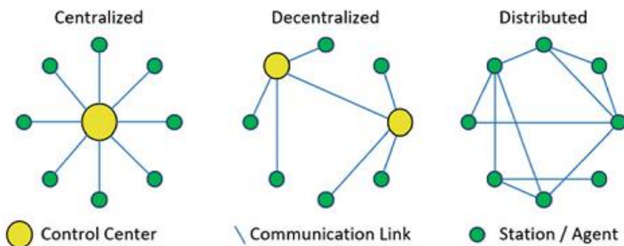
Figura 6: Esempi di reti di distribuzione energetica con strutture centralizzata, decentralizzata e distribuita (Hamidi, 2020)
