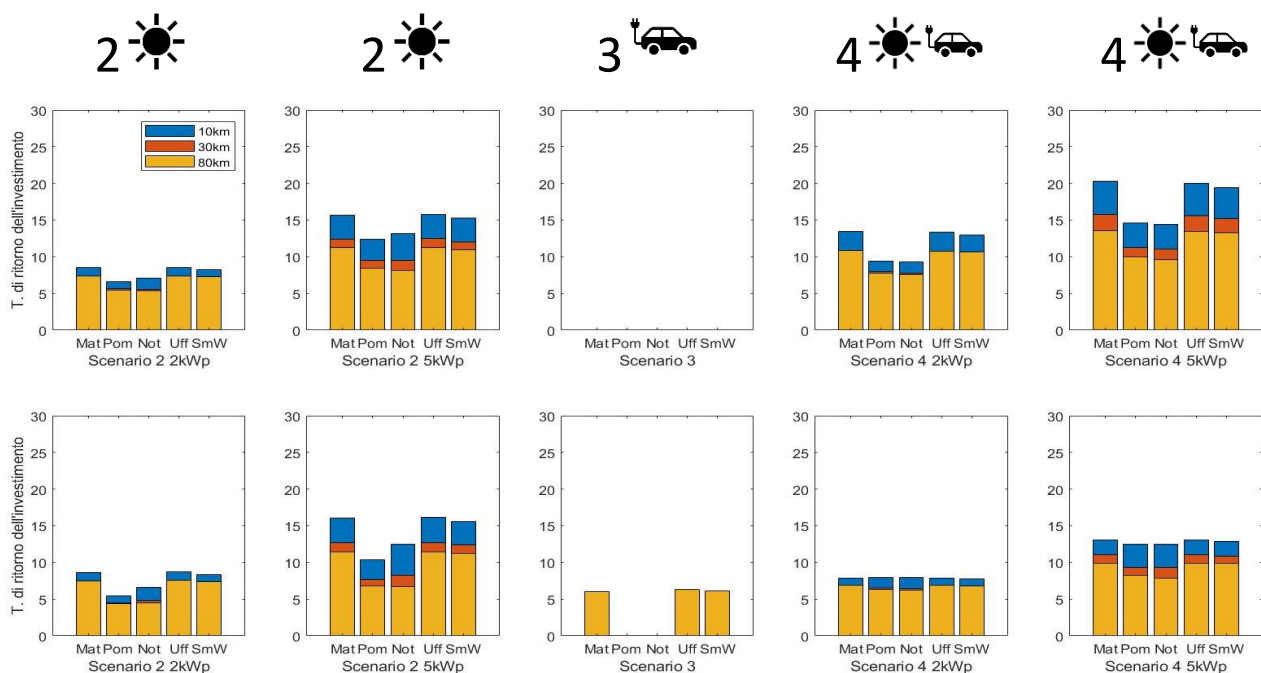
Figura 29 Tempi di ritorno dell'investimento per proprietario di Nissan Leaf
