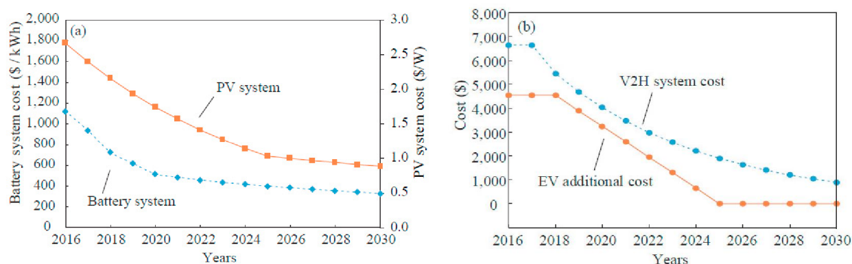
Figura 5: previsione dell'andamento dei prezzi di impianti fotovoltaici e batterie (a), caricatori bidirezionali e futura riduzione costi veicoli elettrici (b) (Kobashi & Yarime, 2019)
