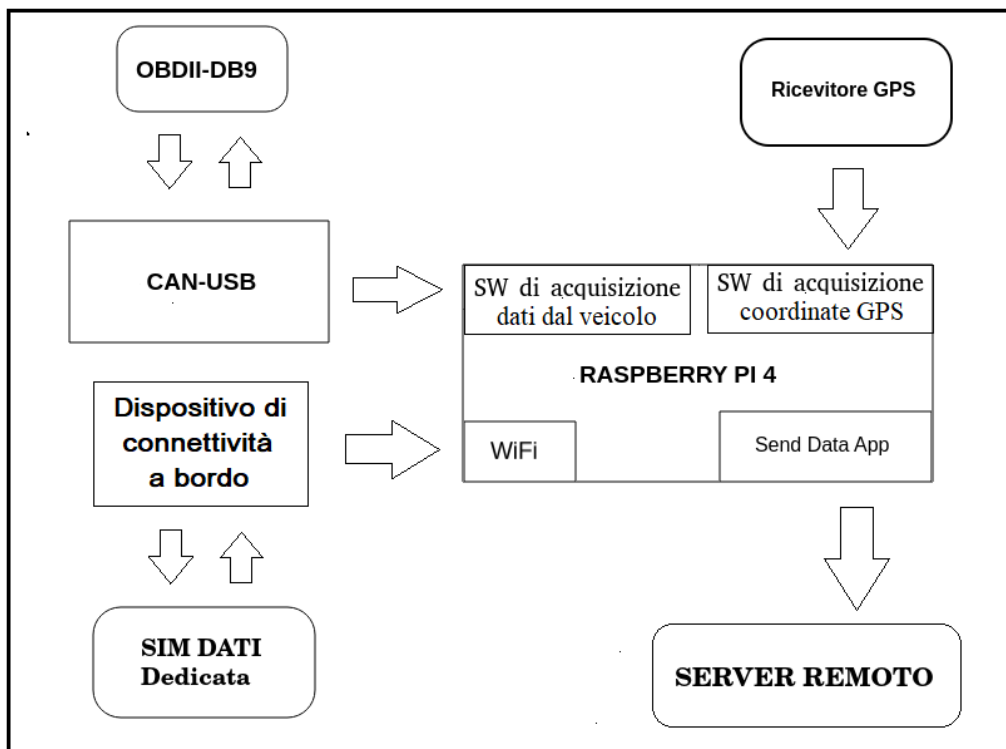
Figura 7- Gli elementi del sistema embedded
