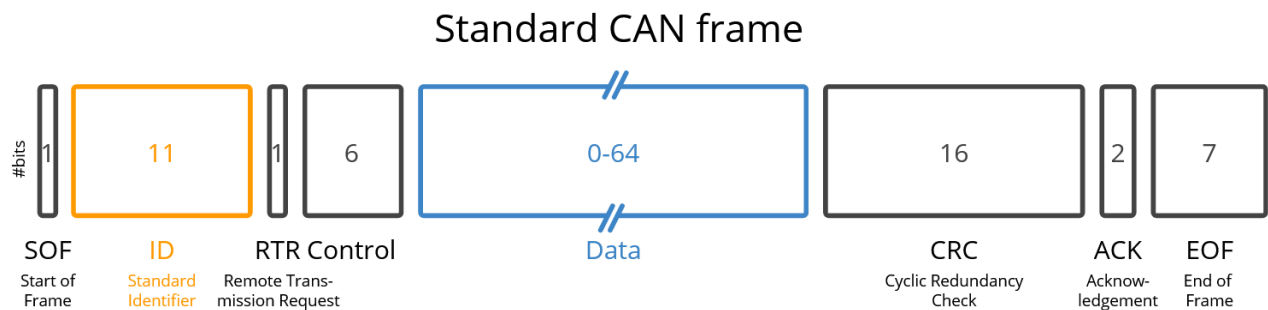
Figura 4- Struttura del frame CAN Bus
