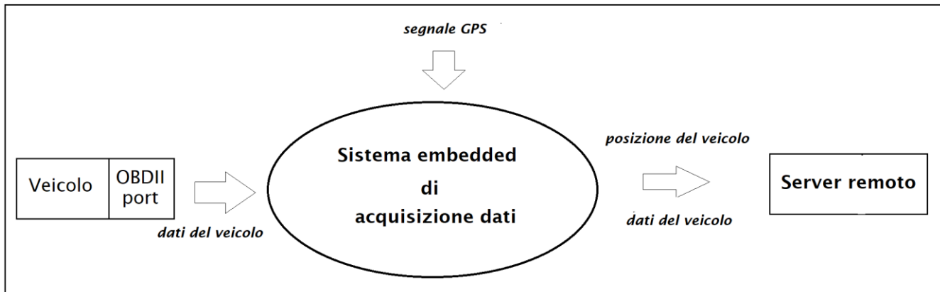
Figura 6 - Il sistema embedded di acquisizione dati
