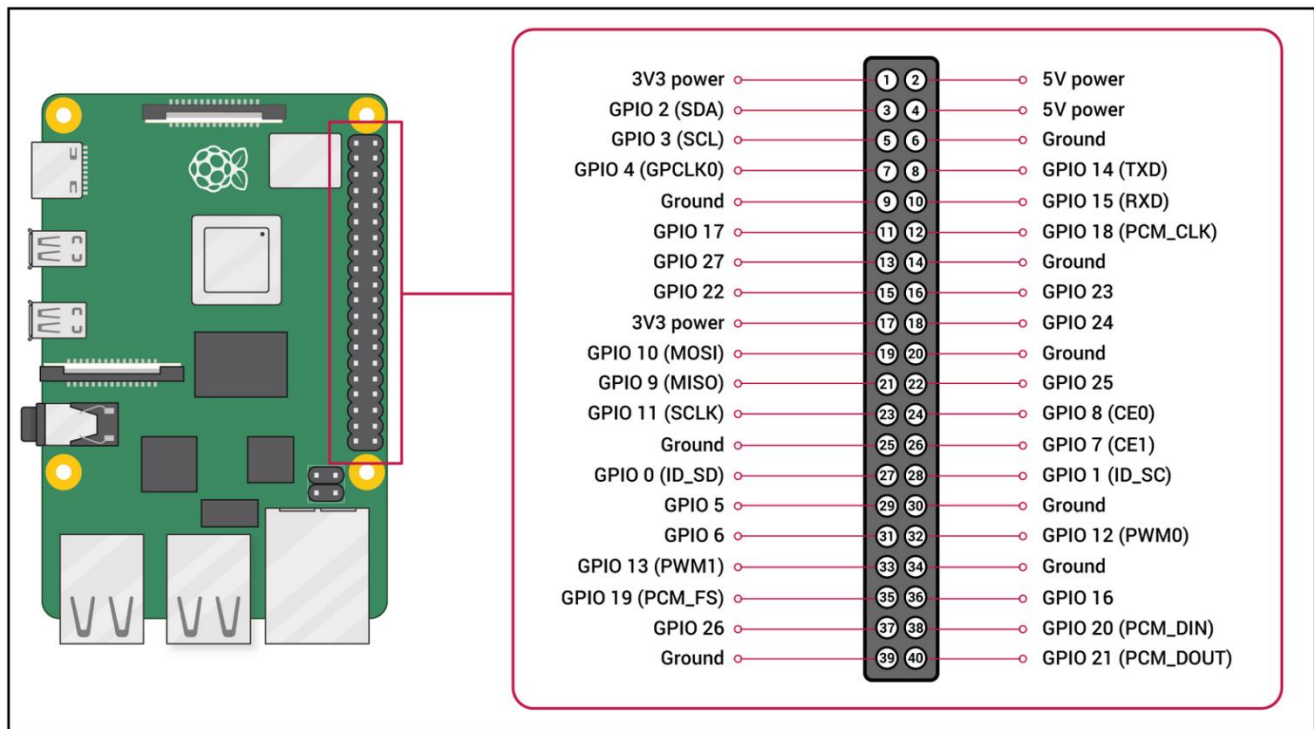
Figura 9- Piedinatura del GPIO del Raspberry PI 4
