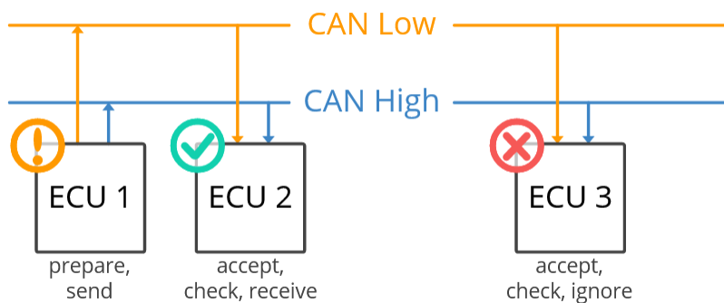
Figura 3-Funzionamento del CAN Bus
