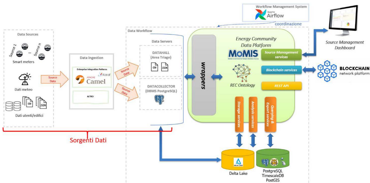
Figura 3 – Architettura finale Piattaforma MOMIS Industrial IoT
