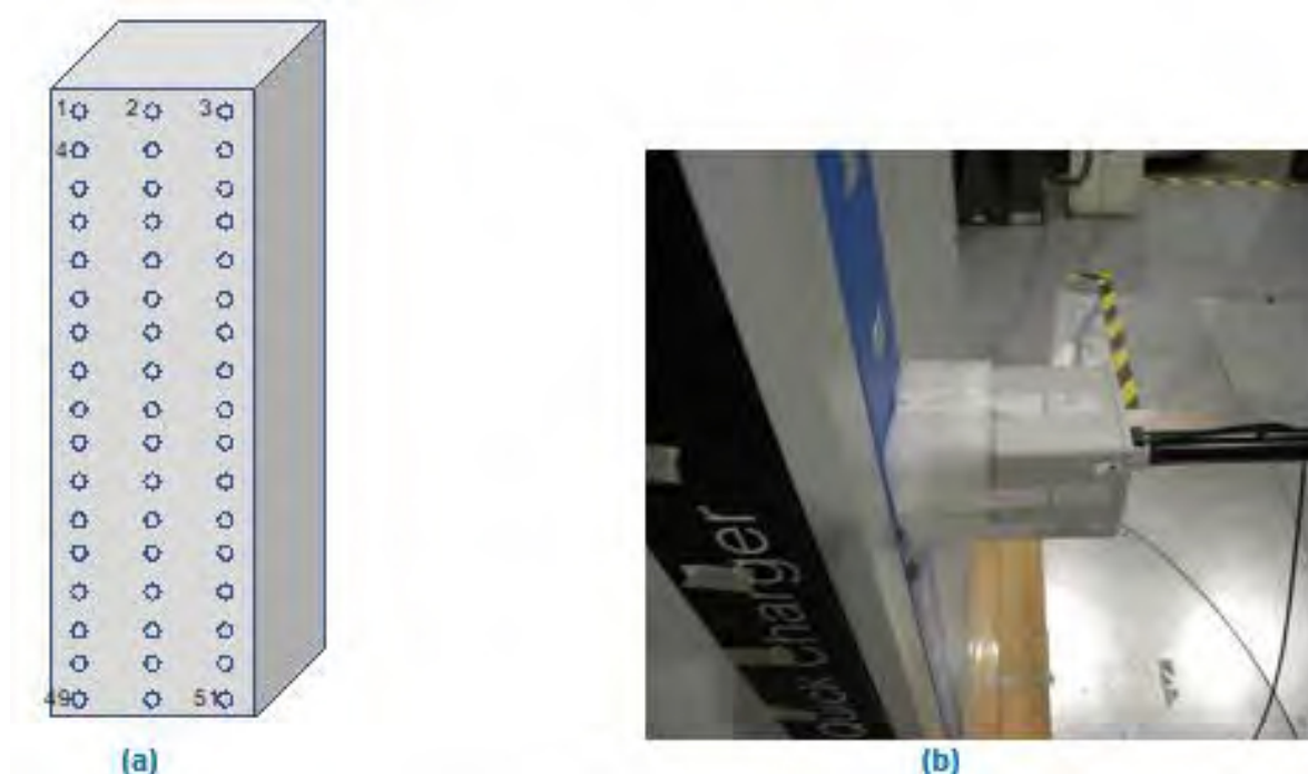
Figura 13 – Allestimento del set-up sperimentale: (a) schema dei punti di misura; (b) accorgimenti per velocizzare il preciso posizionamento del sensore.
