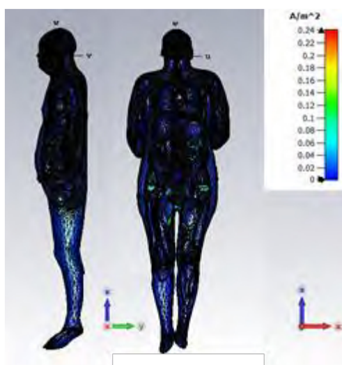
Figura 22: valori di J indotto dal sistema V2H mostrati sui piani sagittale e centrale frontale del modello (fondo scala 0.24 A/m²)
