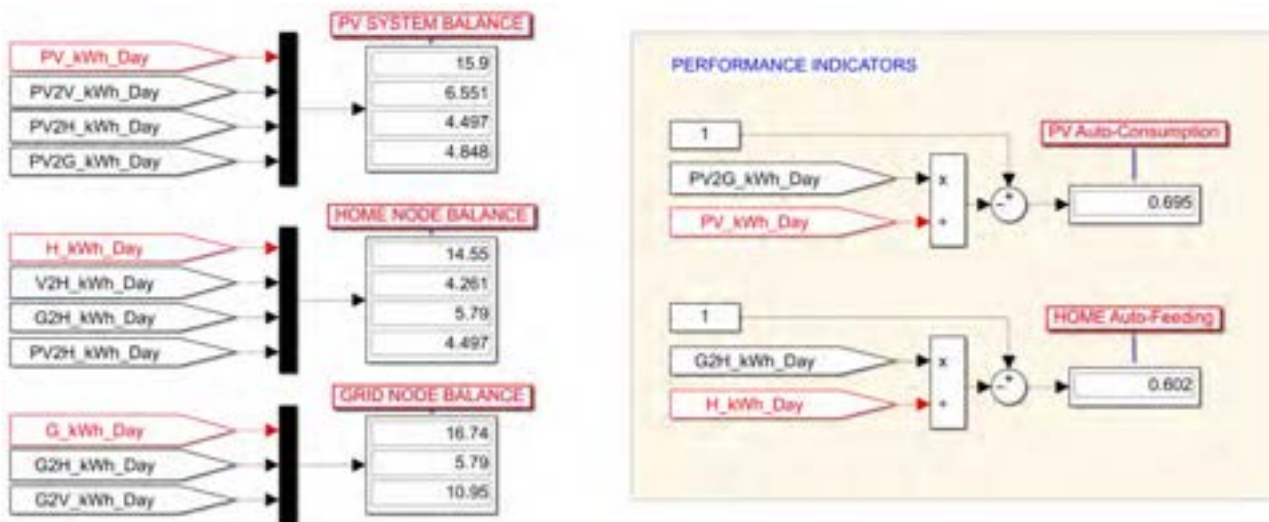
Figura 27: RETE DOMESTICA – INTERO ANNO. CASO 37 : "Nocturne Worker" con V2H MONO-BIREZIONALE.
