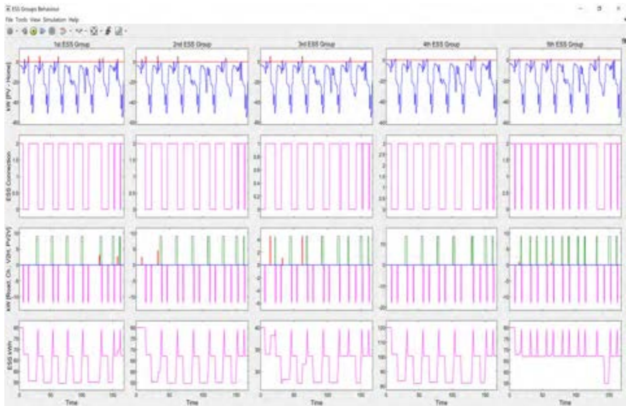
Figura 37: RETE CONDOMINIALE –INVERNO. CASO 1: Funzionalità V2H MONO-DIREZIONALI.
