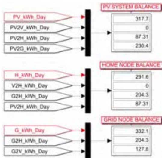
Figura 28: RETE CONDOMINIALE - INTERO ANNO. CASO BASE: Nessuna funzionalità V2H.
