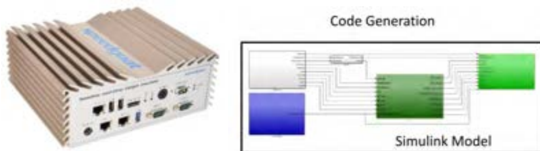
Figura 9: Strumentazione acquisita per l'implementazione sul prototipo dell'algoritmo di gestione proposto
