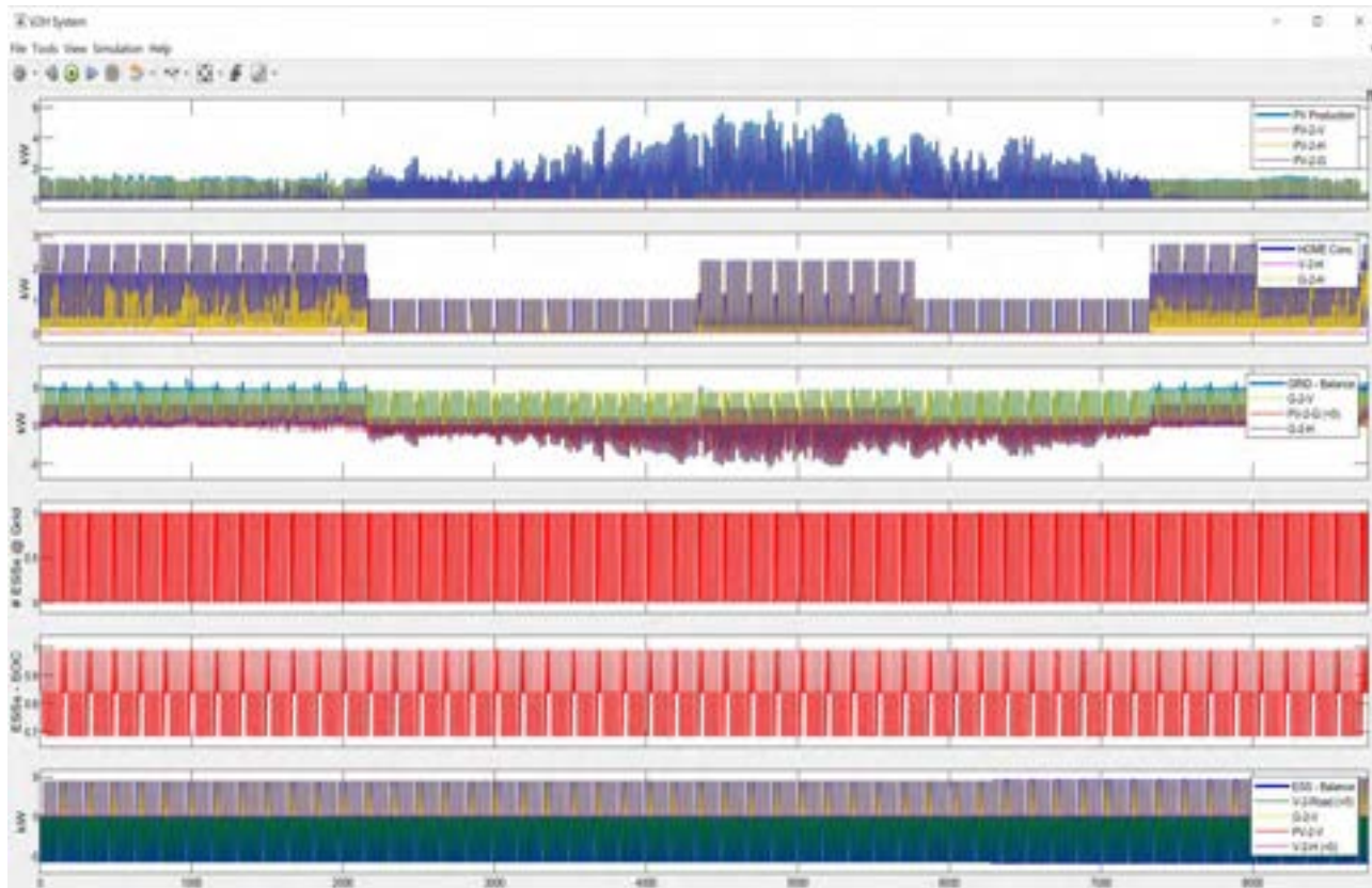
Figura 15: RETE DOMESTICA - INTERO ANNO. CASO BASE : "Office Worker" senza V2H.
