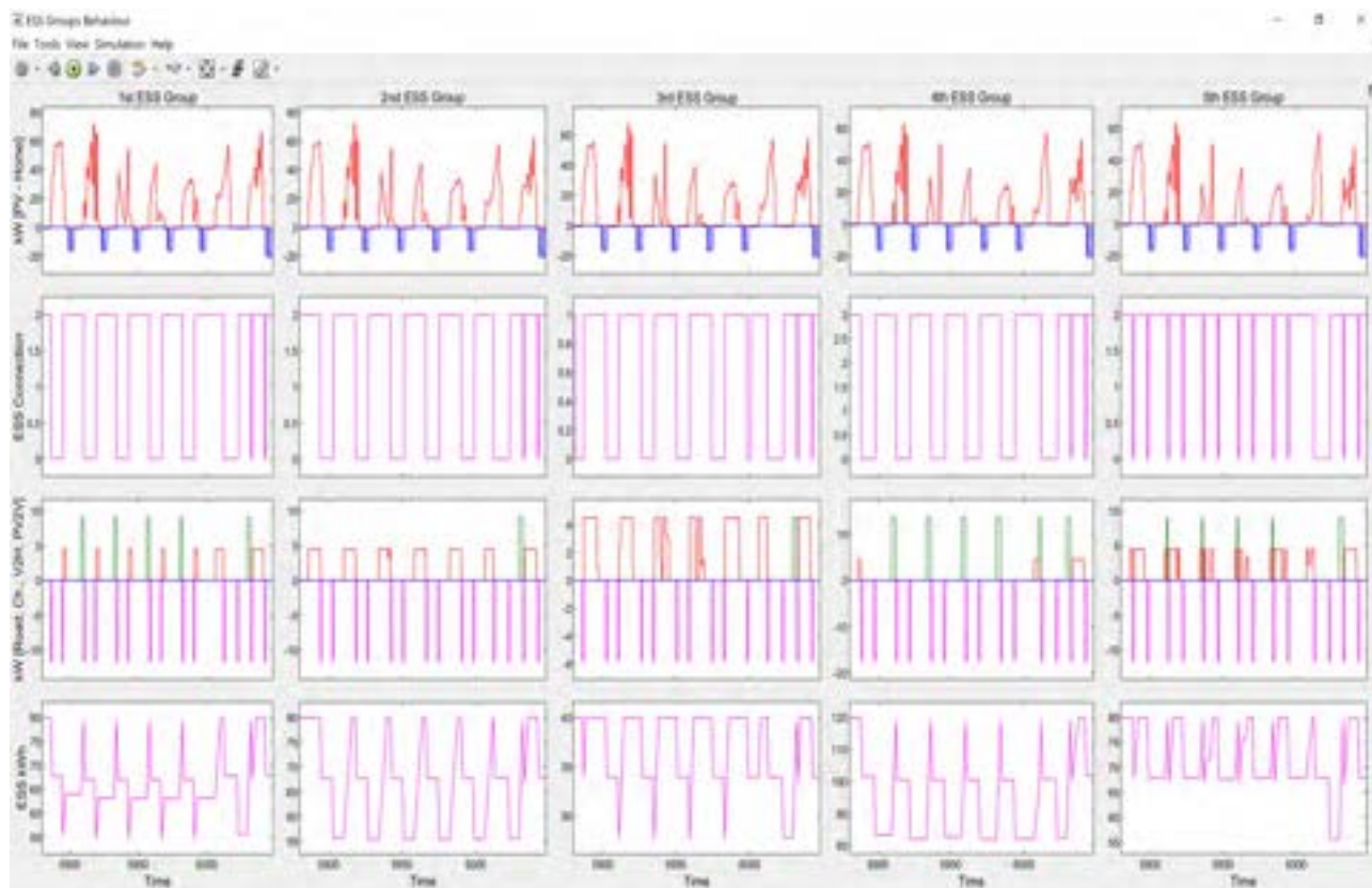
Figura 43: RETE CONDOMINIALE –AUTUNNO. CASO 1: Funzionalità V2H MONO-DIREZIONALI.
