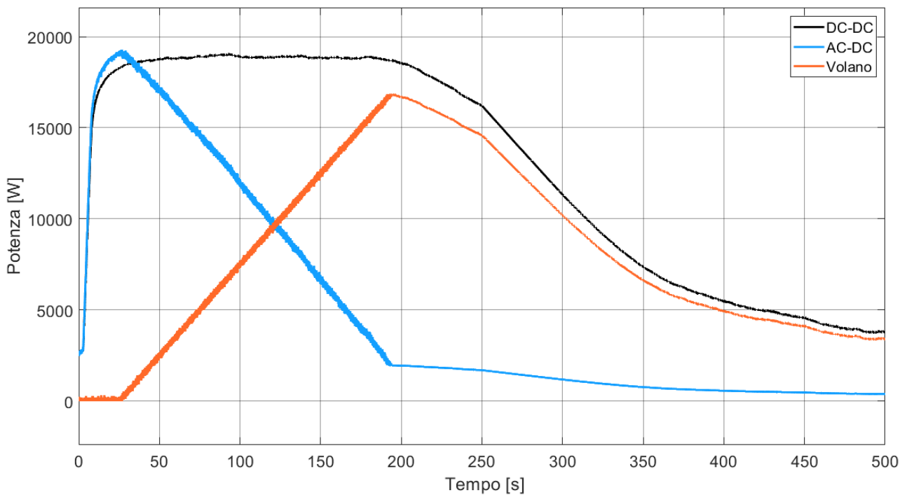
Figura 9: Potenze DCDC (verso la batteria), AC-DC (dalla rete elettrica) e del volano durante la ricarica
