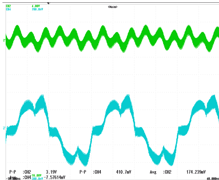
Figura 12: Valori di corrente sul convertitore ACDC collegato alla rete elettrica
