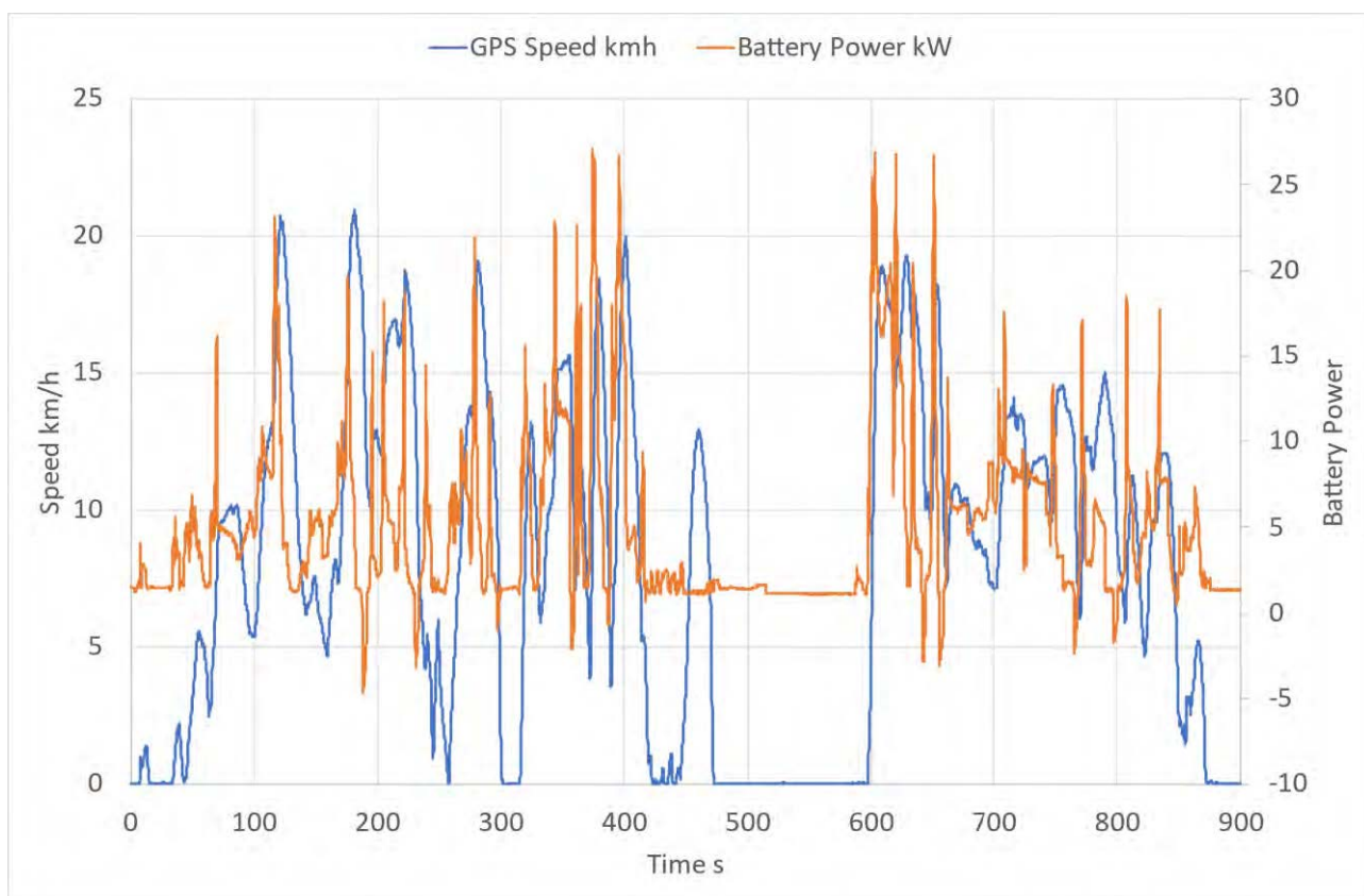
Figura 6: Andamento della velocità del minibus e della potenza erogata dalle batterie
