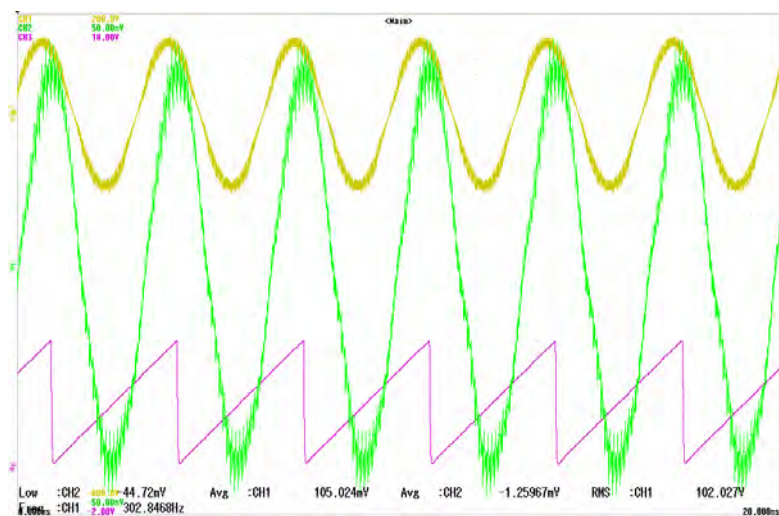
Figura 15: Valori di tensione, corrente e di fase dell'azionamento del volano
