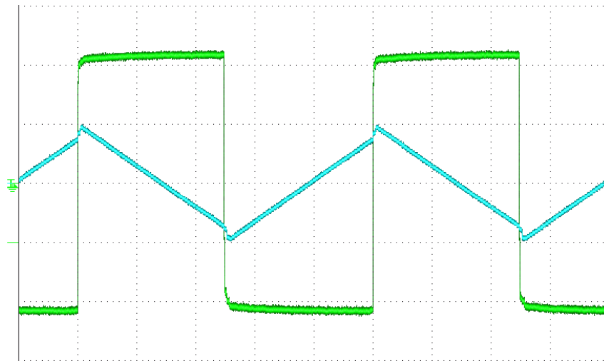
Figura 14: Correnti e tensioni relative al DCDC di uscita
