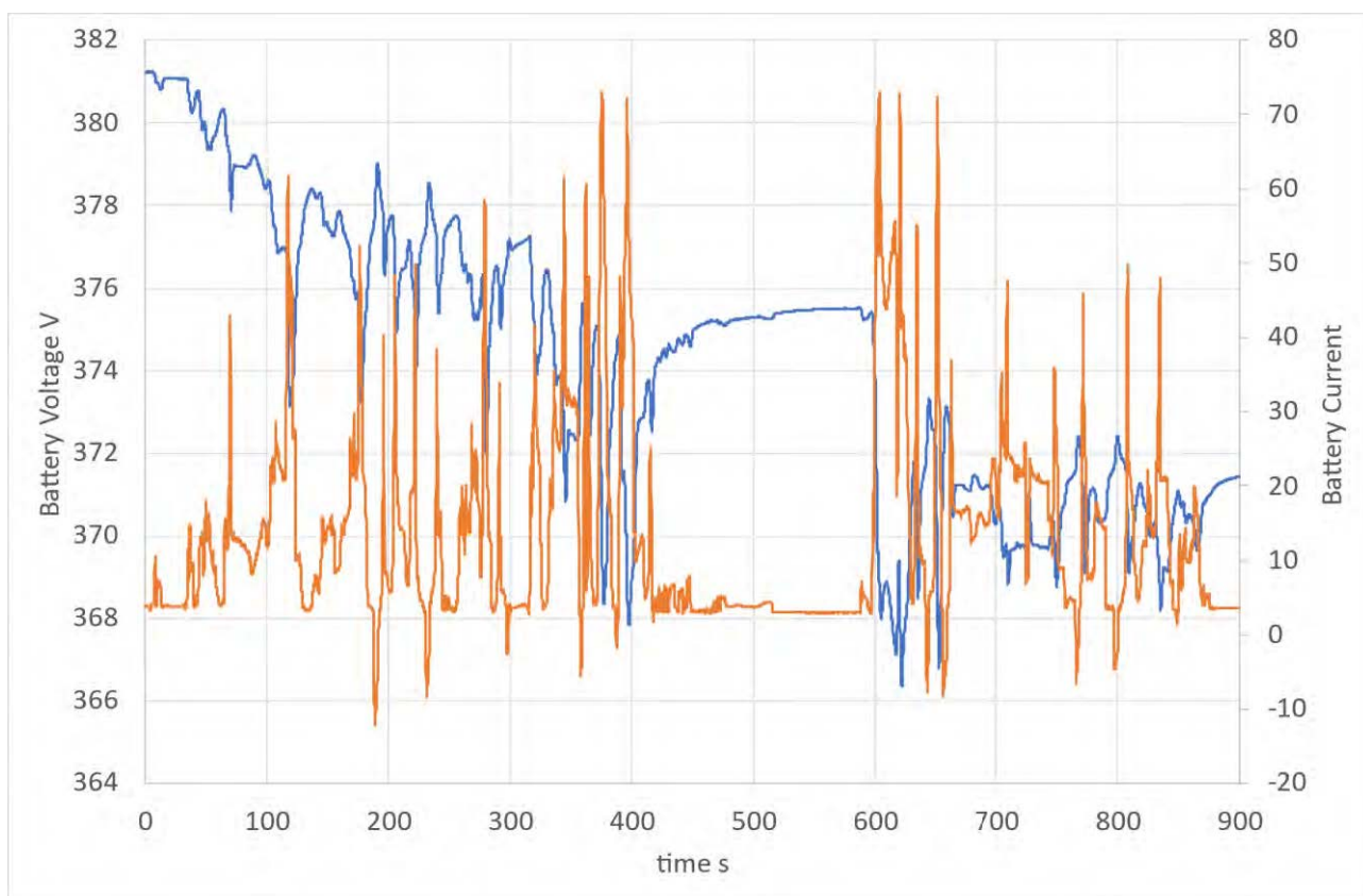
Figura 5: Andamento della tensione e della corrente durante la prova
