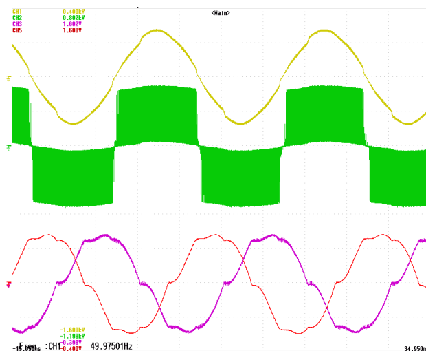
Figura 13: Valori di tensione e corrente in un test a Potenza nominale
