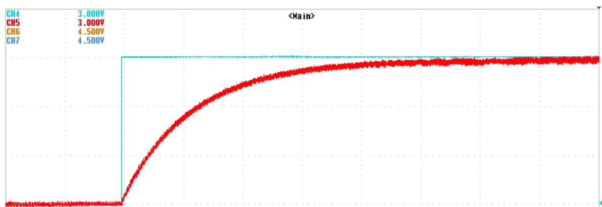
Figura 11: Transitorio di carica del volano da 0 rpm a velocità nominale. Asse x 4 min/div
