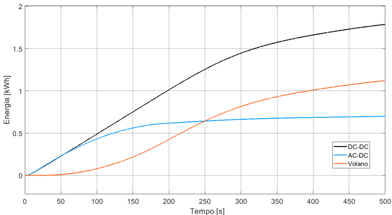
Figura 10: Andamento delle energie della rete elettrica (AC-DC), dal volano e verso la batteria.
