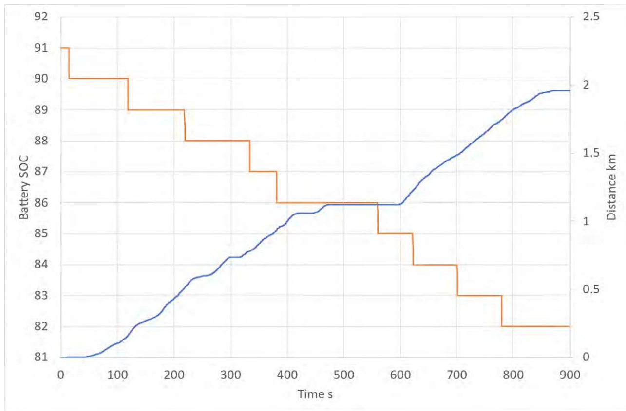
Figura 4: Andamento della distanza percorsa e dello stato di carica della batteria
