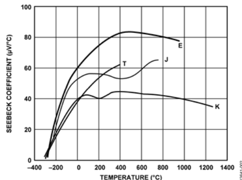
Figura 21: Coefficiente Seebeck per termocoppie J, T e K [10]
