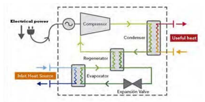
Figura 1: Schema Funzionale di una Pompa di Calore.
