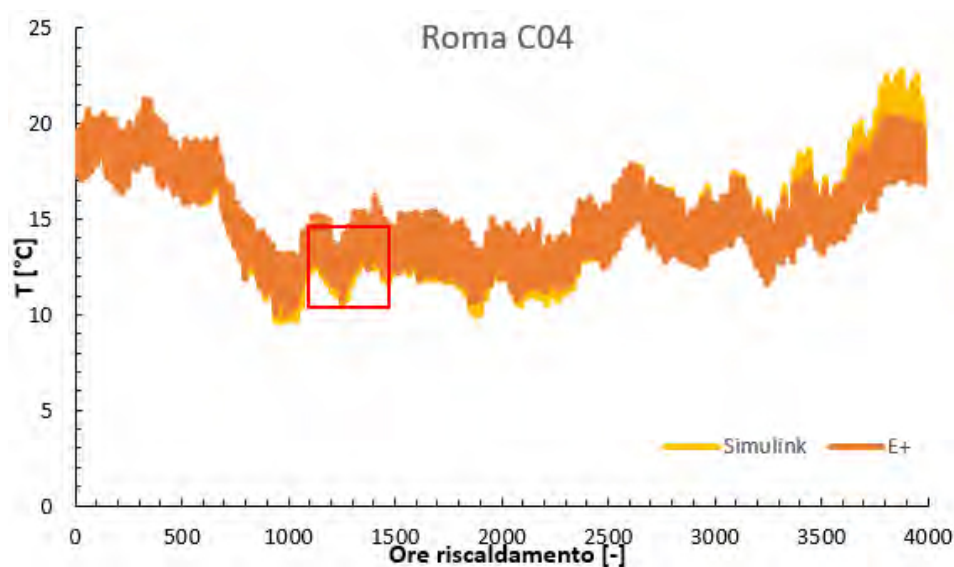
Figura 22: Confronto tra le temperature per il cluster C04 (UAM) a Roma – 1 occupante
