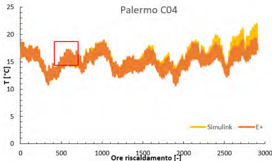
Figura 18: Confronto tra le temperature per il cluster C04 (UAM) a Palermo – 1 occupante
