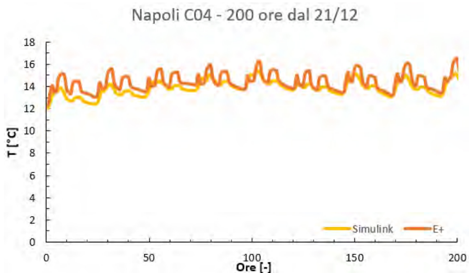
Figura 21: Dettaglio settimana caratteristica invernale - Napoli C04 (UAM) – 1 occupante
