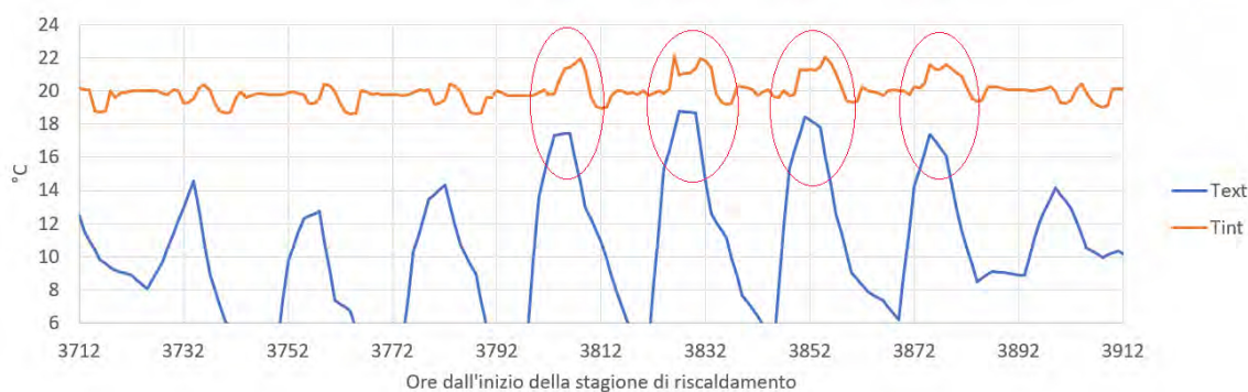
Figura 61 – Confronto tra andamenti di temperatura dell'aria esterna (Text) e dell'aria interna (Tint). Nelle zone cerchiate si evidenziano le accensioni della pompa di calore con set-point maggiorato. Caso di UAC, C01, Milano, profilo 1P, C-CAP2
