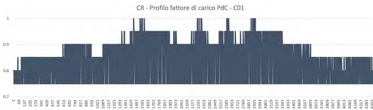
Figura 13 – Andamento fattore di carico della pompa di calore (Milano, UAM, C01, 1p)
