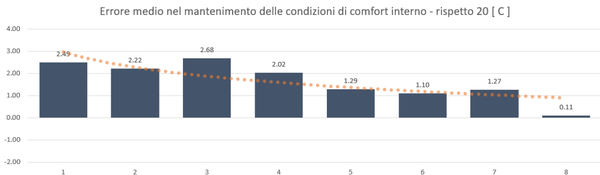
Figura 16 – Scostamento medio tra valore di riferimento e valori ottenuti dalle simulazioni per la temperatura dell'aria interna (esempio di Milano, UAM, 1p, tutti i cluster)
