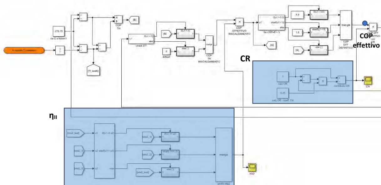
Figura 7 – Rappresentazione schematica del modello logico per il calcolo del COP effettivo realizzato su Matlab/Simulink
