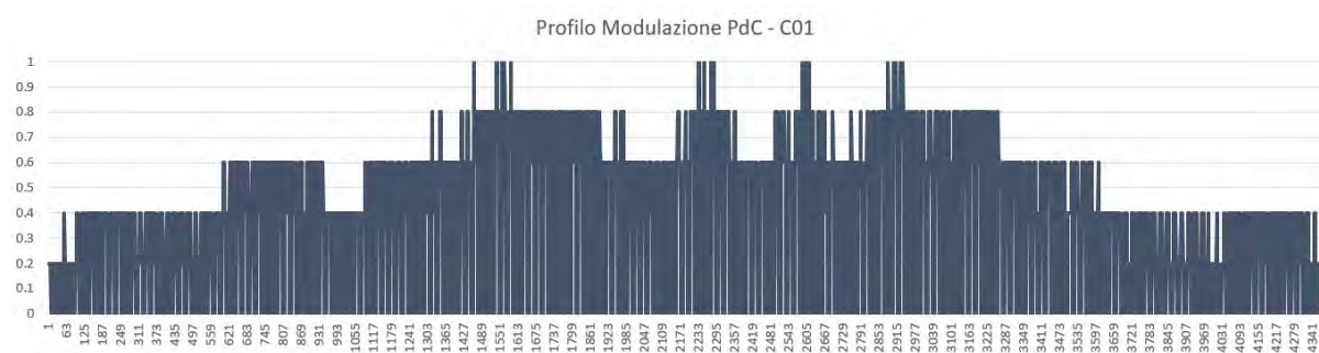
Figura 12 – Andamento modulazione della pompa di calore (Milano, UAM, C01, 1p)
