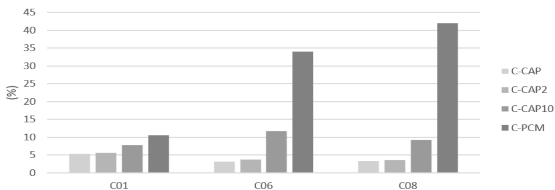
Figura 58 – Riduzioni percentuali dei consumi energetici stagionali ottenuti per le differenti combinazioni (tra configurazioni di funzionamento e cluster costruttivi) analizzate, rispetto alla configurazione di base, caso di UAC ubicata a Milano occupata con profilo 1p
