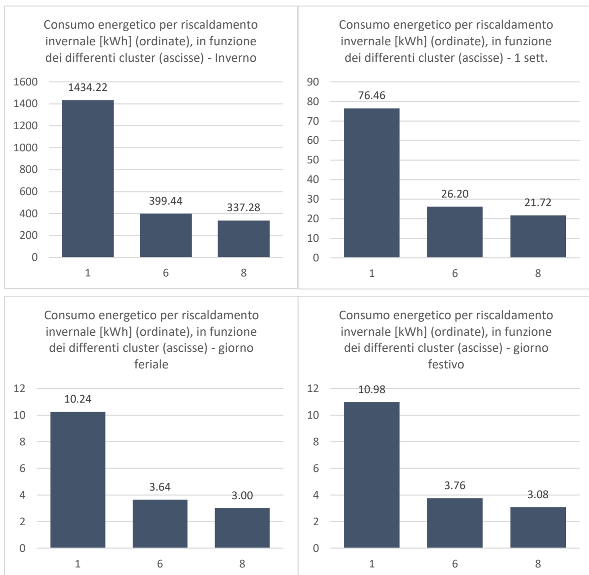
Figura 57 – Consumo energetico per riscaldamento invernale per la configurazione di funzionamento C-CAP10, tipologia UAC a Milano con profilo di occupazione 1p
