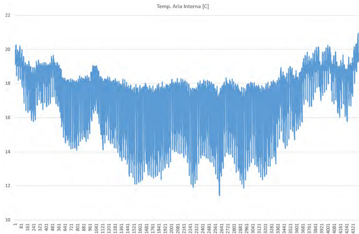
Figura 11 – Andamento temperatura aria interna (Milano, UAM, C01, 1p)
