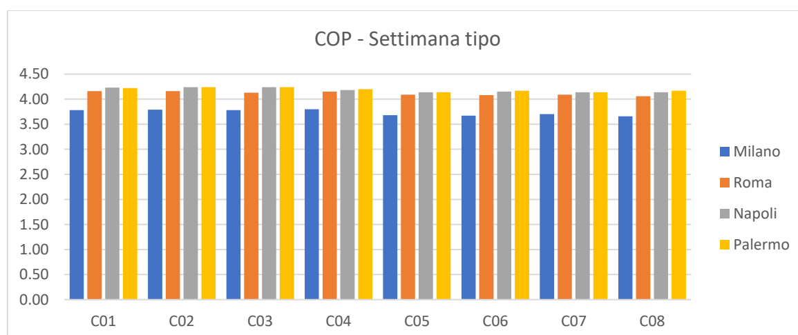
Figura 32 – Valore medio del COP nella settimana tipo per le quattro località climatiche, nel caso di unità abitativa UAC e profilo di occupazione 1p
