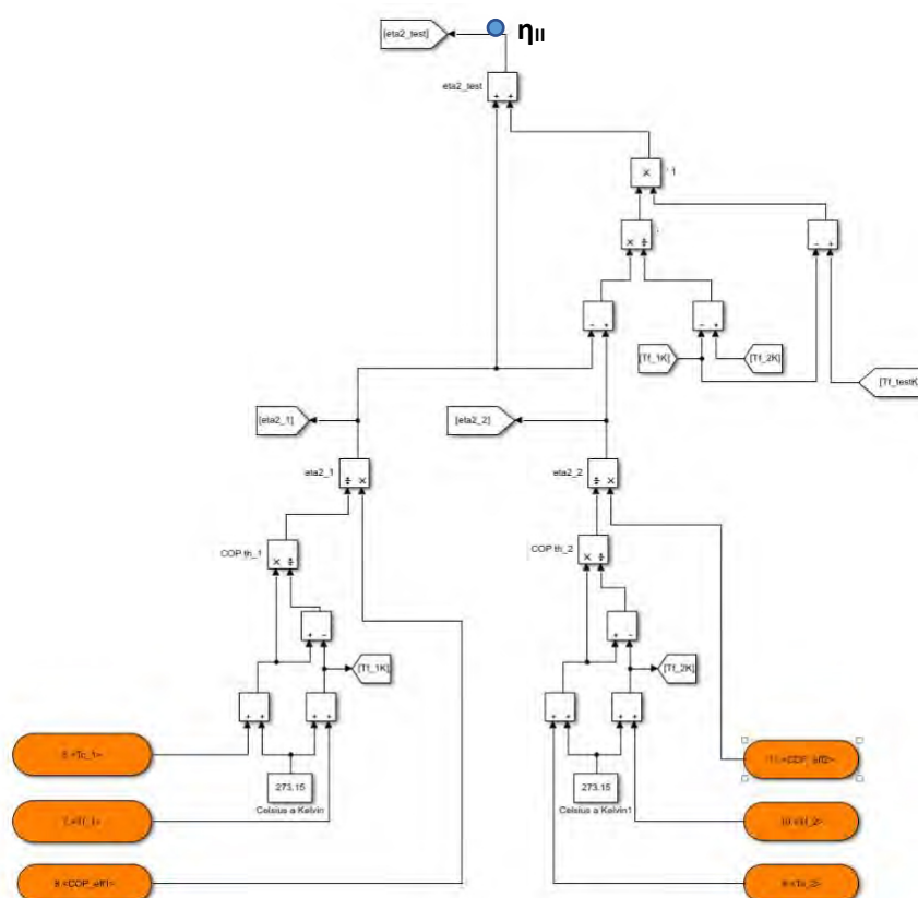
Figura 6 – Rappresentazione schematica del modello logico per il calcolo del rendimento di secondo principio realizzato su Matlab/Simulink
