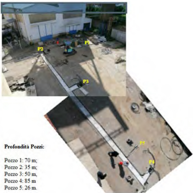
Figura 1. Vista dall’alto del campo geosonde e ubicazione dei pozzi geotermici con relative profondità
