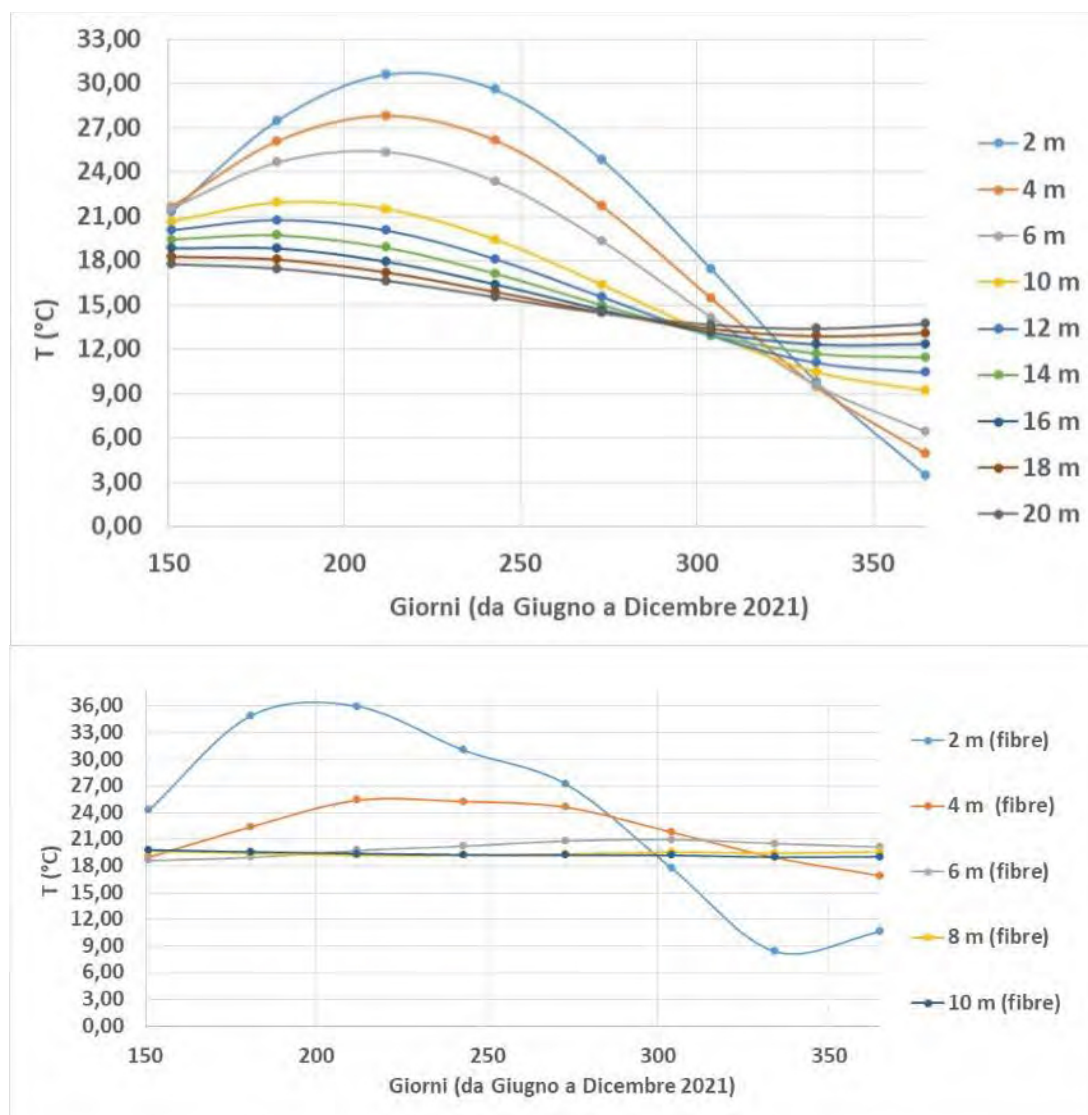
Figura 15. Confronto tra le temperature del terreno a diverse profondità in funzione del tempo e quelle corrispondenti misurate dalle fibre ottiche nel pozzo 4 (periodo giugno-dicembre 2021)
