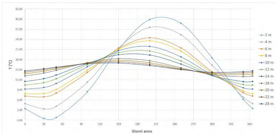
Figura 14. Temperatura del terreno a diverse profondità in funzione del tempo (anno 2021)
