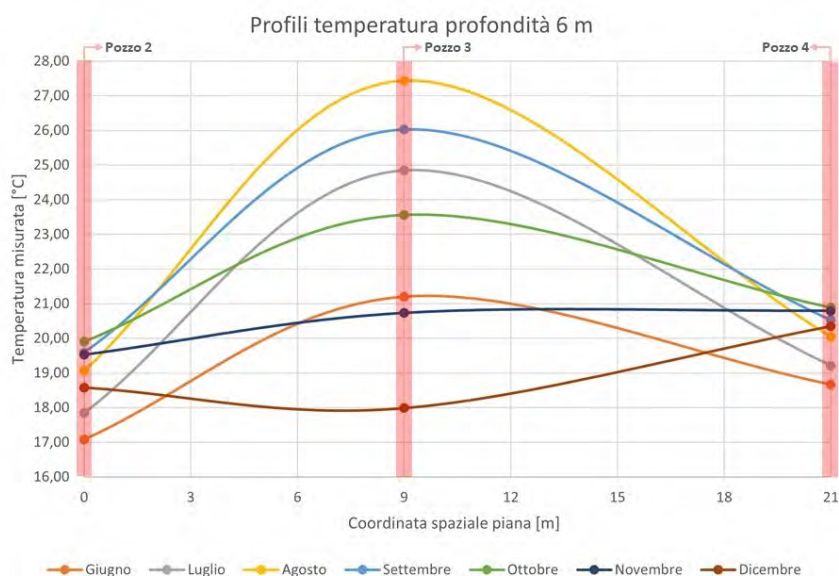
Figura 17. Andamento della temperatura mensile alla profondità di 6 m in coordinata spaziale piana
