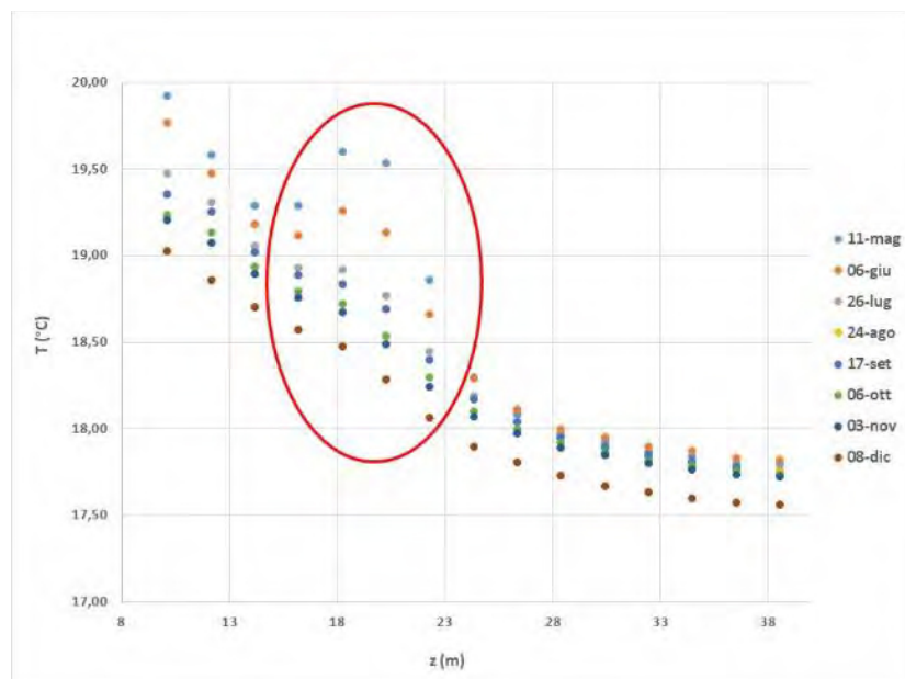
Figura 21. Andamento delle temperature nel pozzo 4 nei giorni più piovosi del 2021
