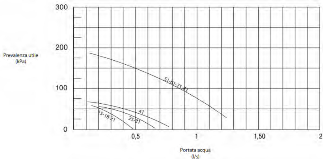
Figura 27. Curva prevalenza utile della pompa in funzione della portata
