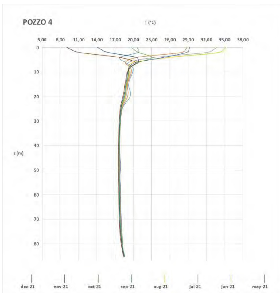
Figura 5. Profilo di temperatura del pozzo 4 in funzione della profondità nei diversi mesi dell'anno
