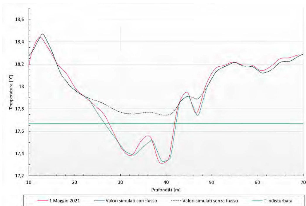
Figura 11. Simulazione conducibilità termica
