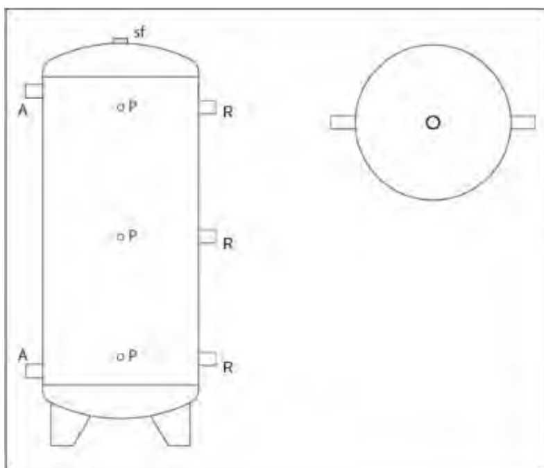
Figura 30. Schema del serbatoio di accumulo con uscite per componenti e tubazioni
