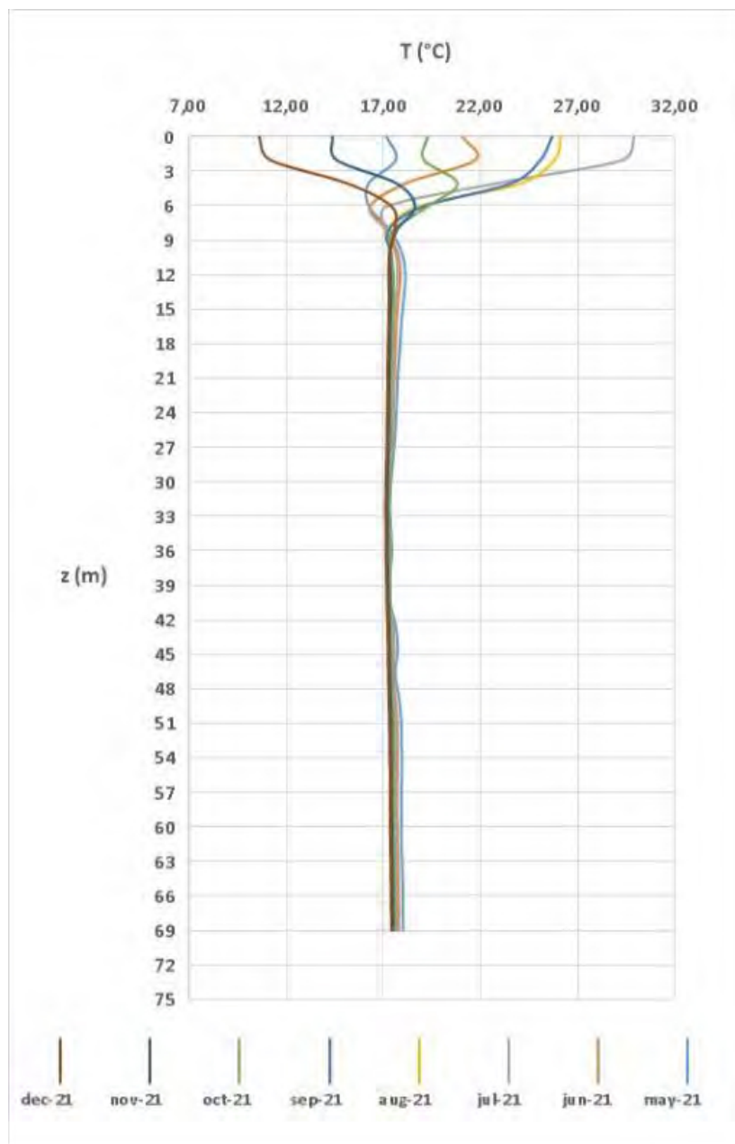
Figura 2. Profilo di temperatura del pozzo 1 in funzione della profondità nei diversi mesi dell'anno
