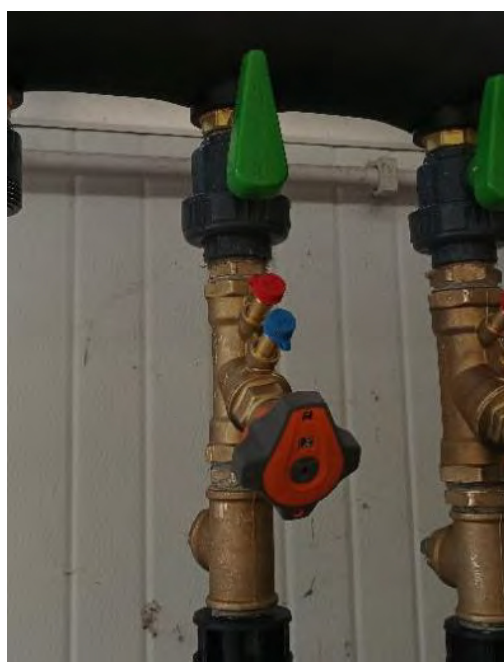
Figura 25. Valvola per regolazione di portata
