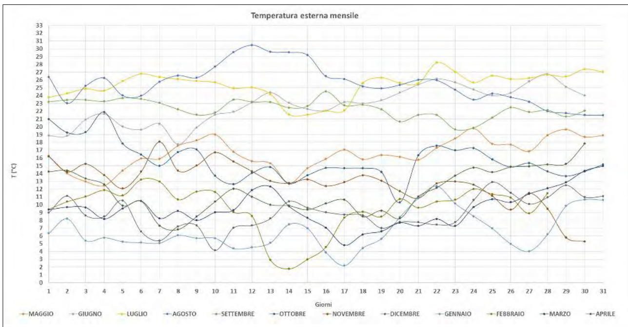
Figura 12. Andamento della temperatura esterna mensile nel C.R. ENEA-Casaccia (anno 2021)
