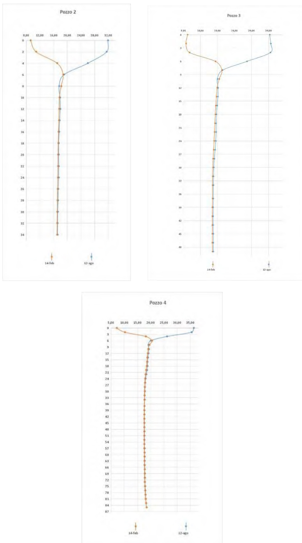
Figura 13. Andamento della temperatura nel giorno più caldo e in quello più freddo del 2021 (pozzi 2,3 e 4)
