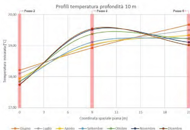
Figura 19. Andamento della temperatura mensile alla profondità di 10 m in coordinata spaziale piana
