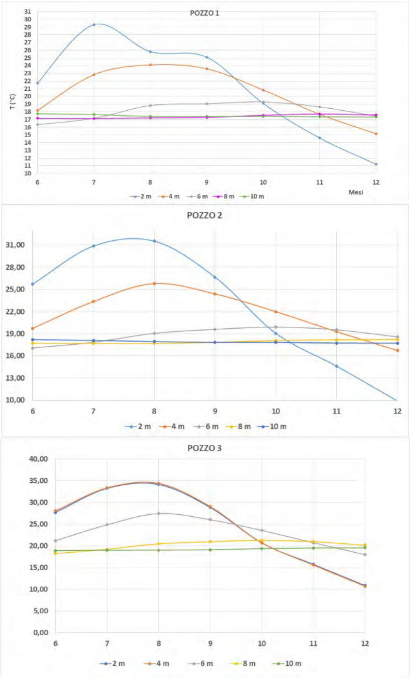
Figura 16. Andamento delle curve di temperatura nei pozzi 1, 2 e 3 in funzione della profondità (periodo giugno-dicembre 2021)
