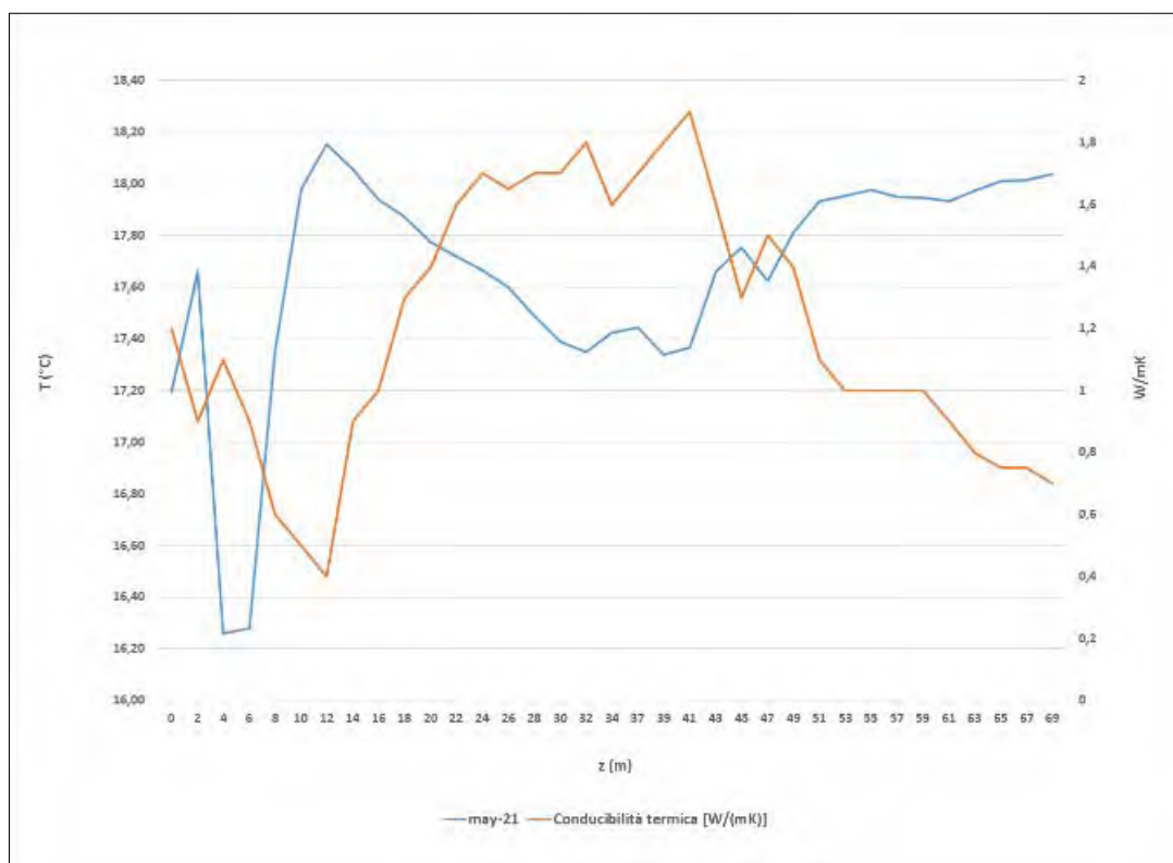
Figura 7. Correlazione tra profilo di temperatura e conducibilità termica (W/mK)
