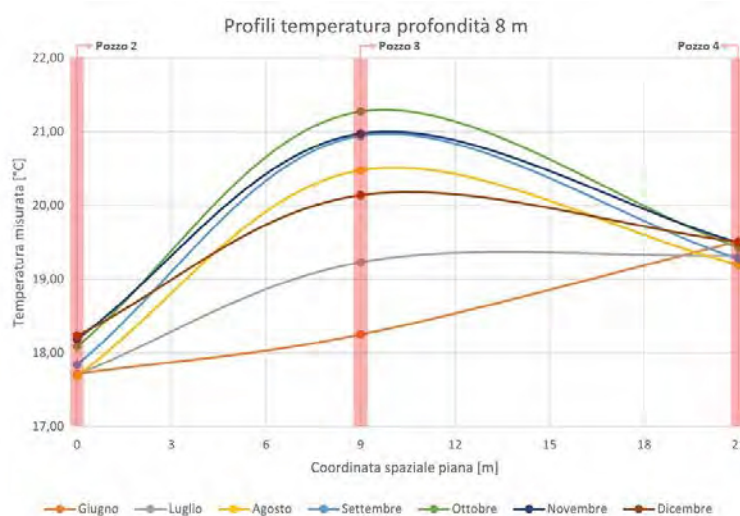
Figura 18. Andamento della temperatura mensile alla profondità di 8 m in coordinata spaziale piana
