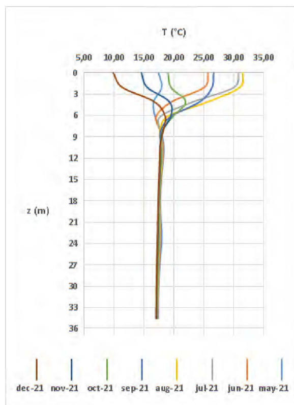
Figura 3. Profilo di temperatura del pozzo 2 in funzione della profondità nei diversi mesi dell'anno
