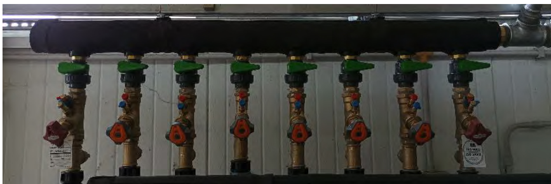
Figura 24. Valvole di regolazione di portata (collettore di mandata alle sonde)
