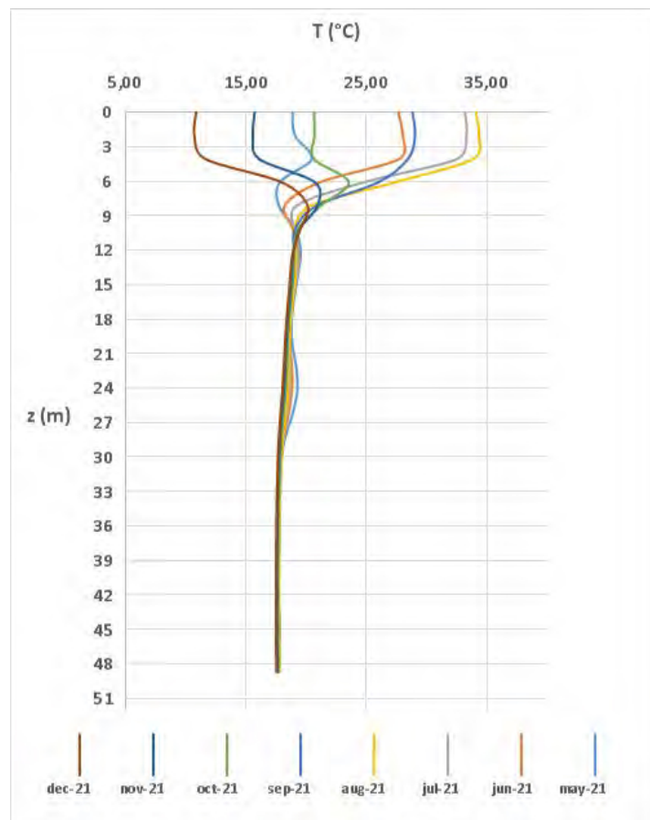
Figura 4. Profilo di temperatura del pozzo 3 in funzione della profondità nei diversi mesi dell'anno
