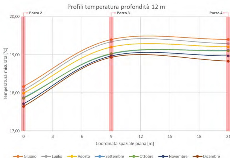
Figura 20. Andamento della temperatura mensile alla profondità di 12 m in coordinata spaziale plana
