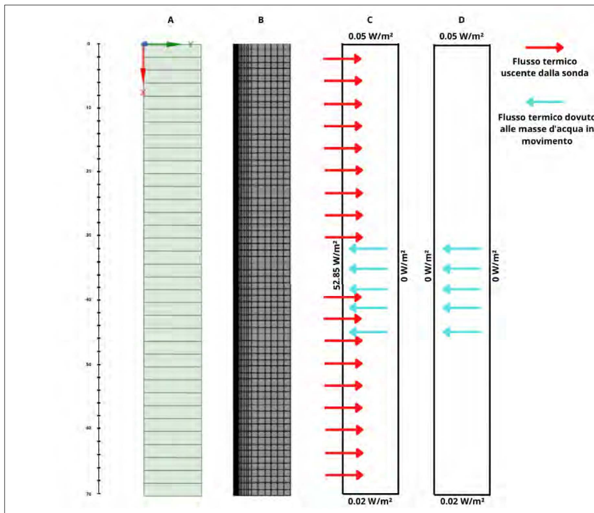
Figura 8. A: modello geometrico stratigrafico; B: mesh; C: condizioni al contorno "Periodo 1"; D: condizioni al contorno "Periodo 2"
