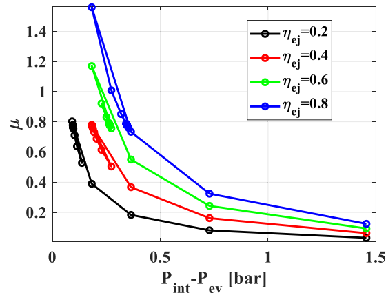
Figura 7 – Andamento del rapporto di trascinamento \mu in funzione della differenza tra pressione intermedia e dell'evaporatore, per diversi valori del rendimento eietttore [7]
