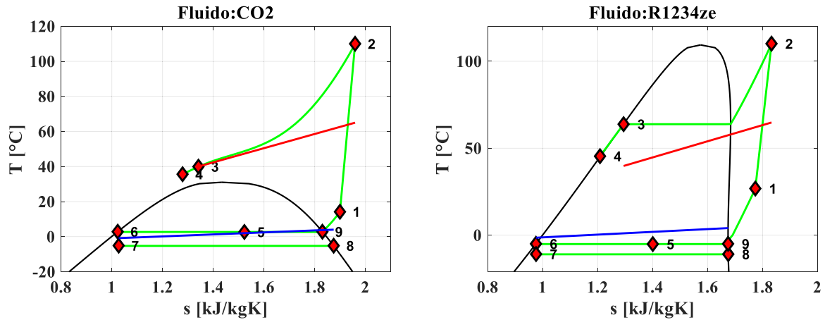
Figura 10 - Diagramma T-s in modalità acqua calda sanitaria per fluidi CO 2 (sx) e R1234ze (dx), per la città di Milano e per rendimento eiettore 0.4
