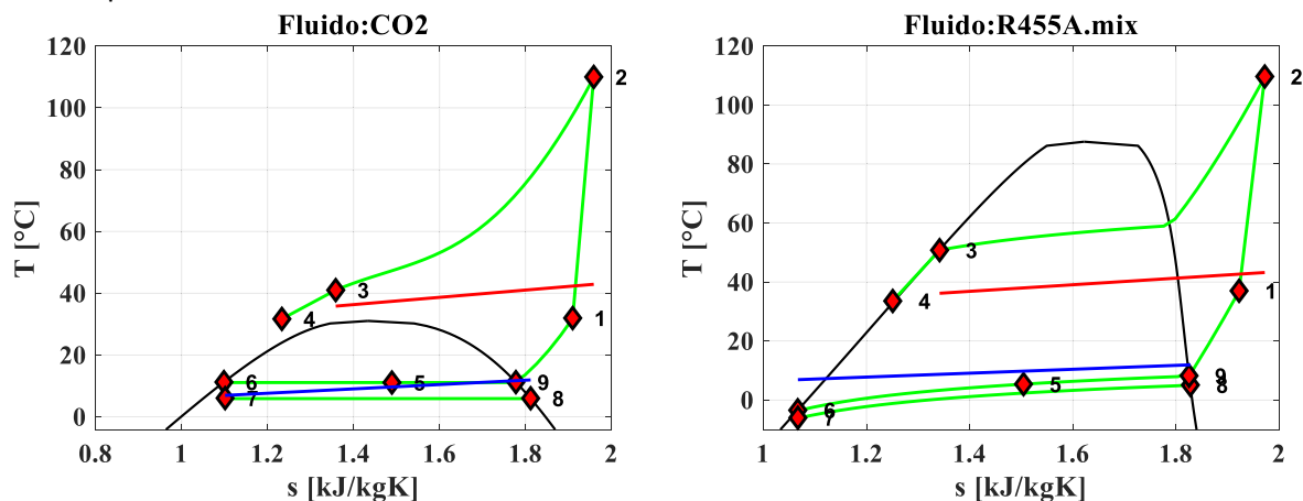
Figura 9 - Diagramma T-s in modalità raffrescamento per fluidi CO 2 (sx) e R455A (dx), per la città di Palermo e per rendimento eiettore 0.4
