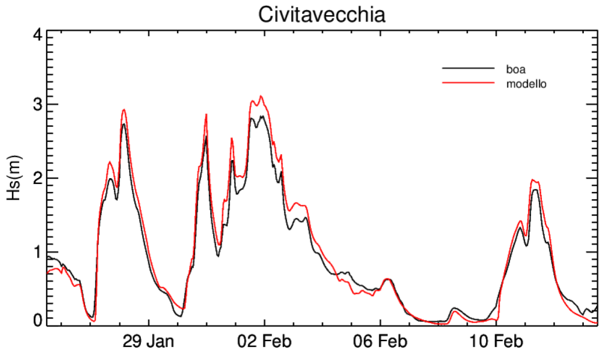
Figura 3 – Confronto dell'altezza significativa ricavata dalla simulazione con il modello WW3 con il valore registrato alla boa di Civitavecchia.
