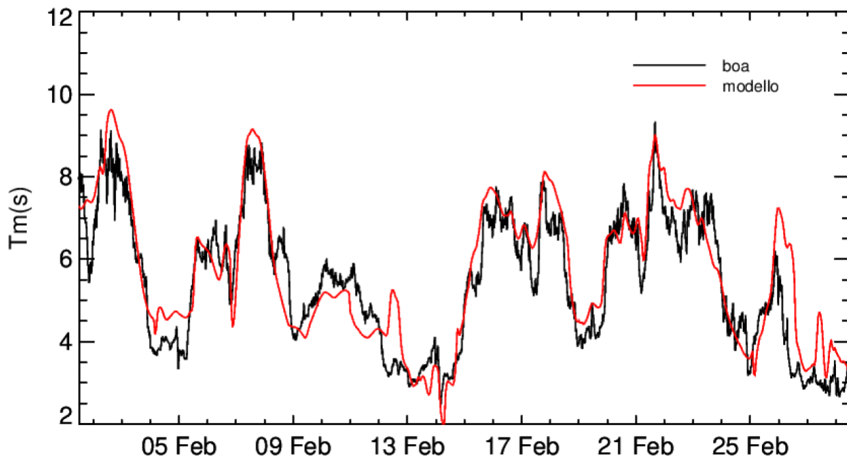
Figura 10 – Confronto del periodo medio dell'onda ricavato dal primo giorno di simulazione del sistema operativo con la boa di La Spezia, per il mese febbraio 2022.
