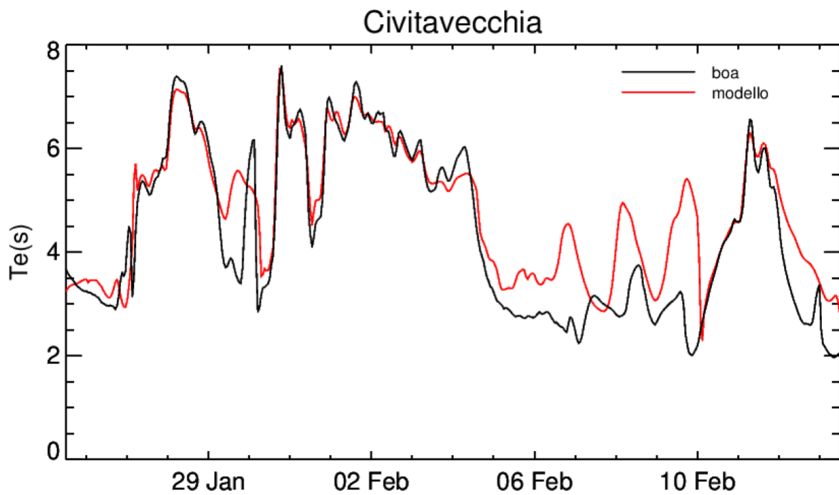
Figura 4 – Confronto del periodo medio dell'onda ricavato dalla simulazione con il modello WW3 con il valore registrato alla boa di Civitavecchia.
