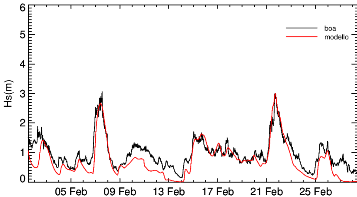
Figura 9 – Confronto dell'altezza significativa ricavata dal primo giorno di simulazione del sistema operativo con la boa di La Spezia, per il mese febbraio 2022.
