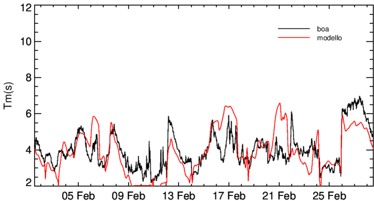
Figura 14 – Confronto del periodo medio dell'onda ricavato dal primo giorno di simulazione del sistema operativo con la boa di Ancona, per il mese febbraio 2022.
