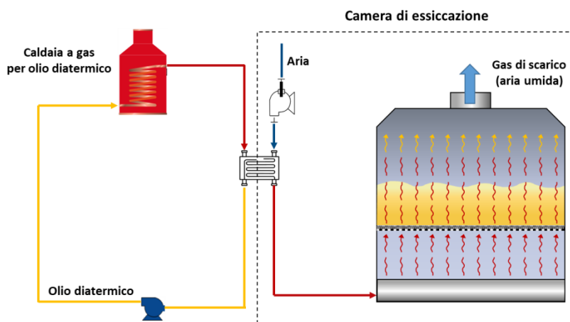
Figura 32. Schema di processo convenzionale per l'essiccazione del malto.
