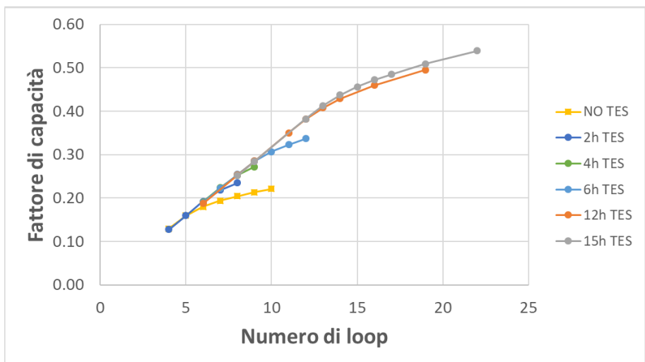
Figura 17. Andamento del fattore di capacità in funzione del numero di loop e al variare della dimensione dello stoccaggio termico.
