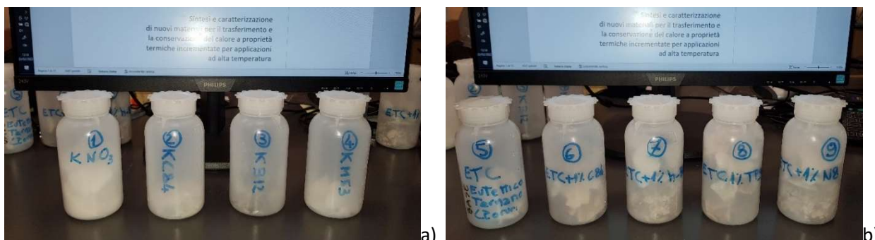
Figura 7. Campioni di NEPC prodotti a base di: a) KNO 3 e b) ETC
