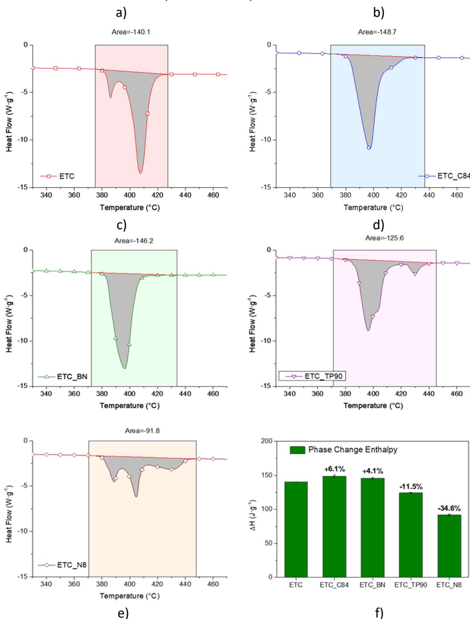
Figura 12. Curve DSC nell'intorno della fusione al II° riscaldamento dei NEPCM a base di ETC ; definizione delle aree per il calcolo delle entalpie specifiche di fusione per i campioni di: a) ETC, b) ETC_C84, c) ETC_BN, d) ETC_TP90, e) ETC_N8, f) confronto e variazioni delle entalpie medie dei NEPCM
