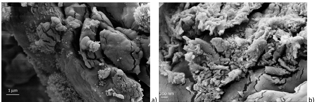
Figura 22. Micrografia del KNO 3 con nanocarica di COK84 a: a) 25000x , b) 50000x
