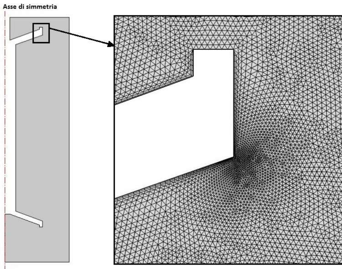
Figura 7- Particolare del mesh per il modello CFD del TES a termoclino
