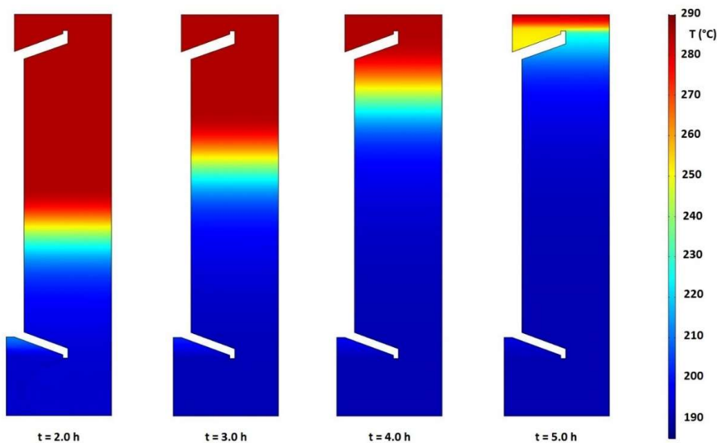
Figura 9- Campo termico all'interno del sistema di accumulo termico a termoclino dopo 2 ore, dopo 3 ore, dopo 4 ore e dopo 5 ore dall'inizio della fase di scarica
