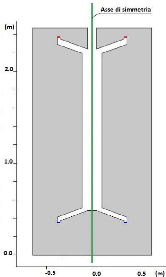
Figura 2- Sezione passante per l'asse di simmetria del sistema di accumulo termico a termoclino
