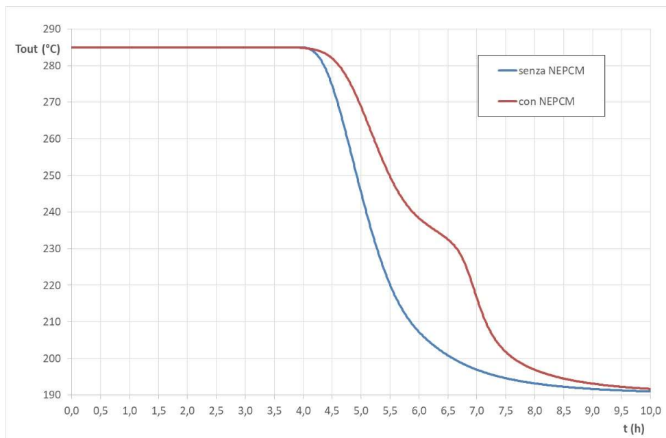
Figura 15- Andamento temporale delle temperature di uscita del sale ternario dal sistema di accumulo termico nei due modelli
