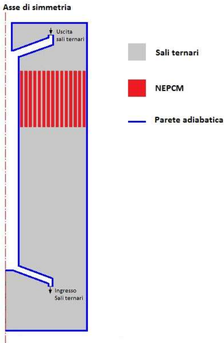
Figura 11- Condizioni al contorno modello sistema di accumulo termico a termoclino con NEPCM
