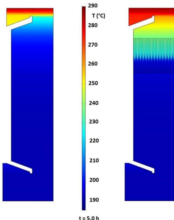
Figura 18- Confronto tra i campi termici all'interno dei due sistemi di accumulo termico, al tempo t = 5.0 h
