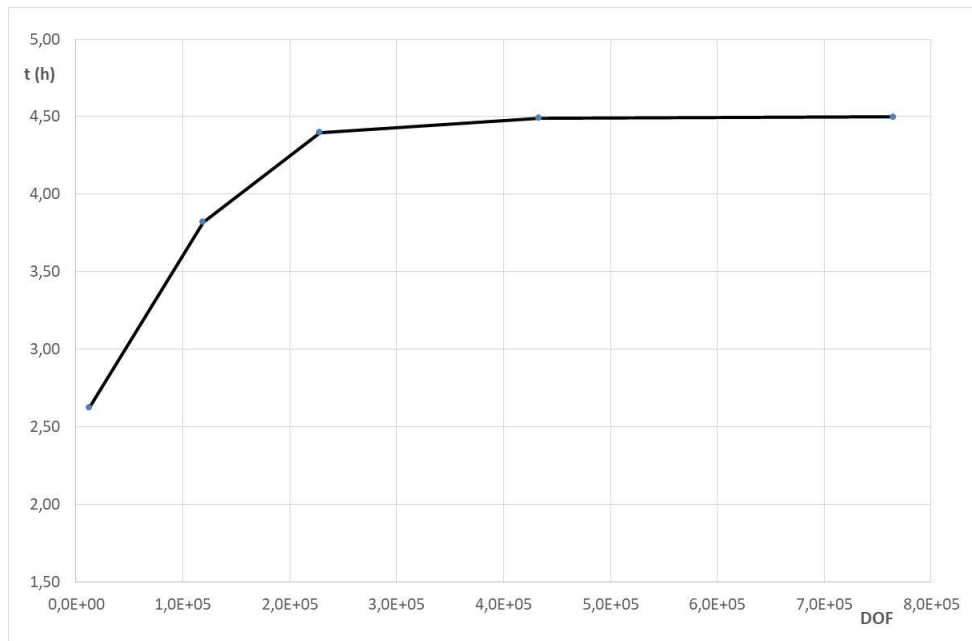
Figura 6- Andamento del tempo necessario al raggiungimento di T_{out}=275^{\circ}\text{C} in funzione del numero di gradi di libertà (DoF)
