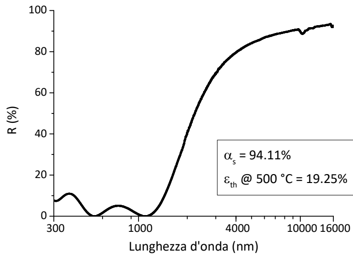
Figura 1. Riflettanza del coating solare realizzato per operare in aria a 500 °C
