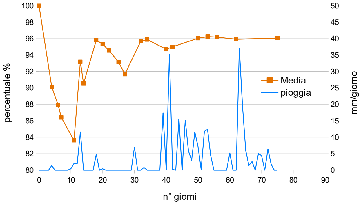
Figura 3: in rosso la riflettanza media a 660 nm e 12.5 mrad di semi-angolo di accettazione del collettore PCS durante il periodo di misura; in blu la piovosità giornaliera
