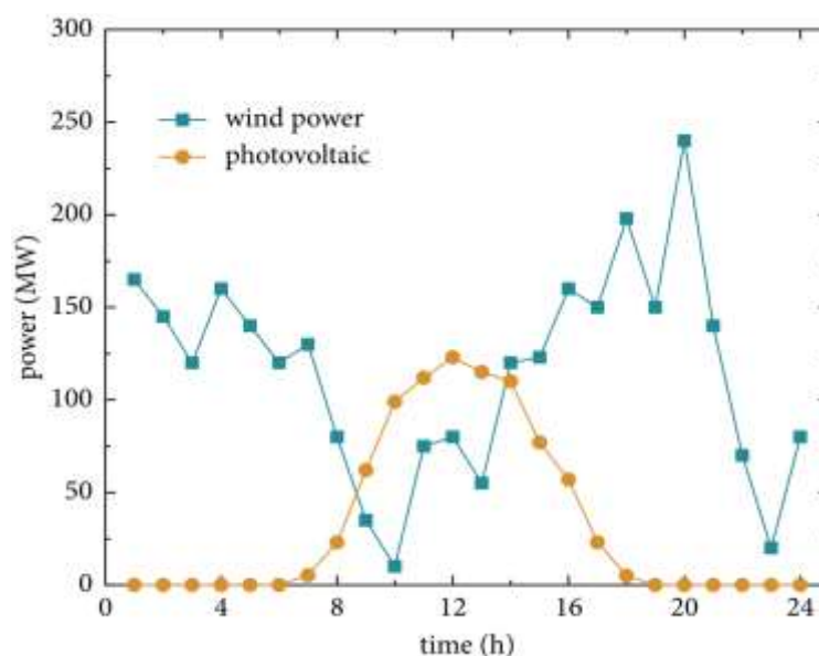
Figura 17: Esempio dell'andamento della produzione giornaliera da fonte solare (PV) ed eolica [5].
